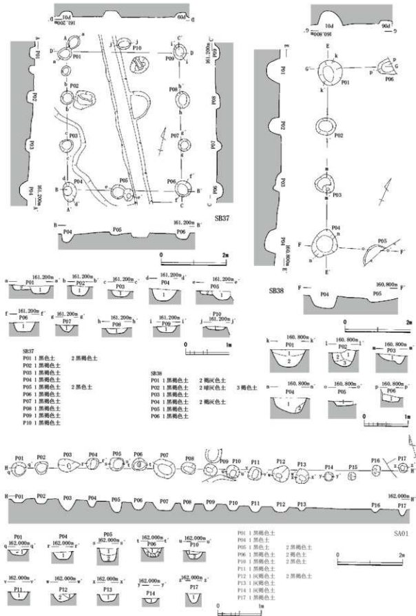
第35図 SB37・38、SA01 (縮尺1/60・1/80)
