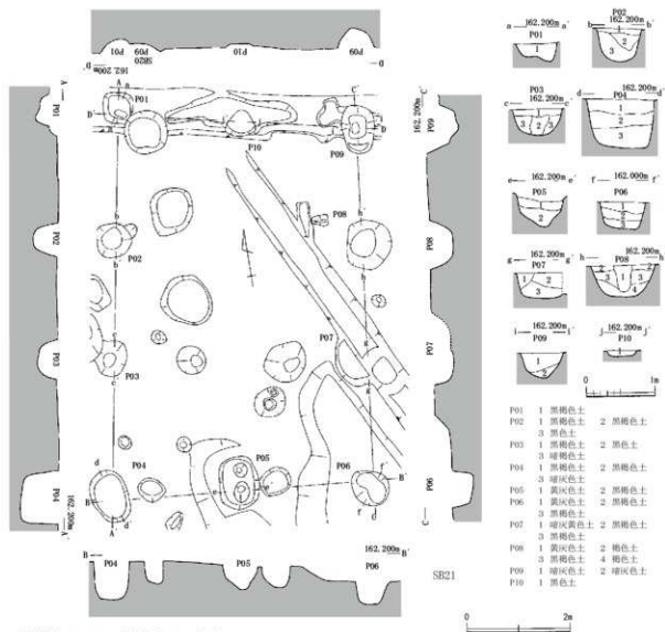
第22図 SB21 (縮尺1/60・1/80)
