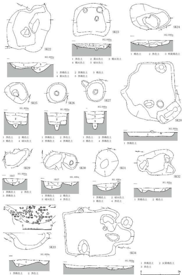
第47図 SK22~34 (縮尺1/40・1/60)
