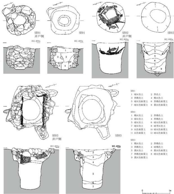
第41図 SE01~03 (縮尺1/40)
