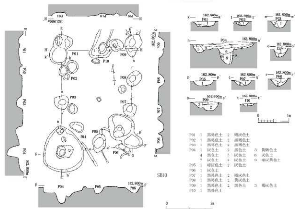
第13図 SB09・10 (縮尺1/60・1/80)
