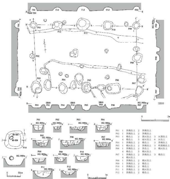
第12図 SB08 (縮尺1/40・1/60・1/80)
