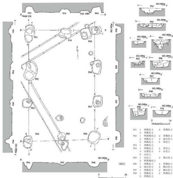
第8図 SB02 (縮尺1/60・1/80)
