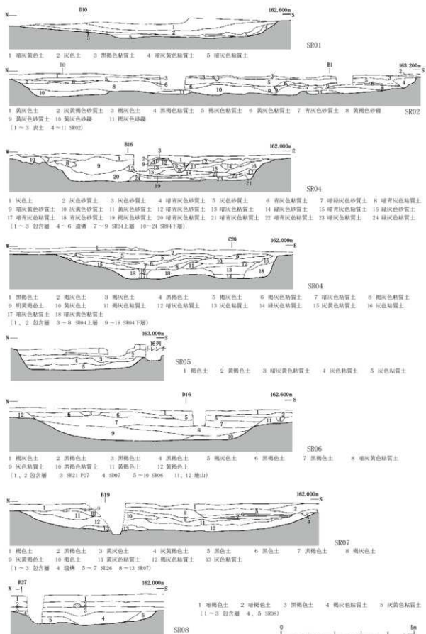
第50図 SR01・02・04~08土層断面図(縮尺1/100)
