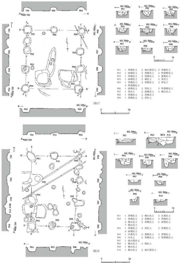
第19図 SB17・18 (縮尺1/60・1/80)
