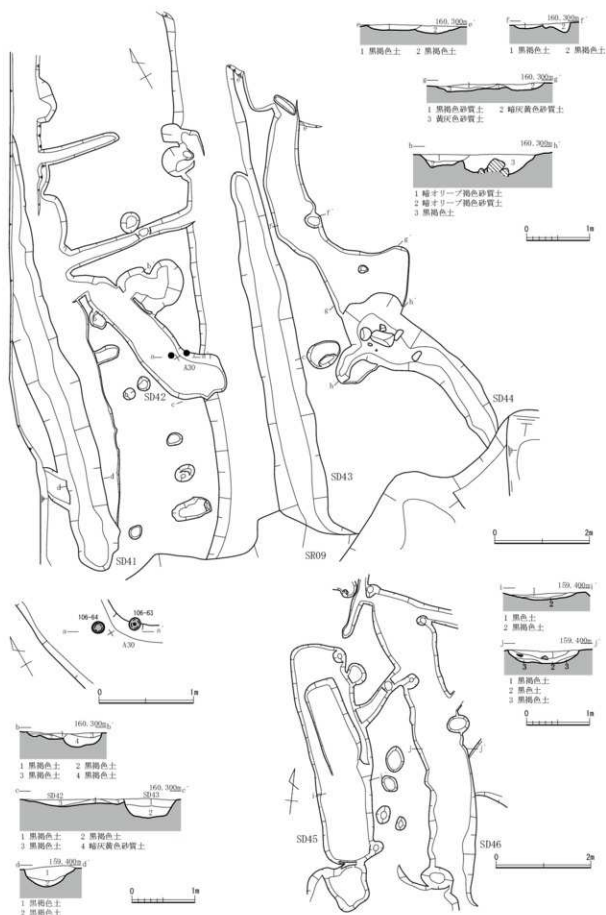
第57図 SD41~46 (縮尺1/40・1/60・1/80)
