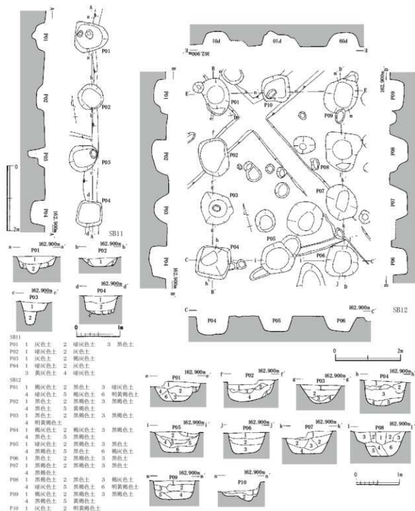
第14図 SB11・12 (縮尺1/60・1/80)
