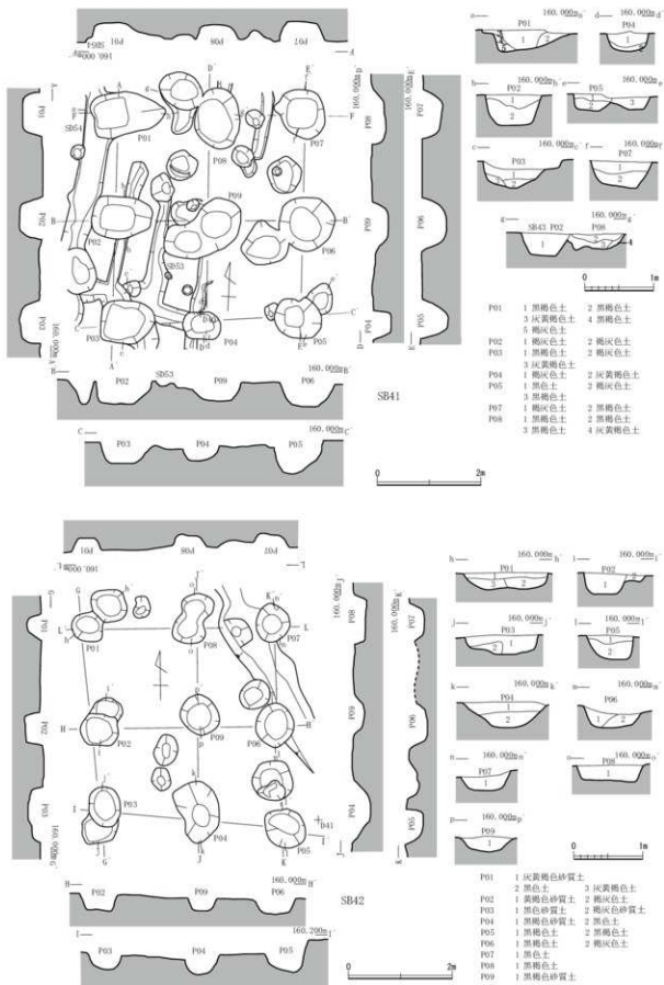
第52圖 S B 41・42 (縮尺1/60・1/80)
