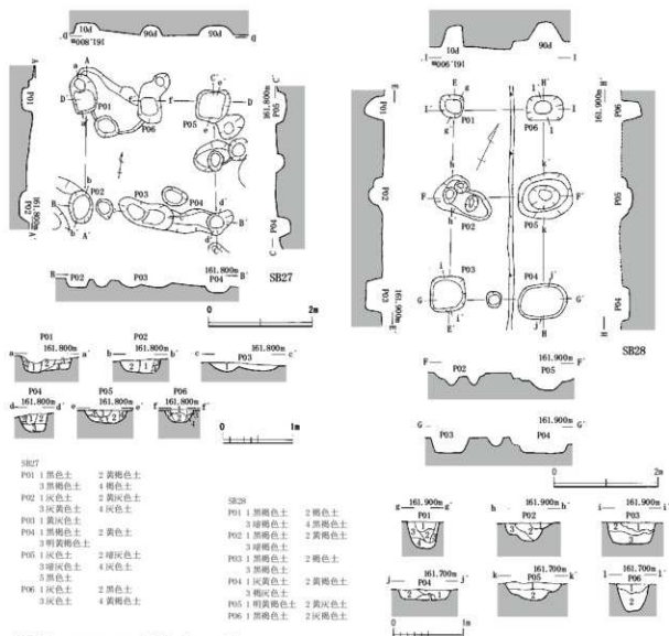
第28図 SB27・28 (縮尺1/60・1/80)
