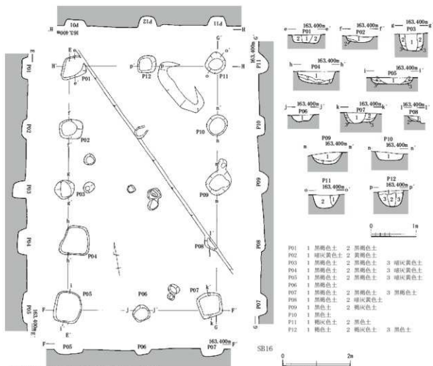
第18圖 SB15・16 (縮尺1/60・1/80)
