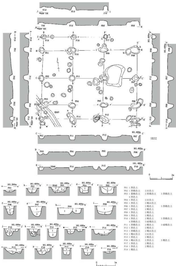
第32図 SB32 (縮尺1/60・1/100)
