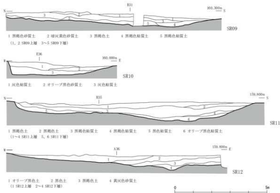
第60図 SR09～12土層断面図（縮尺1/100）
