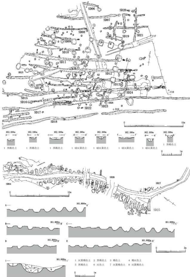
第37図 SD06~25 (縮尺1/60・1/80・1/200)
