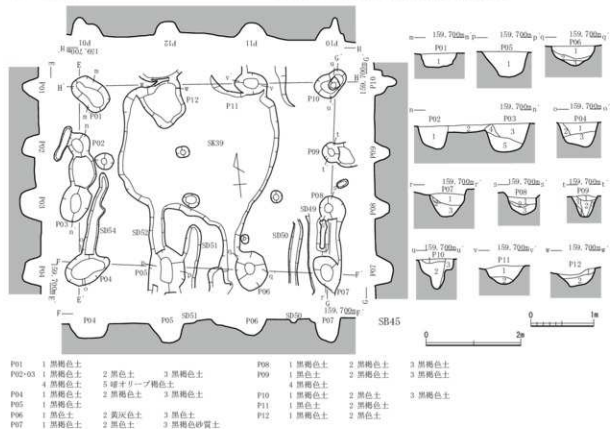
第54図 SB44・45 (縮尺1/60・1/80)
