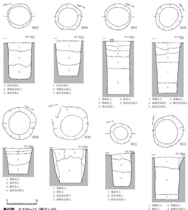
第43図 SE05～12 (縮尺1/40)
