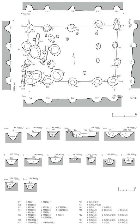
第53図 SB43 (縮尺1/60・1/80)
