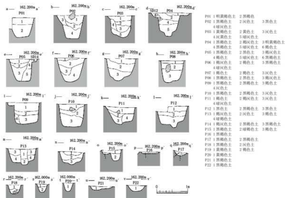
第27図 SB26 (2) (縮尺1/60)
