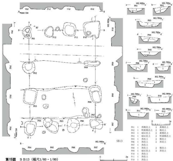
第15図 SB13 (縮尺1/60・1/80)
