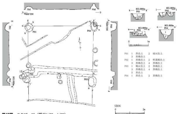
第10圖 SB05・06 (縮尺1/60・1/80)
