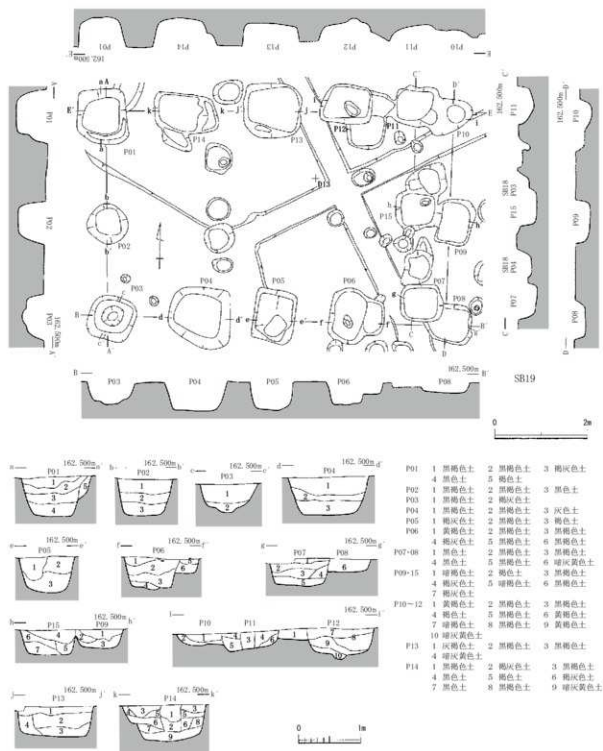
第20図 SB19 (縮尺1/60・1/80)
