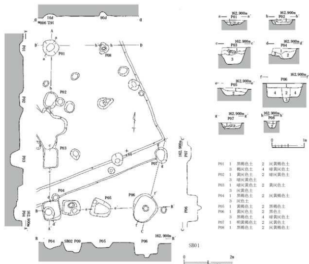
第7図 SB 01（縮尺1/60・1/80）
