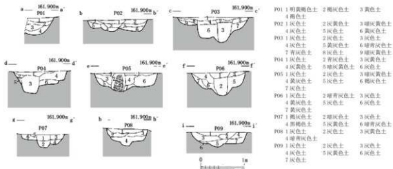
第29図 S B29 (縮尺1/60・1/80)
