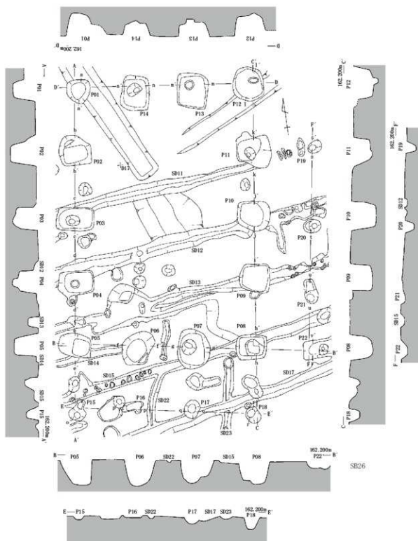
第26図 SB26 (1) (縮尺1/80)
