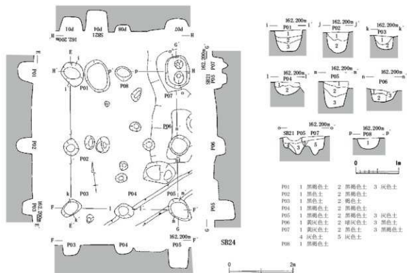
第24图 SB23·24 (縮尺1/60·1/80)
