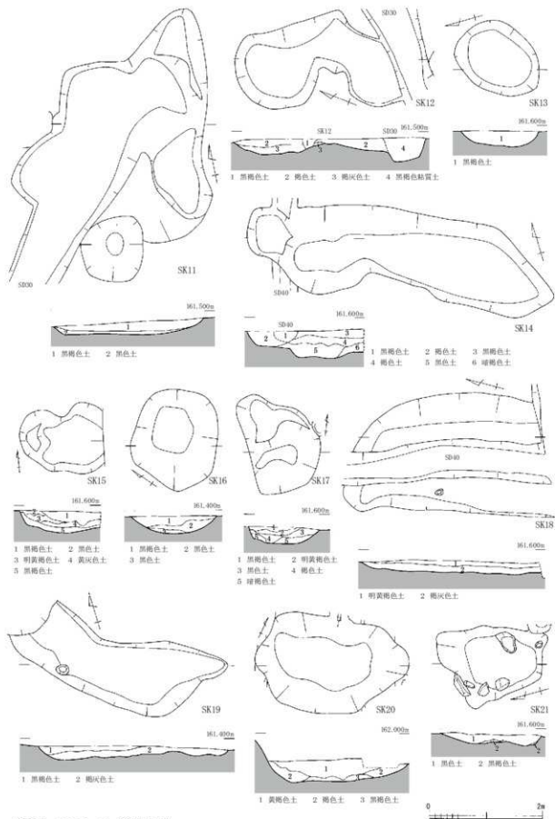
第46図 SK11~21 (縮尺1/60)
