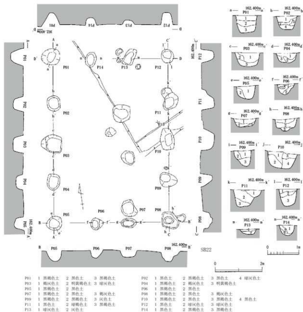
第23図 SB22 (縮尺1/60・1/80)
