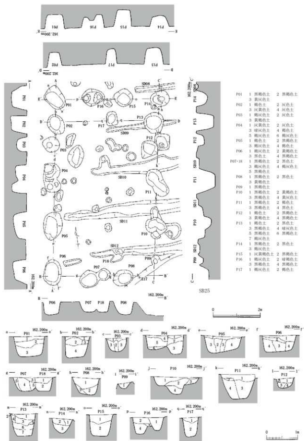
第25図 SB25 (縮尺1/60・1/80)
