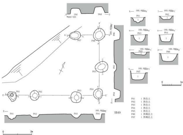
第56圖 SB48・49 (縮尺1/60・1/80)
