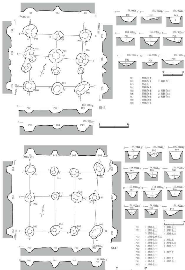
第55図 SB46・47 (縮尺1/60・1/80)
