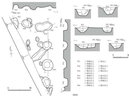
第51図 SB39・40 (縮尺1/60・1/80)
