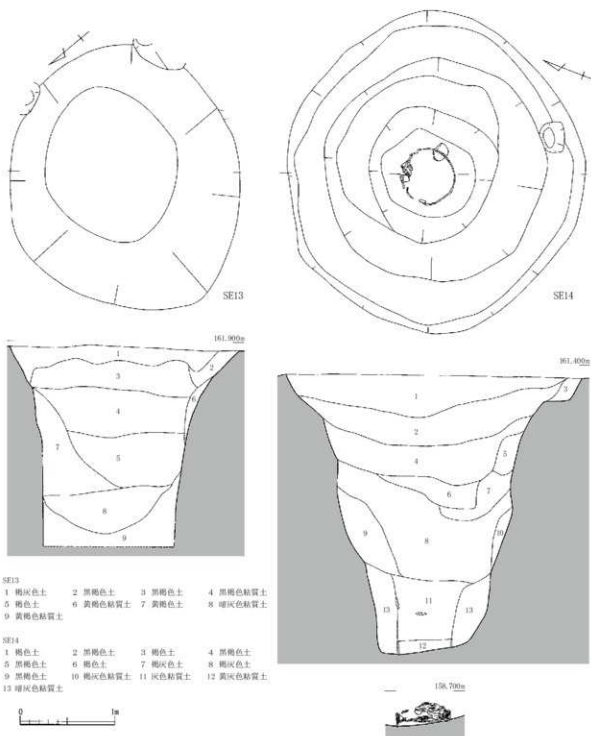
第44図 SE13・14 (縮尺1/40)
