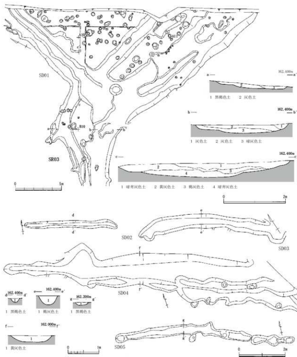
第36図 SD01～05 (縮尺1/60・1/80・1/200)
