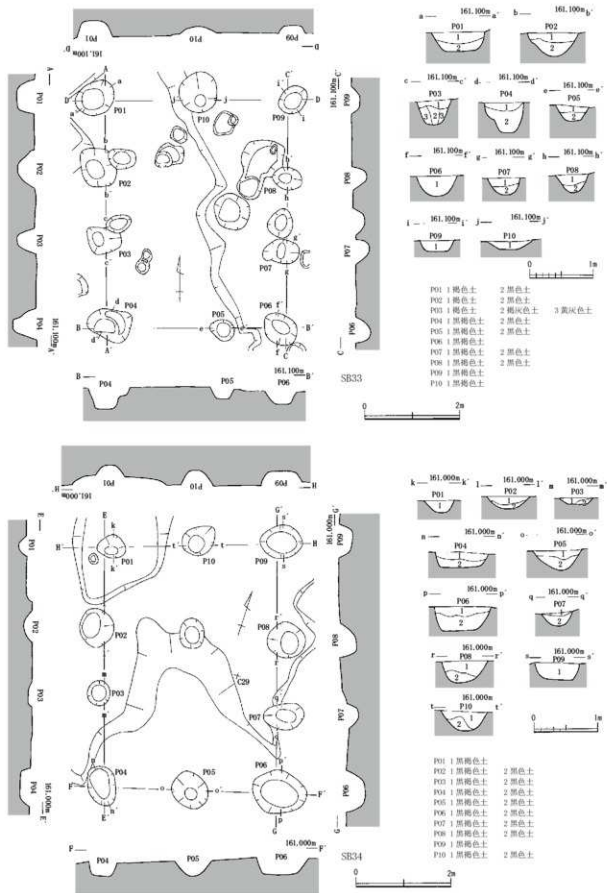
第33図 S B33・34 (縮尺1/60・1/80)
