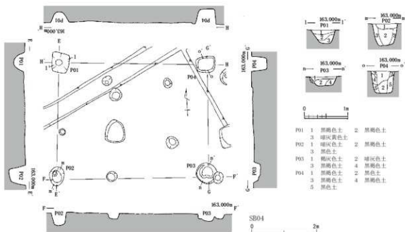
第9図 S B03・04 (縮尺1/60・1/80)
