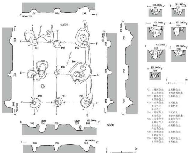
第30図 SB30 (縮尺1/60・1/80)
