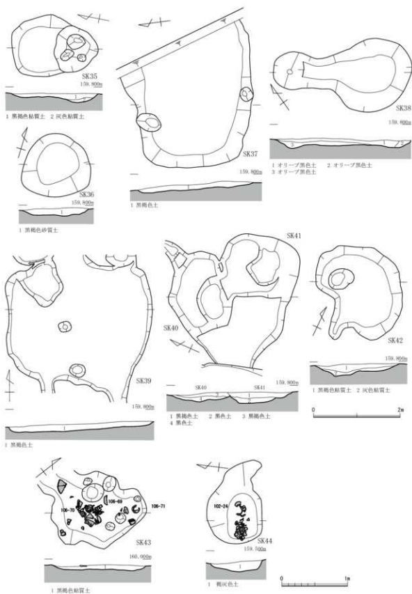
第59図 SK35~44 (縮尺1/40・1/60)
