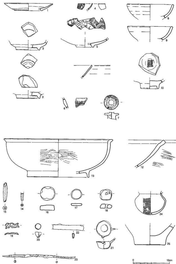
第384图 A63区出土遗物夹测图②
