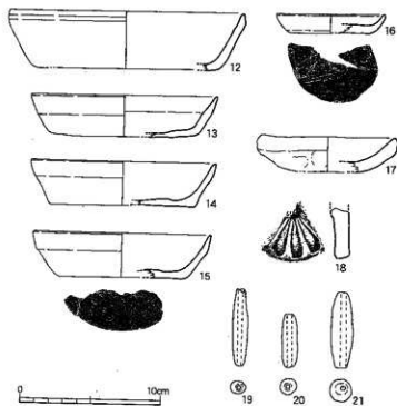
第399图 E64区出土文物实测图
