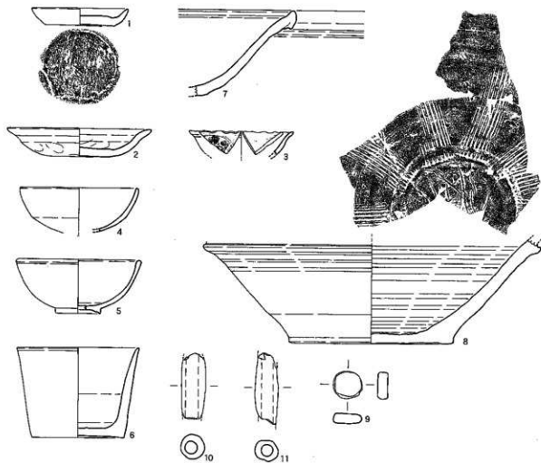
第398图 D64区出土文物实测图
