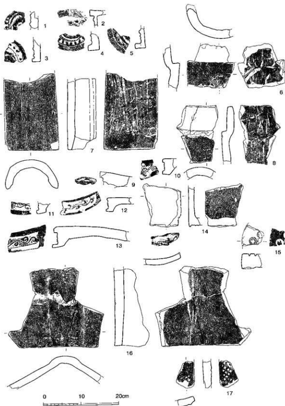
第204図 包倉層出土瓦実測図 ⑨ (1/5)
