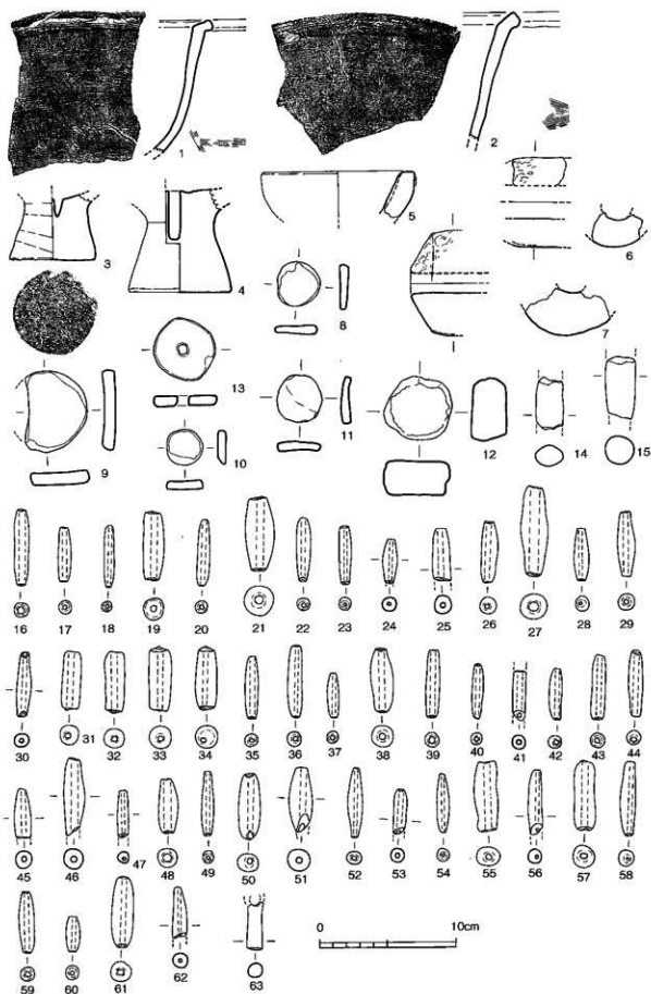
第199図 包倉層出土遺物実測図⑬ (1/3)
