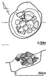
第160図 SK248実測図 (1/20)
