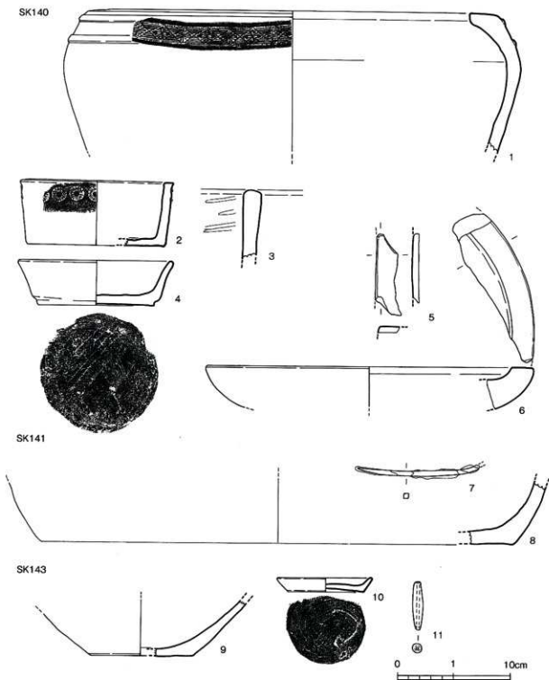
第121図 SK140・141・143出土遺物実測図 (1/3)
