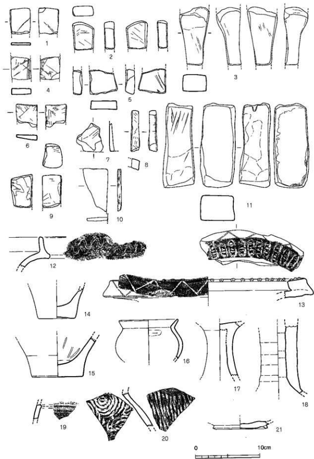
第201図 包倉層出土遺物実測図⑤ (1/3)
