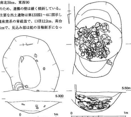
第132図 SK155実測図 (1/20)
