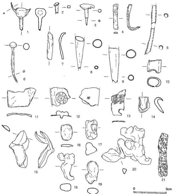
第203図 包倉層出土青銅製品実測図⑪ (1/1)
