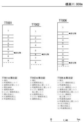
第 24 図 整理番号 19-2-309 試掘調査実施箇所及び土層断面模式図
