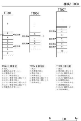
第 25 図 整理番号 19-2-310 試掘調査実施箇所及び土層断面模式図
