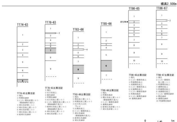
第 11 図 整理番号 15-3-301 試掘調査実施箇所及び土層断面模式図
