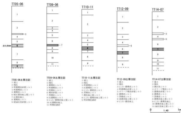
第16図 整理番号19-3-310 試掘調査実施箇所及び土層断面模式図
