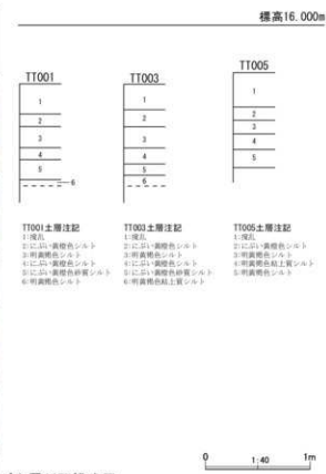
第 29 図 整理番号 18-2-308 試掘調査実施箇所及び土層断面模式図
