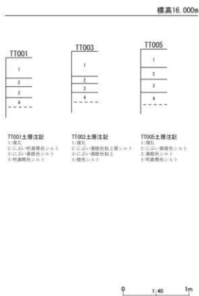
第 31 図 整理番号 18-2-310 試掘調査実施箇所及び土層断面模式図
