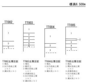
第26図 整理番号 18-2-305 試掘調査実施箇所及び土層断面模式図
