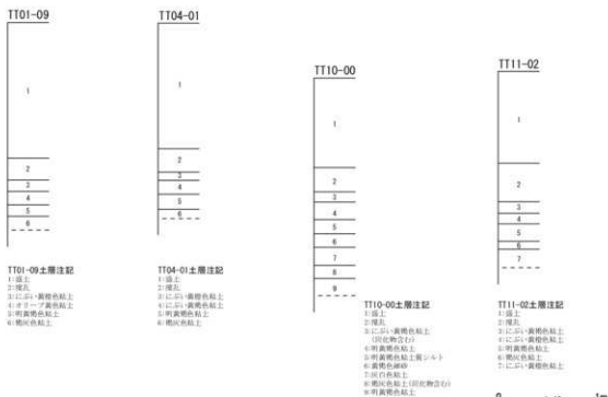
第16図 整理番号 18-3-301 試掘調査実施箇所及び土層断面模式図
