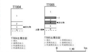
第 28 図 整理番号 18-2-307 試掘調査実施箇所及び土層断面模式図
