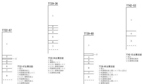
第 9 図 整理番号 14-3-321 試掘調査実施箇所及び土層断面模式図
