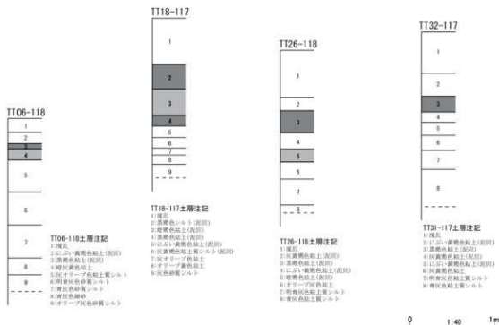
第7図 整理番号 07-3-325 試掘調査実施箇所及び土層断面模式図
