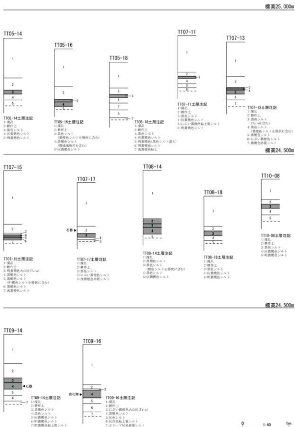
第20図 整理番号16-3-312 試験調査土層断面模式図
