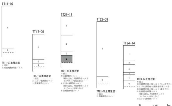
第16図 整理番号 16-3-304 試験調査実施箇所及び土層断面模式図
