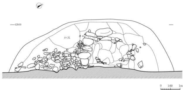
图7 断面图
