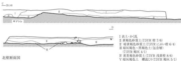
南壁断面図
