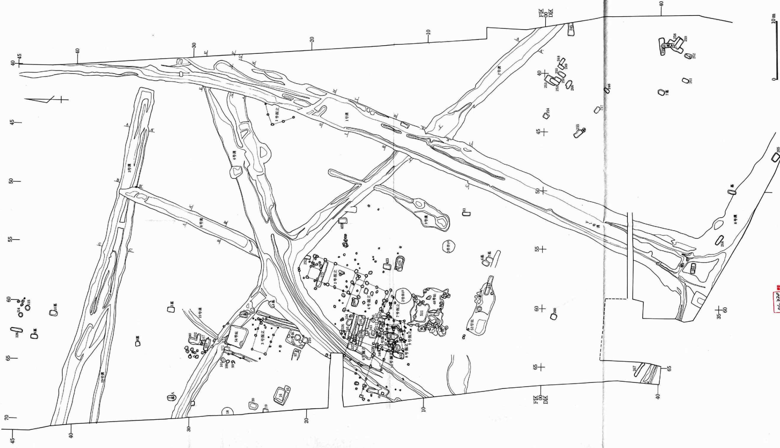
附圖 2 D·F·F 区 全体圖 (1:200)
