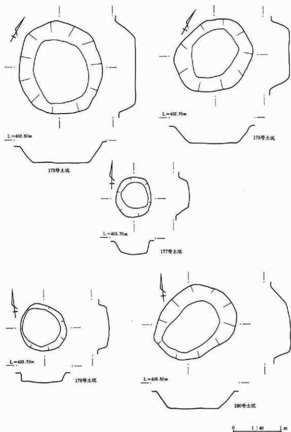
第521图 土坑实测图
