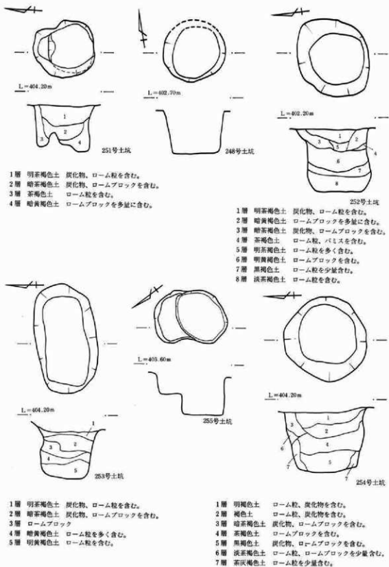
第534図 土坑実測図
