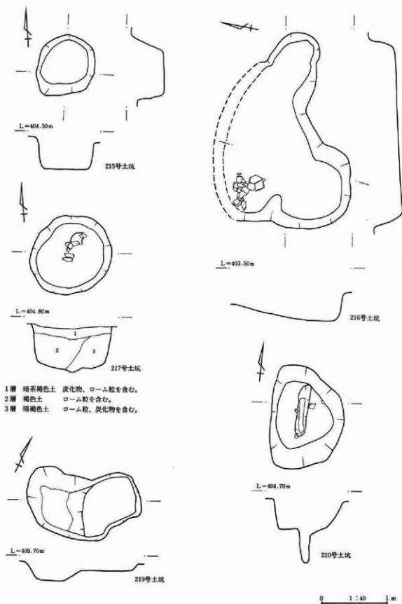
第529図 土坑実測図
