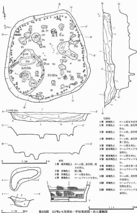
第335図 121号a・b住居址・炉址実測図・出土遺物図
