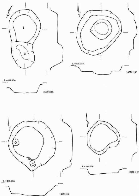
第519图 土坑实测图
