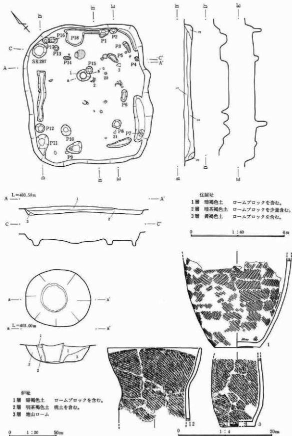
第440図 144号住居址・炉址実測図・出土遺物図
