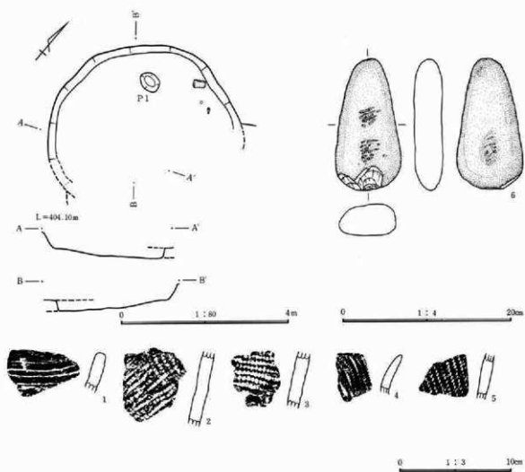
第8图 6号住居址实测图·出土物图
