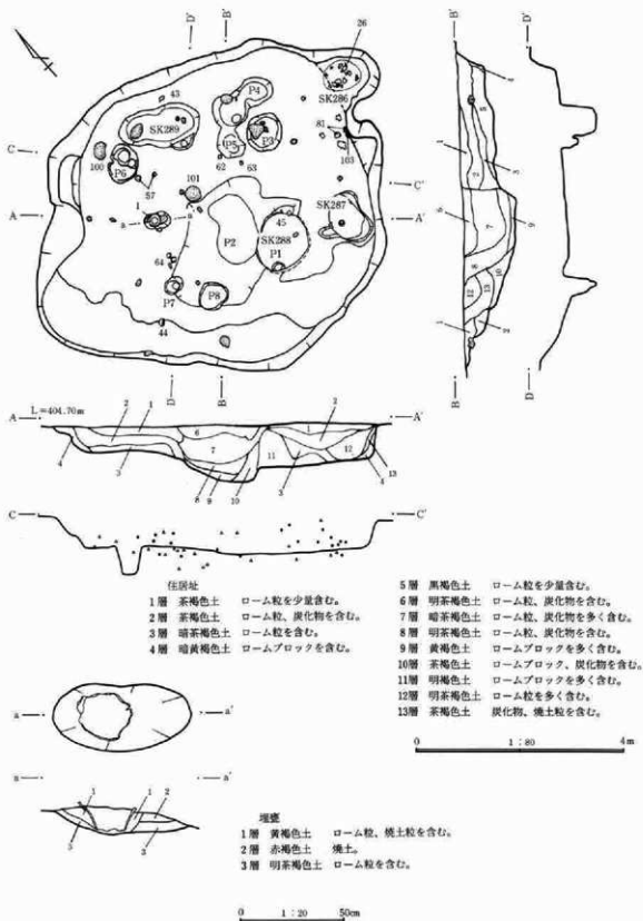
第182図 90号住居址・炉址実測図
