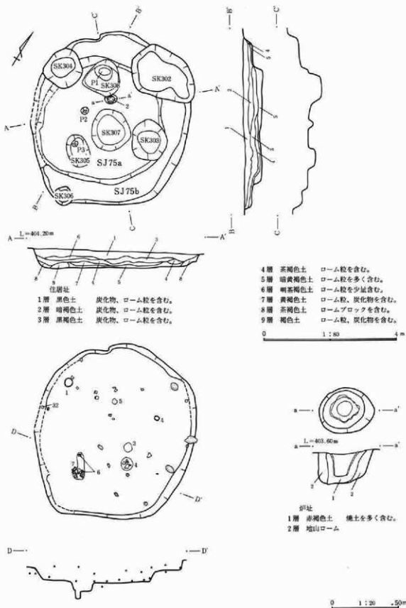
第107図 75号a・b住居址・炉址・遺物出土状態実測図
