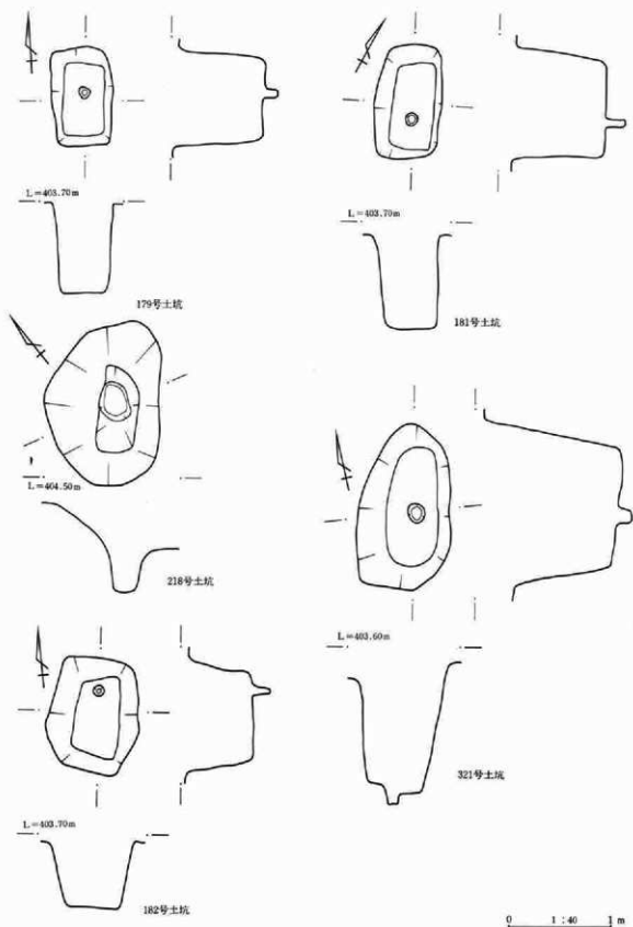
第487图 土坑实测图
