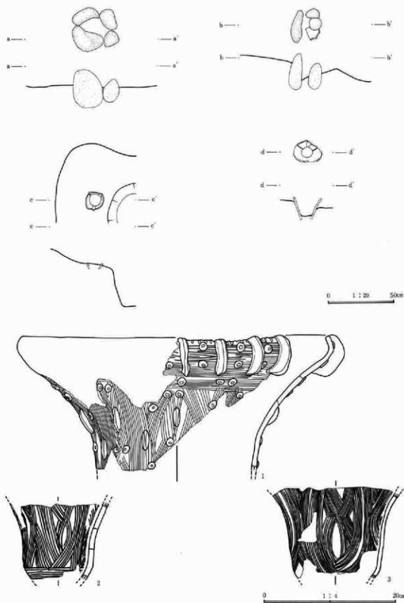
第27图 15号住居炉址实测图·出土遗物图
