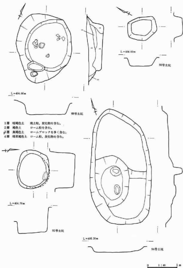
第503図 土坑実測図
