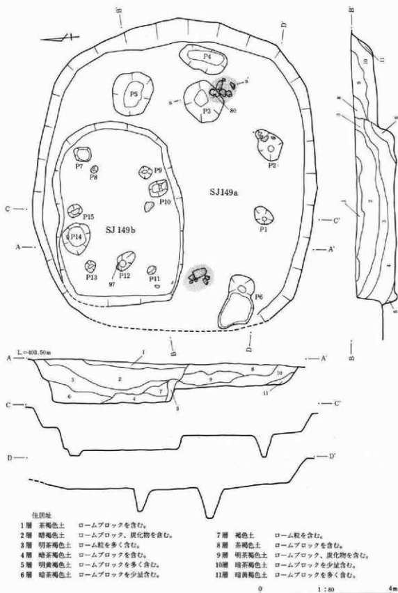
第451図 149号a・b住居址実測図
