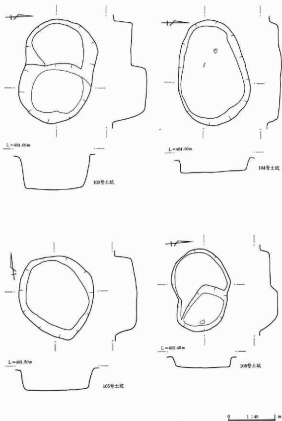
第507图 土坑实测图
