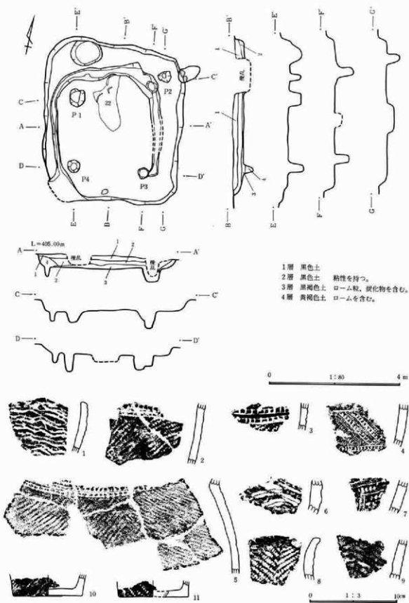
第2図 2号住居址実測図・出土遺物図
