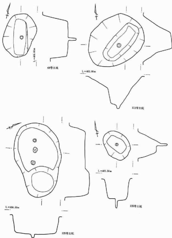
第485图 土坑实测图
