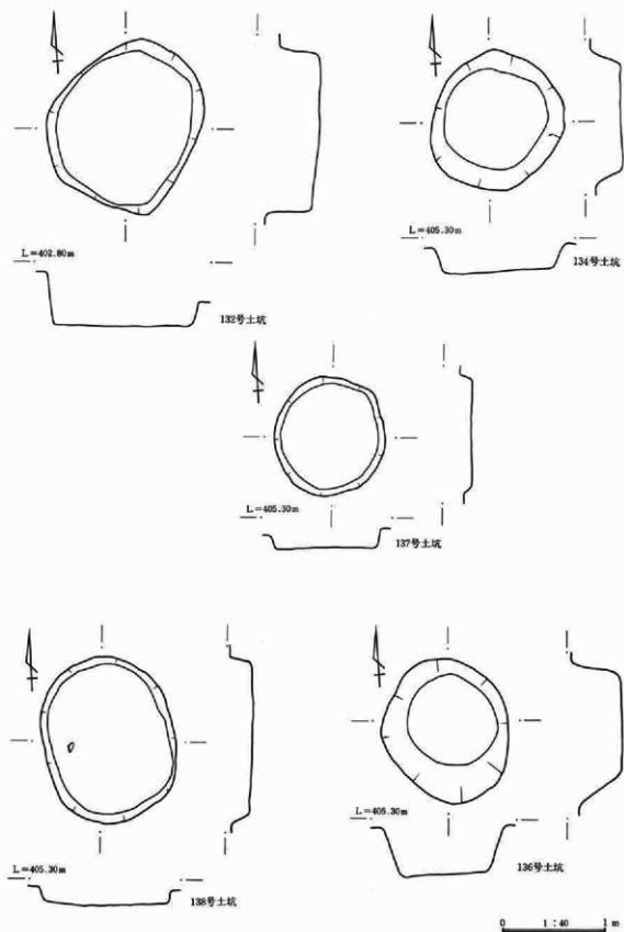
第513图 土坑实测图
