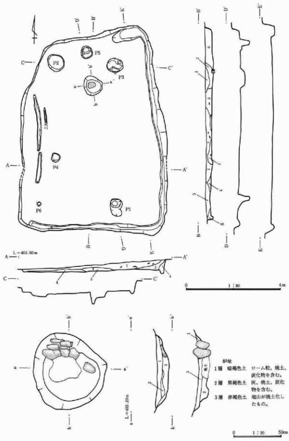
第90図 72号住居址・炉址実測図
