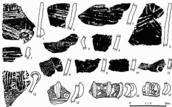
第9図 7号住居址実測図・出土遺物図
