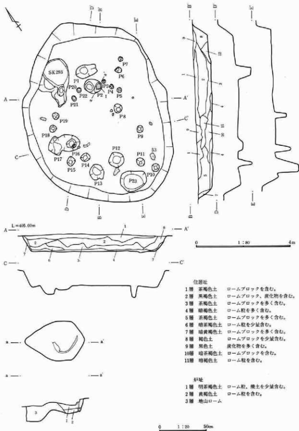
第423図 140号住居址・炉址実測図
