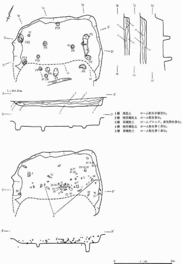
第72図 67号住居址・遺物出土状態実測図
