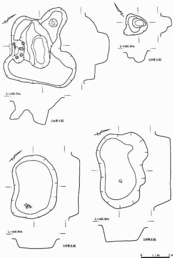
第509图 土坑实测图
