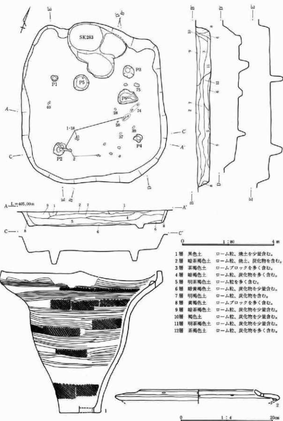
第326図 117号住居址実測図・出土遺物図
