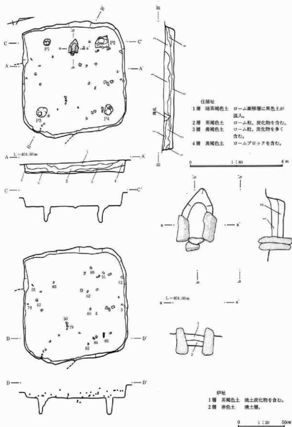
第40図 63号住居址・炉址・遺物出土状態実測図
