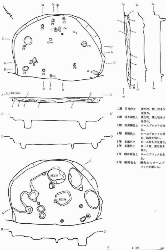
第52図 65号住居址実測図
