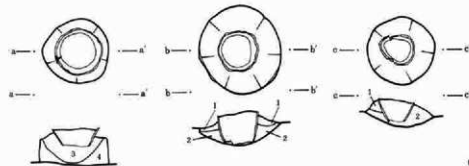
第369図 129号住居址・炉址実測図
