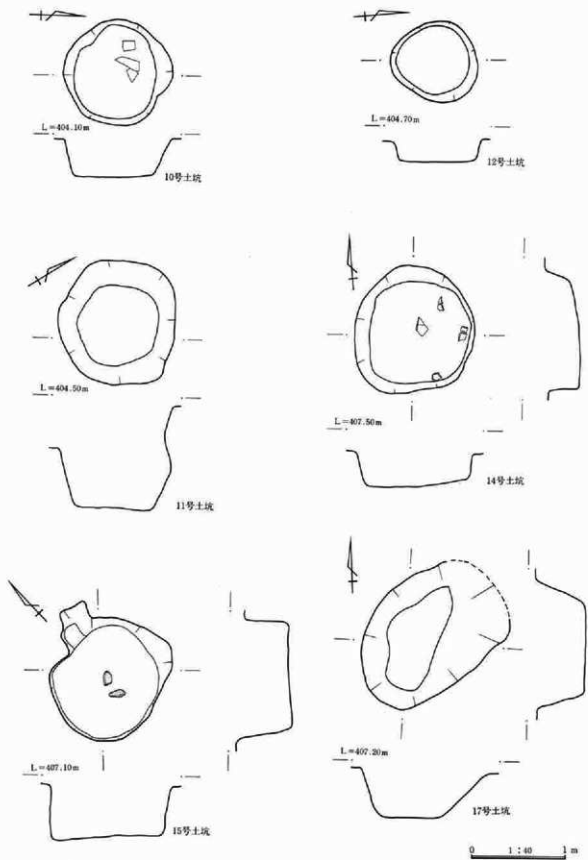
第491图 土坑实测图
