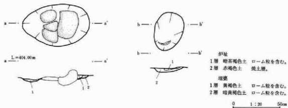
第410図 136号住居址・炉址実測図
