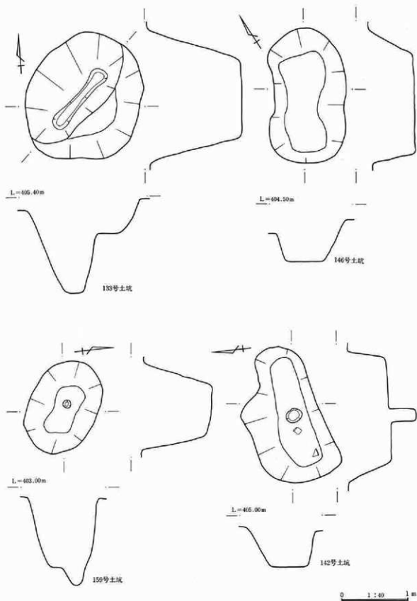
第486图 土坑实测图
