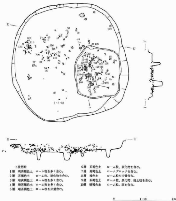
第57図 66号住居址遺物出土状態実測図
