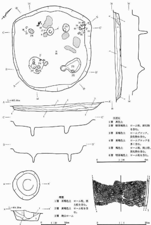
第178図 89号住居址・炉址実測図・出土遺物図
