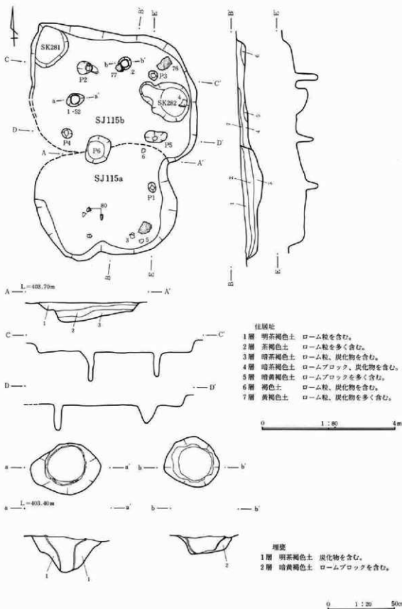
第307図 115号a・b住居址・炉址実測図
