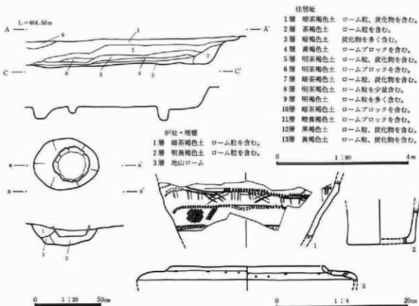
第418図 139号住居址・炉址実測図・出土遺物図
