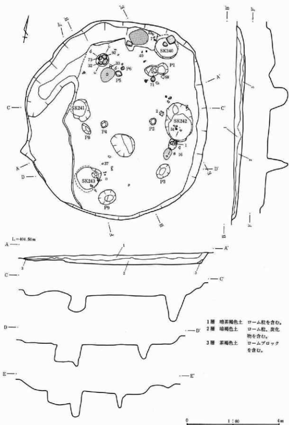
第78図 68号住居址実測図
