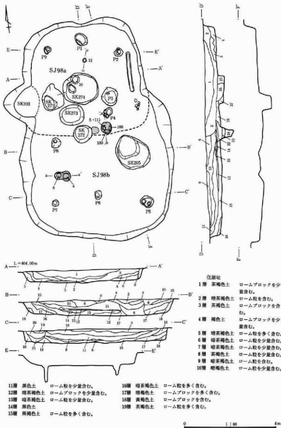
第217図 98a・b住居址実測図
