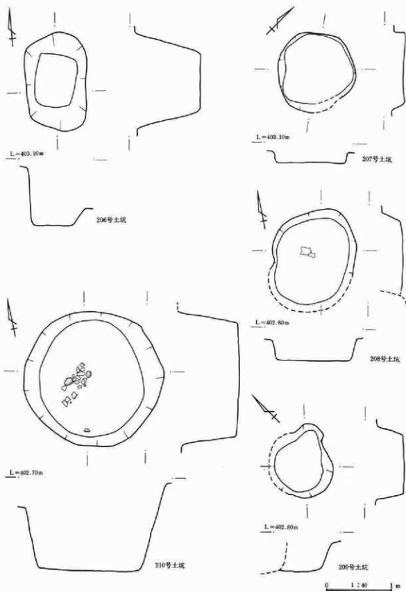
第527图 土坑实测图
