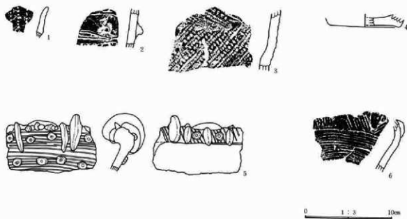
第24図 14号住居址実測図・出土遺物図
