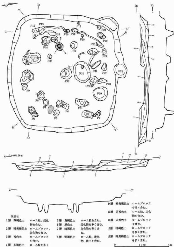
第353図 128号住居址実測図
