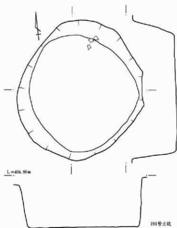
第523图 土坑实测图
