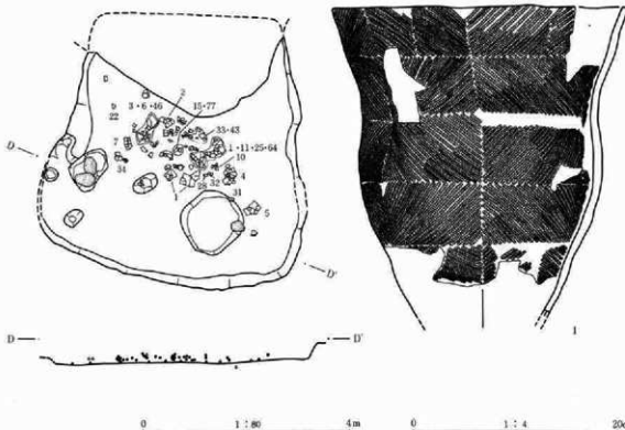
第46図 64号住居址・遺物出土状態実測図・出土遺物図
