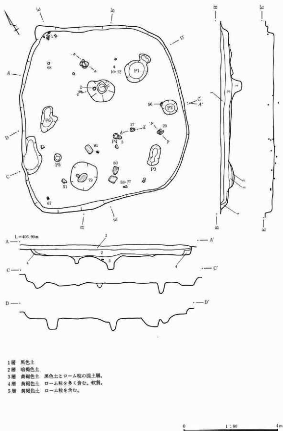
第26図 15号住居址実測図
