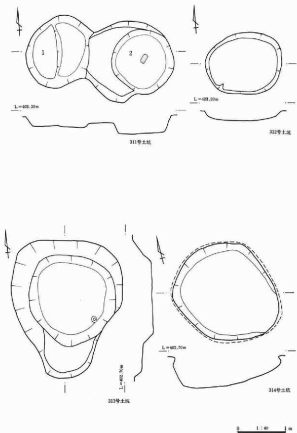
第549图 土坑实测图
