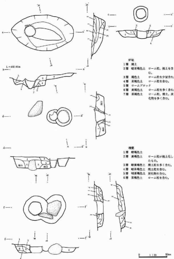
第97図 73号住居炉址実測図
