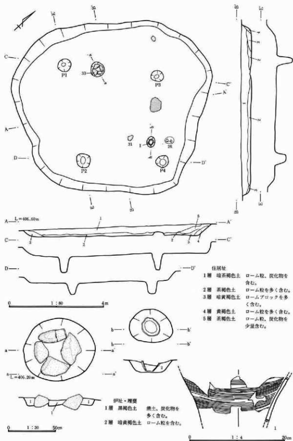
第347図 126号住居址・炉址実測図・出土遺物図
