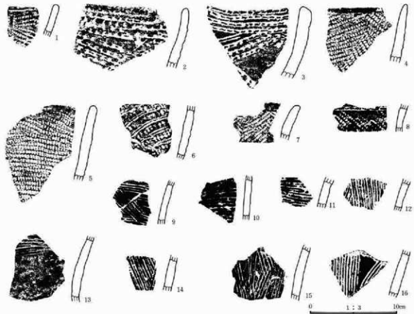
第35図 17号住居址実測図・出土遺物図
