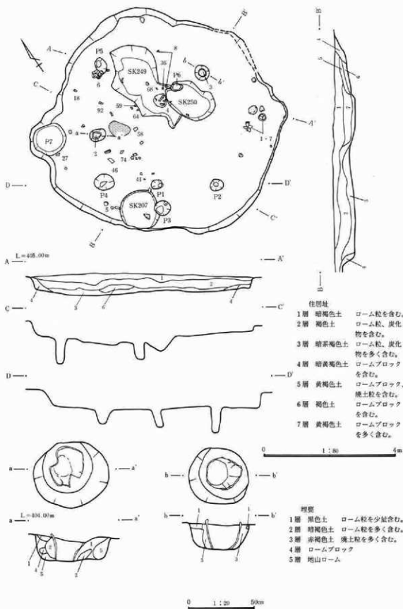
第148図 81号住居址・塚墓実測図
