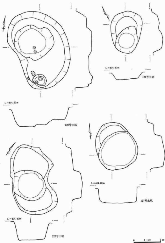
第511图 土坑实测图
