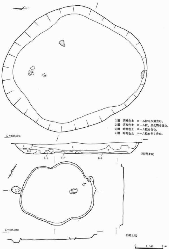
第552図 土坑実測図
