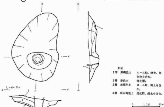
第37図 53号住居址・炉址実測図
