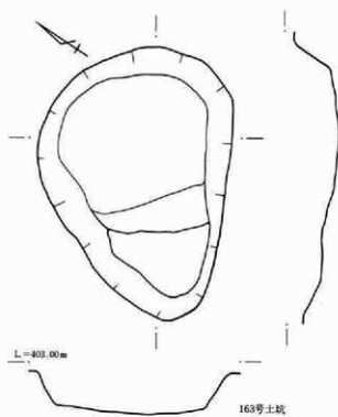
第518图 土坑实测图
