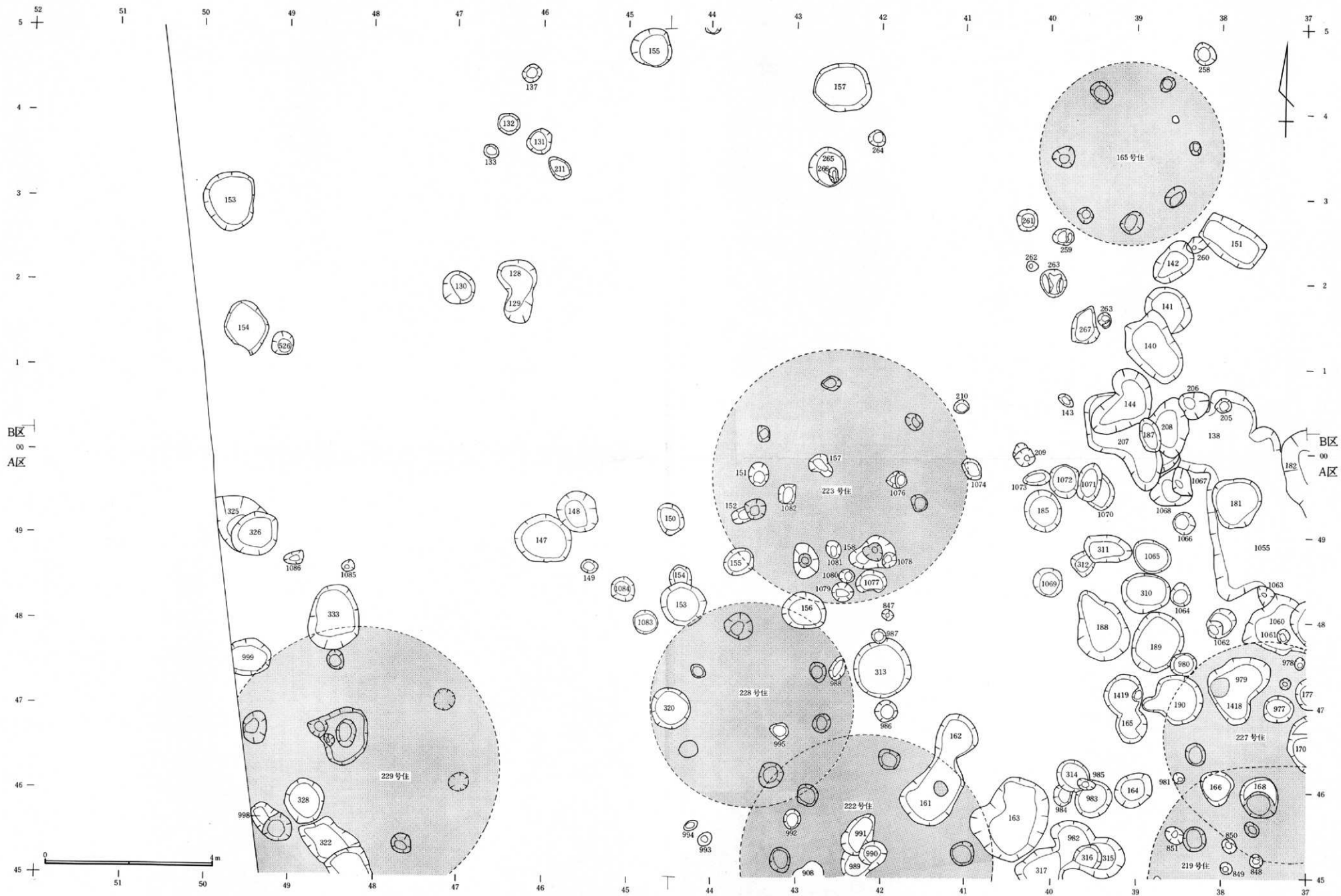
付図7. 縄文時代土坑全体図(部分) 4 1:60
