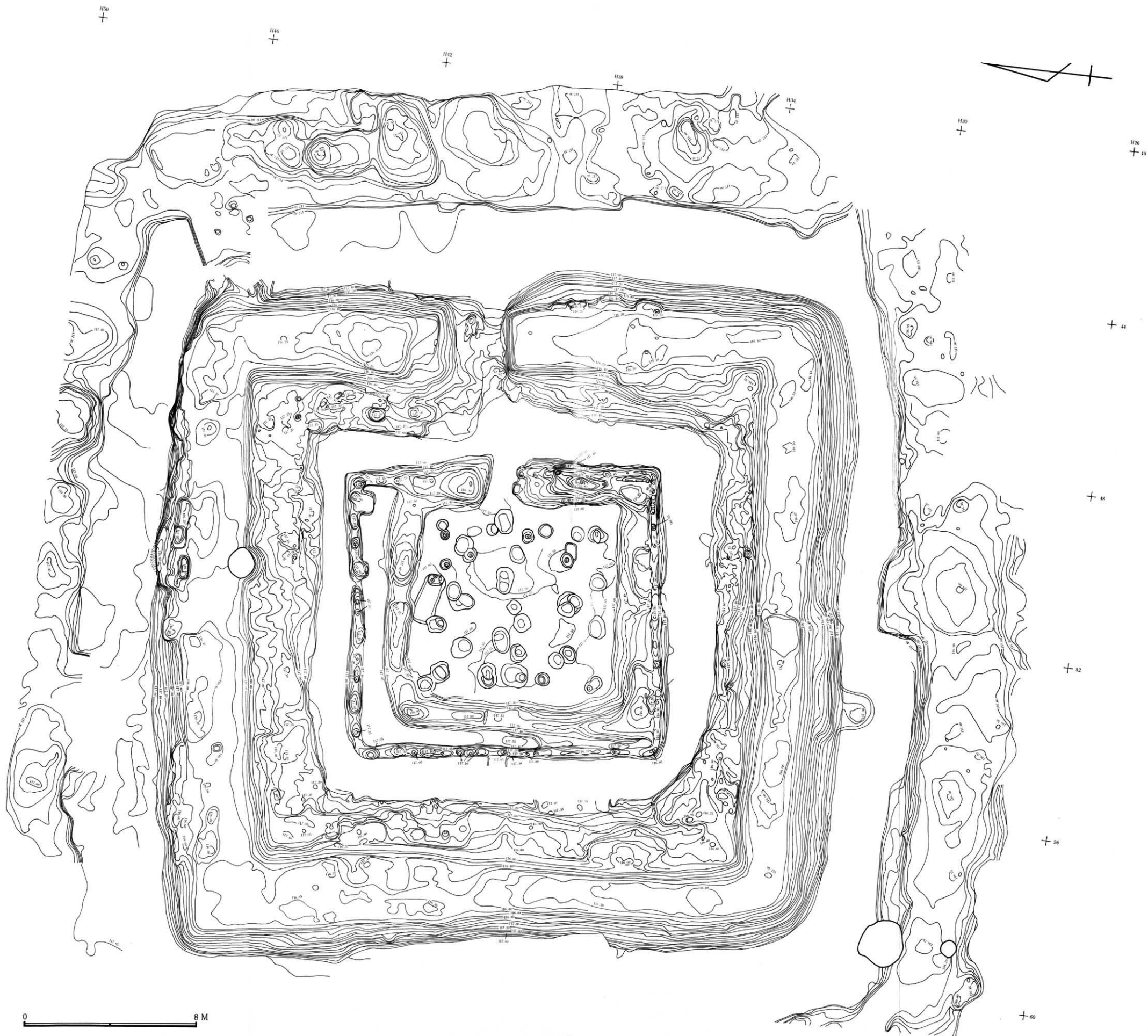
付图4 H1号掘立柱建物跡等高线图1:80
