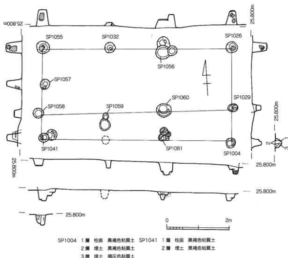
第9図 1次調査区SB1049実測図(S=1/60)
