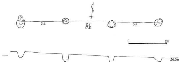
第63図 3次調査区SA019(1/60)
