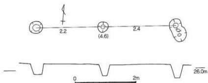
第65図 3次調査区SA021(1/60)
