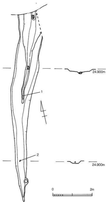
第21图 1次調査区SD2012実測図(S=1/60)
