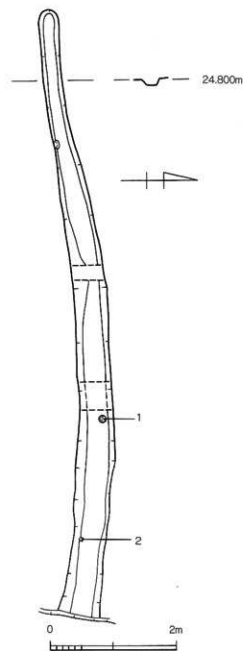
第23图 1次調査区SD2001実測図(S=1/60)
