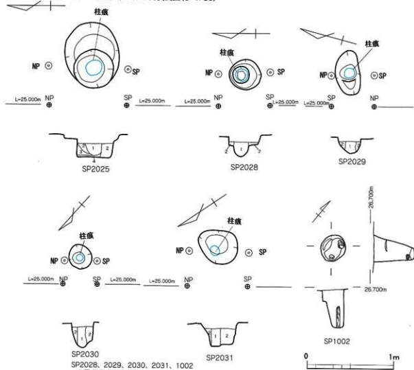
第31図 1次調査区SK2035実測図(S=1/30)
