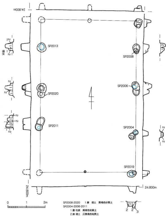
第14図 1次調査区SB2037実測図(S=1/60)
