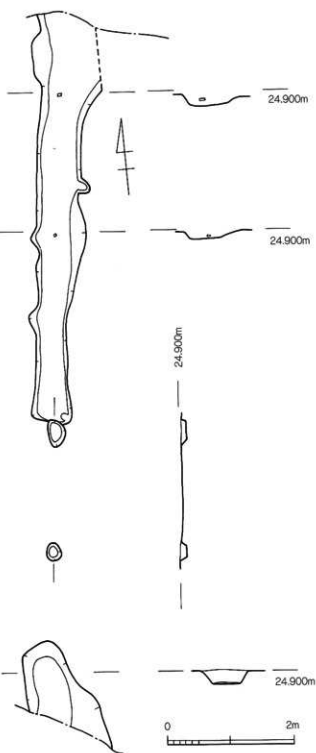
第25図 1次調査区SD2022実測図(S=1/60)
