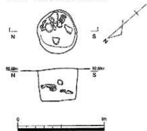
SK01 遺構平面図・立面図
