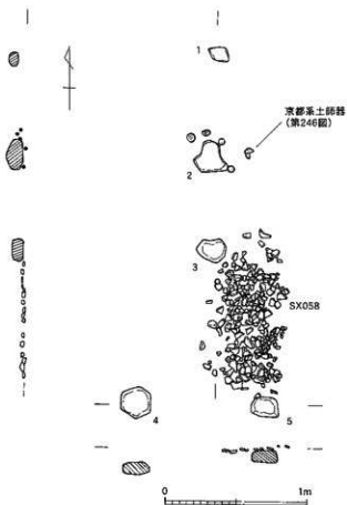
第245図 礎石建物2実測図(1/60)
