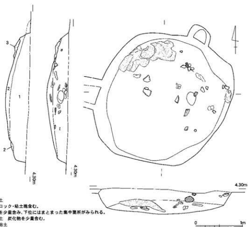
第268図 SK174実測図(1/40)
