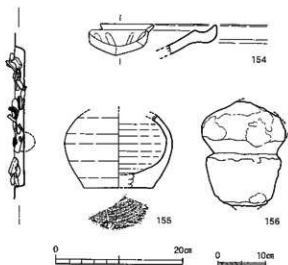
第258図 SK017出土遺物(1/3, 1/8)
