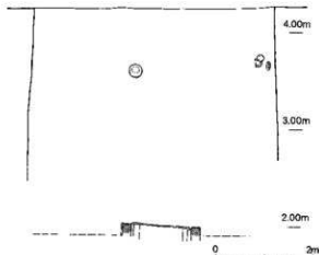
第280図 SE001実測図(1/50)
