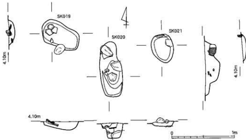
第259図 SK019～SK021実測図(1/30)
