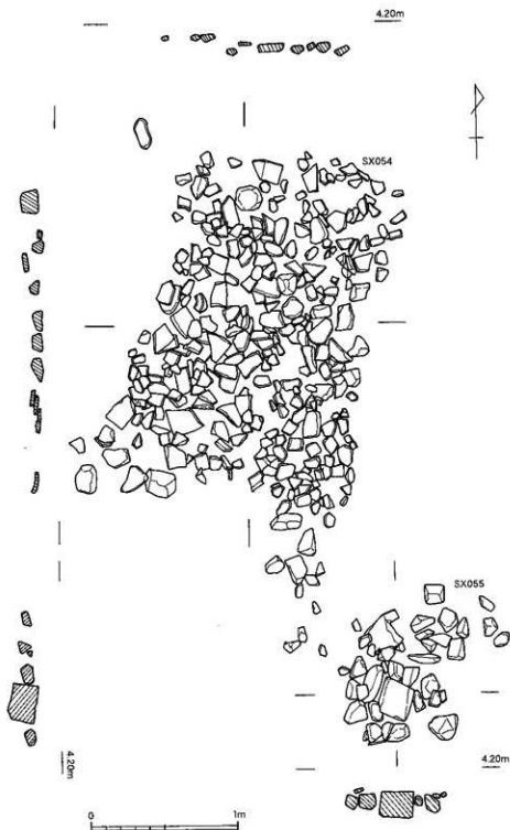
第275図 SX054・SX055実測図(1/30)
