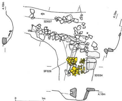
第241図 SD034・SD037・SF026実測図(1/40)
