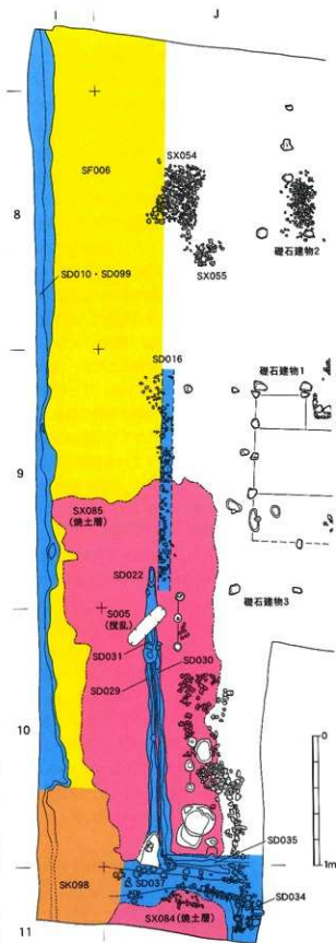
第232図 SF006と周辺の遺構配置図(1/160)
