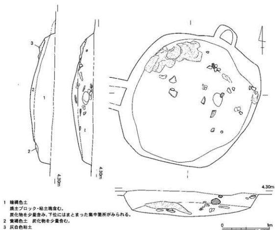
第268図 SK174実測図(1/40)
