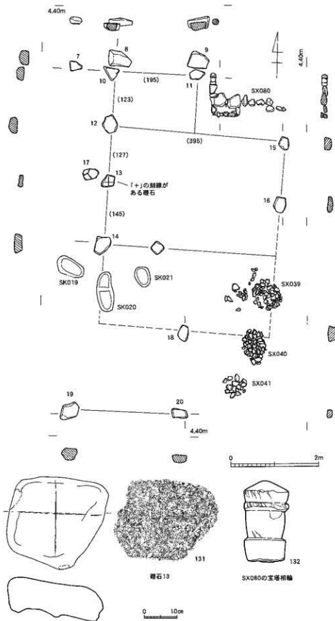
第244図 礎石建物1-3と周辺の遺構実測図(1/60, 1/8)
