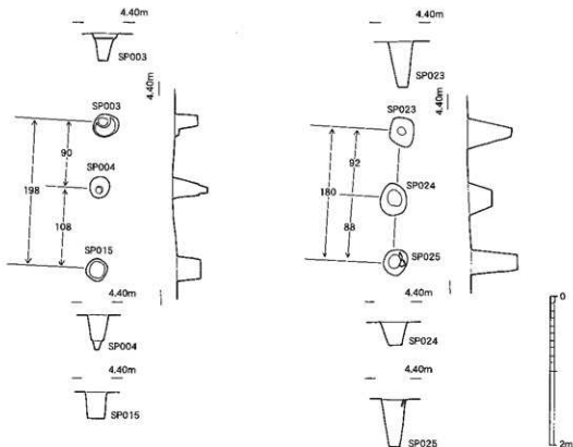
第248図 柱穴列表測図(1/60)
