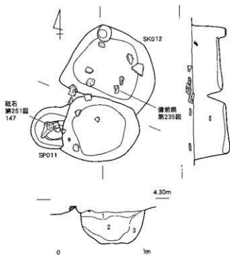
第252図 SK012実測図(1/30)
