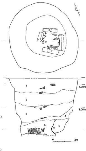
第282図 SE002実測図(1/50)
