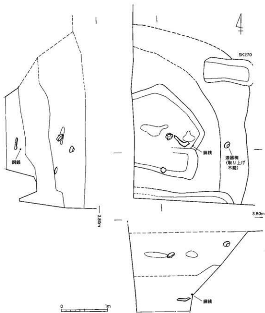
第270図 SK198実測図(1/40)
