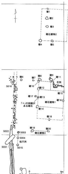
第243図 礎石建物と周辺の遺構配置図(1/150)
