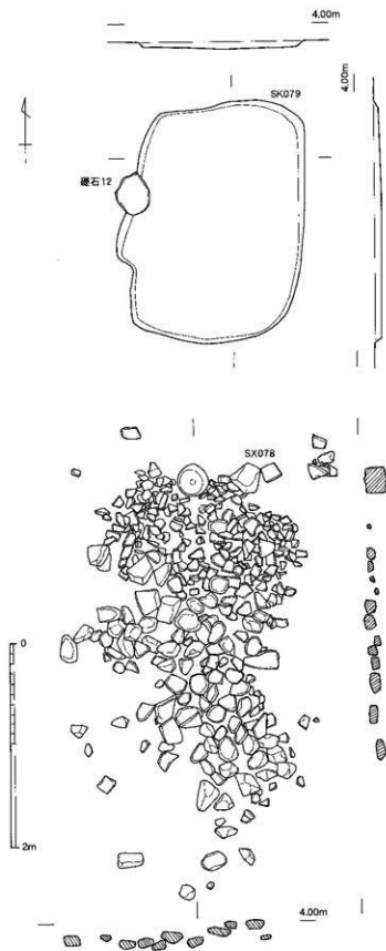
第265図 SK078・SK079実測図(1/40)
