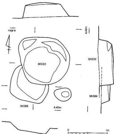
第261図 SK032・SK086実測図(1/30)
