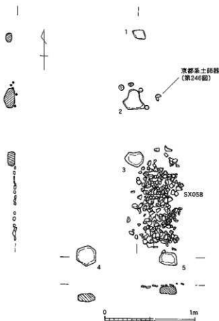
第245図 礎石建物2実測図(1/60)
