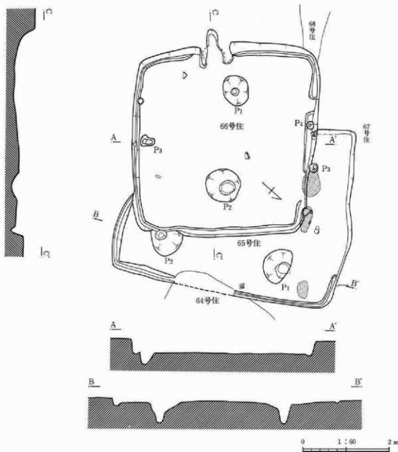
第60図 65号・66号住居跡
