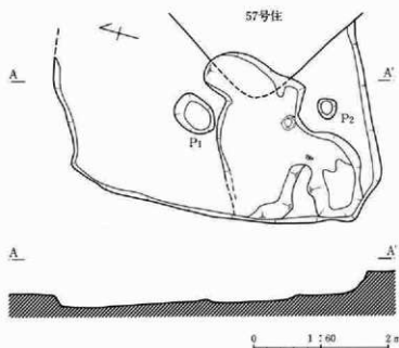
第54図 59号住居跡
