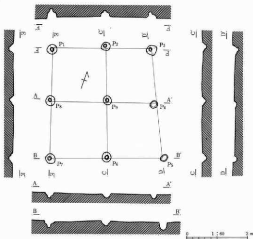
第214図 24号掘立柱建物跡
