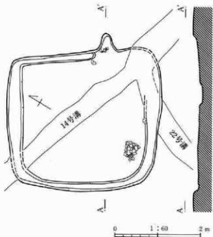
第154図 182号住居跡
