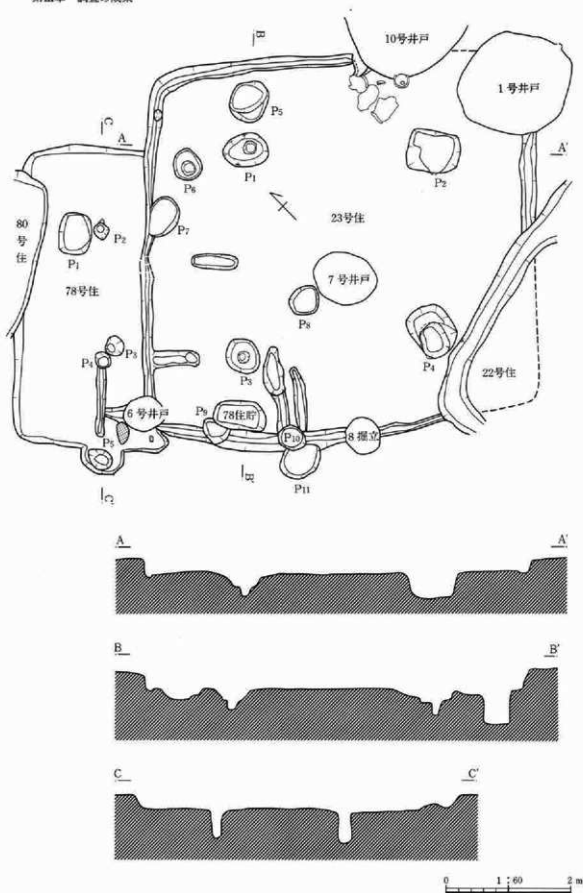
第28図 23号・78号住居跡
