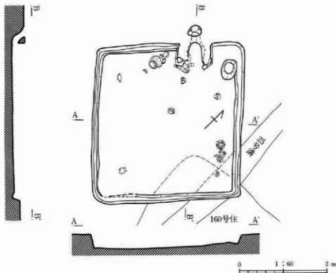
第131図 150号住居跡
