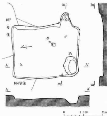
第138図 163号住居跡
