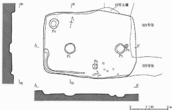
第182図 223号住居跡
