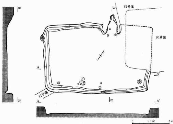
第73図 81号住居跡
