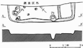
第130図 149号住居跡
