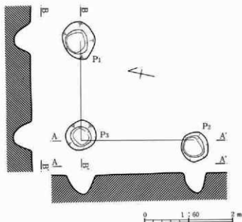
第196図 5号掘立柱建物跡
