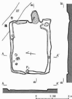
第105図 119号住居跡
