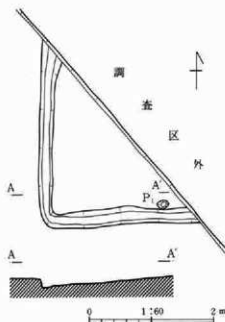
第118図 137号住居跡
