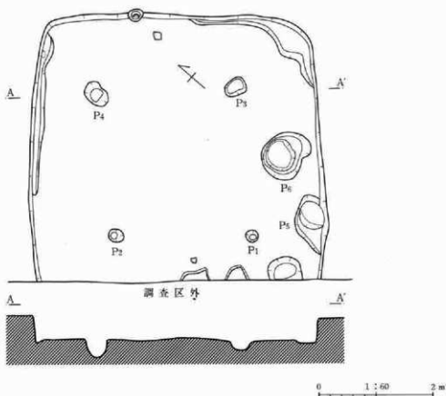
第46図 48号住居跡
