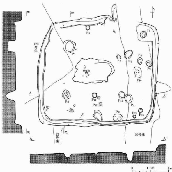
第147図 175号住居跡
