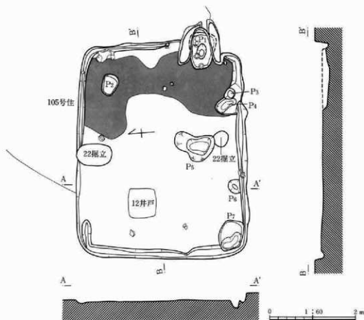
第92図 104号住居跡
