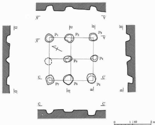
第219図 29号掘立柱建物跡
