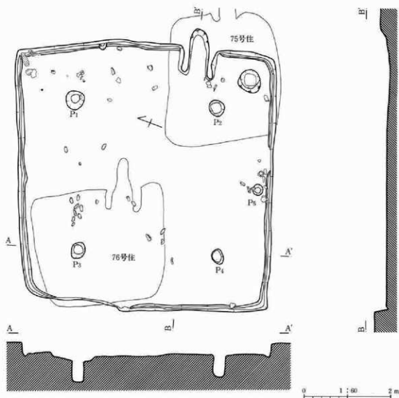
第70図 77号住居跡
