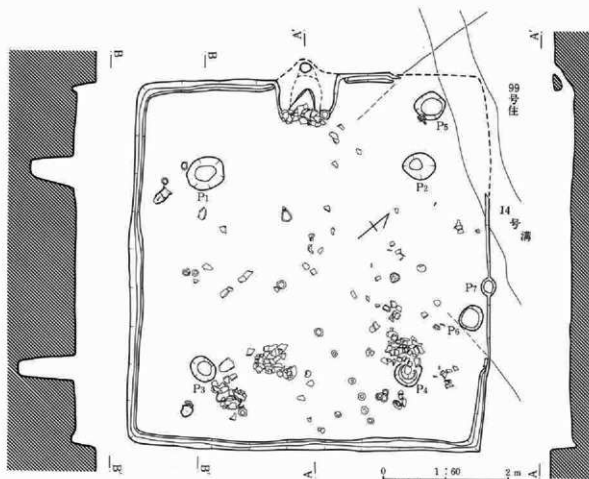
第89図 100号住居跡
