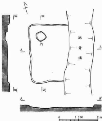
第112図 129号住居跡
