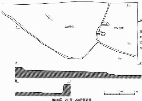
第186図 227号・228号住居跡
