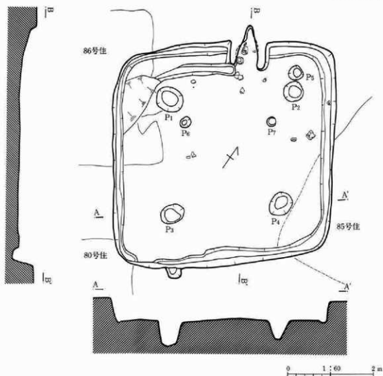
第76図 84号住居跡
