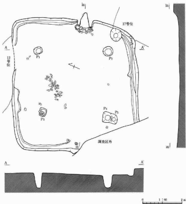
第23図 18号住居跡
