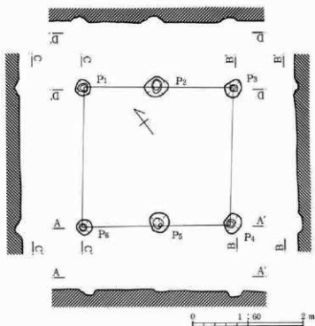
第212図 21号掘立柱建物跡
