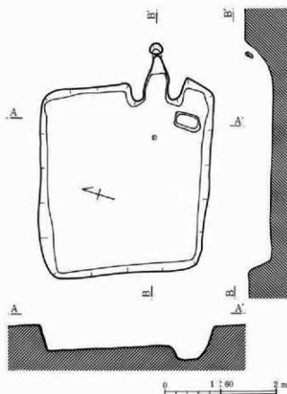
第16図 11号住居跡
