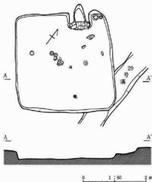
第108図 124号住居跡
