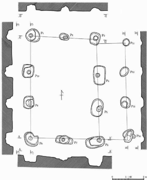
第205図 14号掘立柱建物跡
