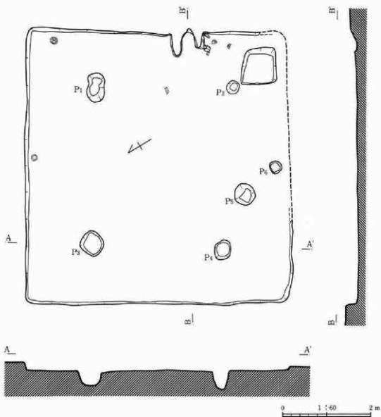
第136図 156号住居跡
