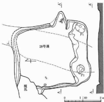
第111図 128号住居跡
