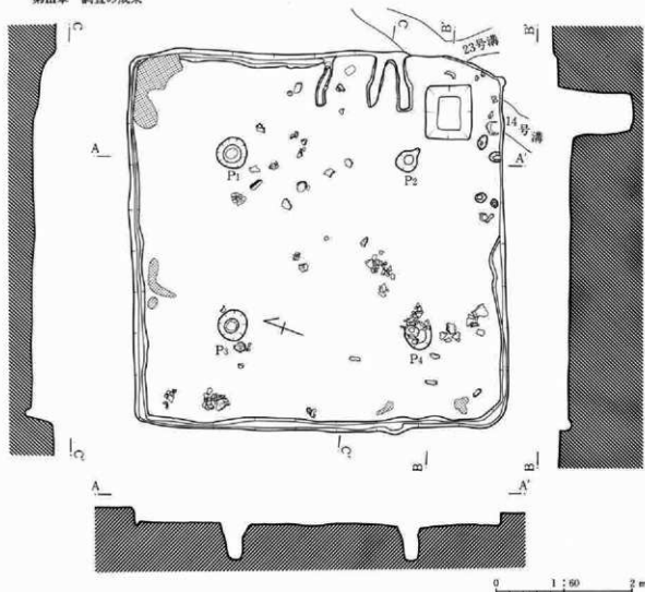
第58図 63号住居跡
