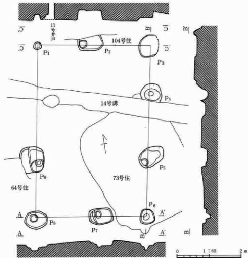
第210図 19号掘立柱建物跡
