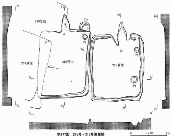
第177図 215号・216号住居跡
