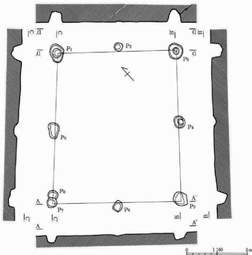
第206号 15号掘立柱建物跡
