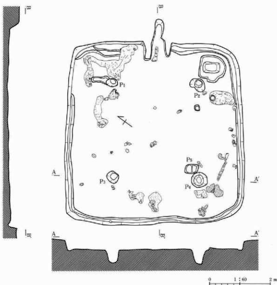
第109図 125号住居跡
