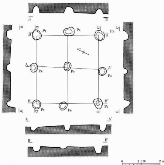
第194図 2号掘立柱建物跡
