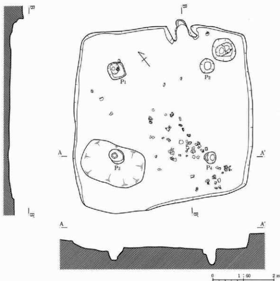
第43図 45号住居跡
