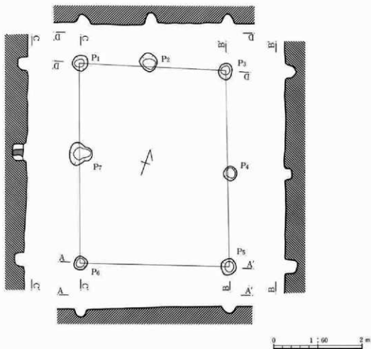
第193図 1号掘立柱建物跡
