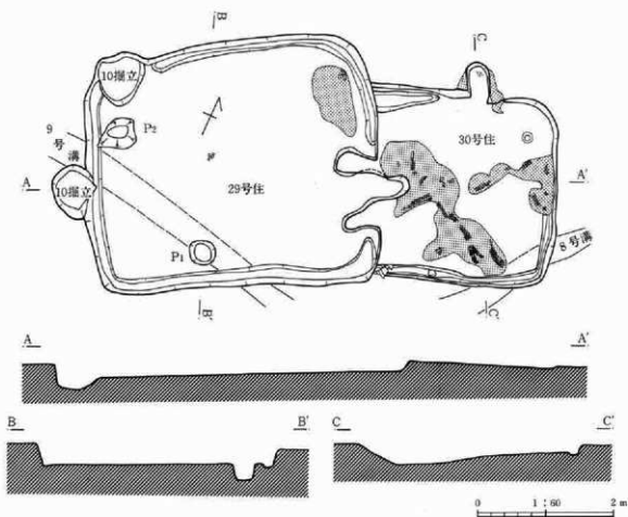
第33図 29号・30号住居跡
