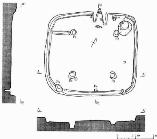
第116図 134号住居跡
