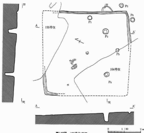
第140図 166号住居跡
