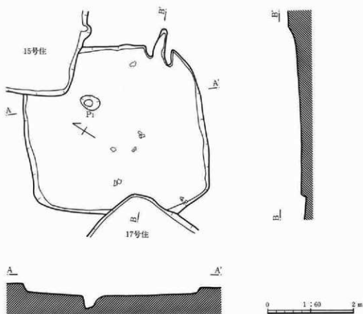
第21図 16号住居跡
