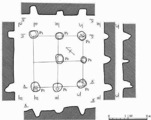
第198図 7号掘立柱建物跡
