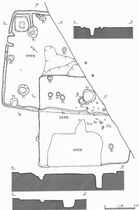
第106図 120号・121号住居跡
