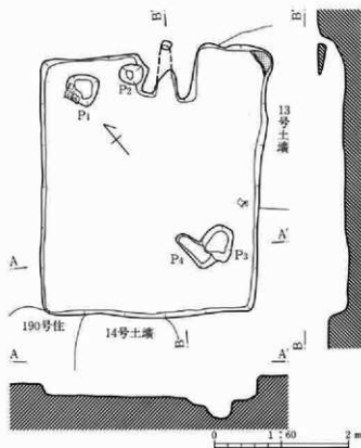
第158図 187号住居跡
