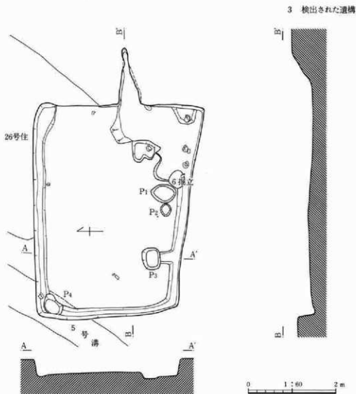
第30図 25号住居跡
