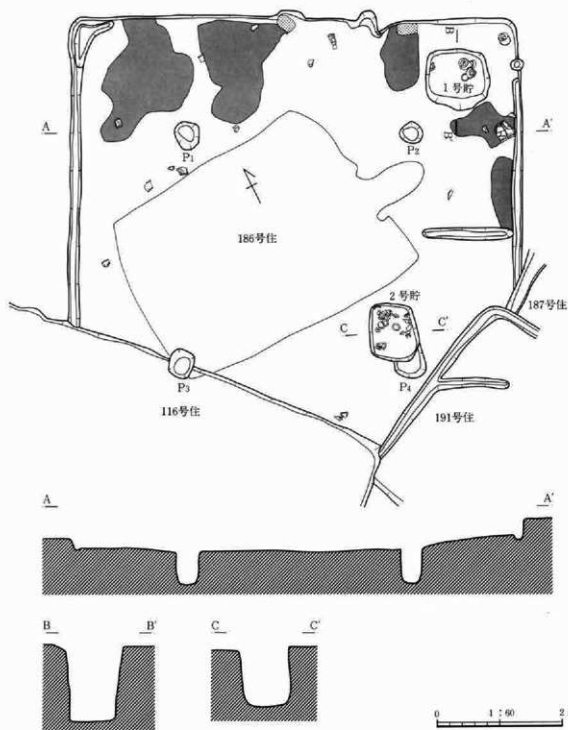
第161図 190号住居跡
