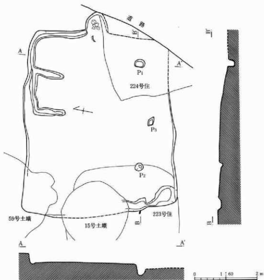
第181図 222号住居跡
