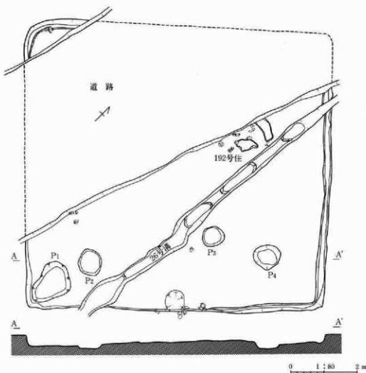
第102図 116号・192号住居跡
