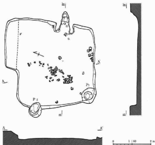
第75図 83号住居跡
