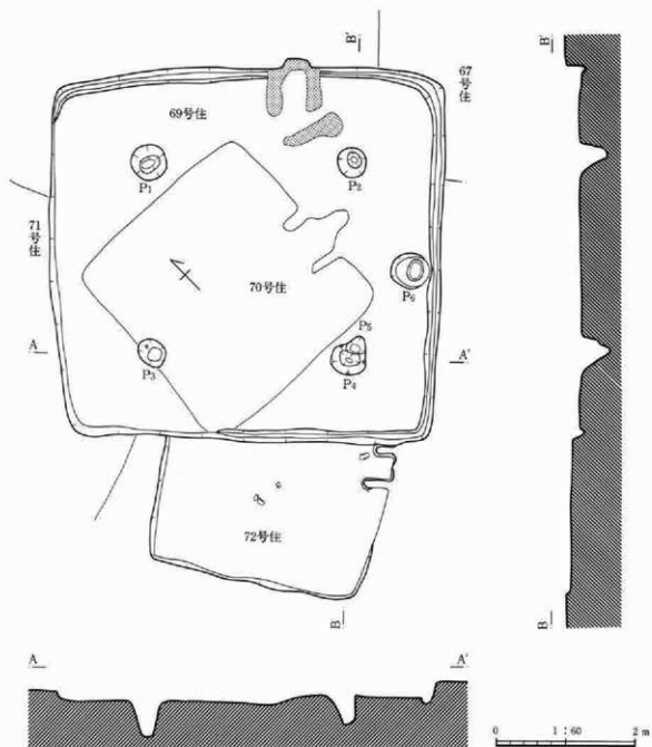
第63図 69号・72号住居跡
