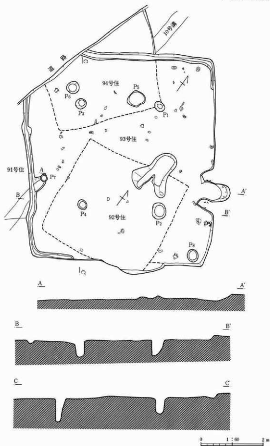
第83図 92号・93号・94号住居跡
