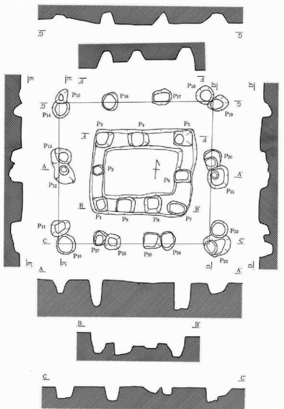
第195図 3号掘立柱建物跡
