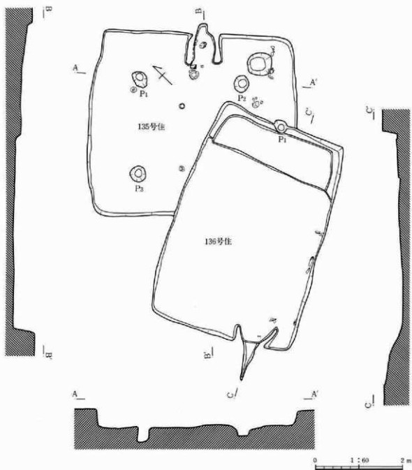
第117図 135号・136号住居跡
