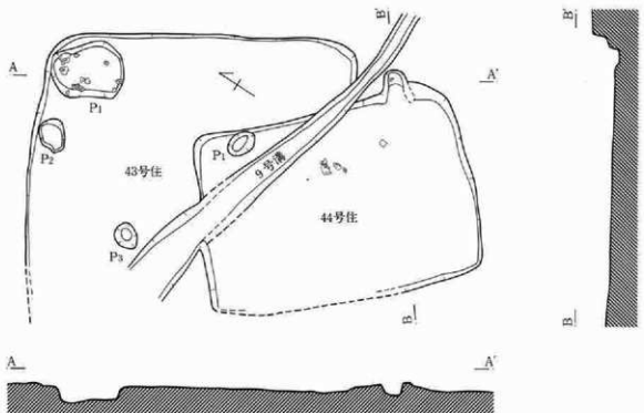
第42図 43号・44号住居跡
