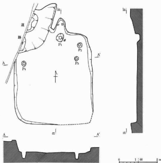
第11図 6号住居跡
