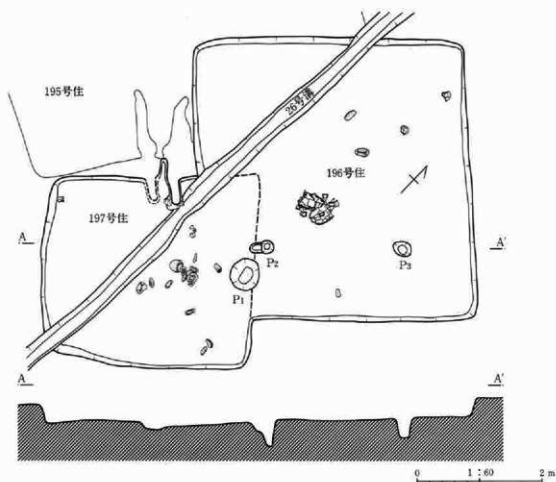
第165図 196号・197号住居跡
