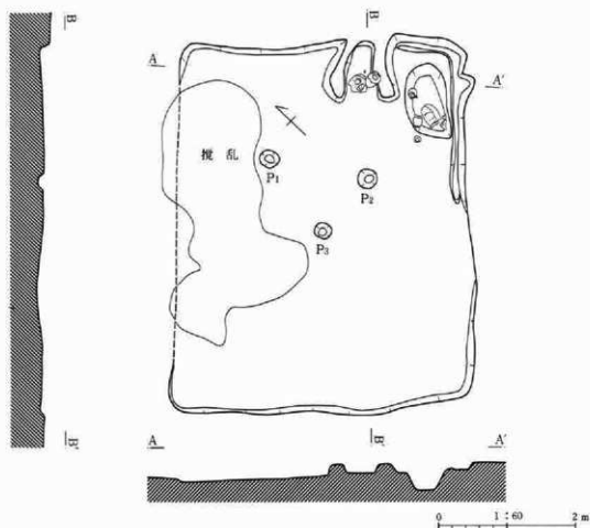
第19図 234号住居跡
