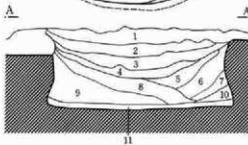
7号土壇 1. 茶褐色土。現耕作土に近似。 2. 黒褐色砂質土。 3. 灰褐色砂質土。 4. 黒色砂質土。白色粘土含む。 5. 灰褐色砂質土。炭化物含む。 6. 黒褐色土。ロームを多く含む。 7. 灰褐色土。 8. 白色粘土。 9. 黄褐色土。ロームを含む。 10. 9層とほぼ同一。 11. 白色粘土 底付近に炭化物が堆積。
