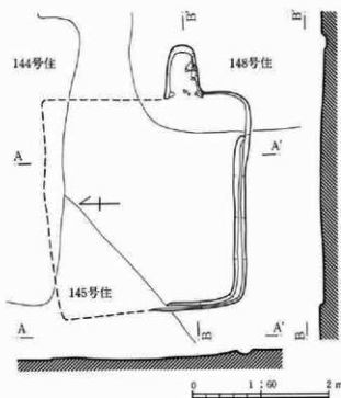
第123図 142号住居跡
