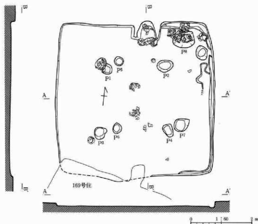
第144図 170号住居跡
