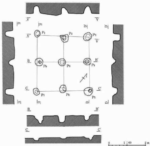
第208図 17号掘立柱建物跡
