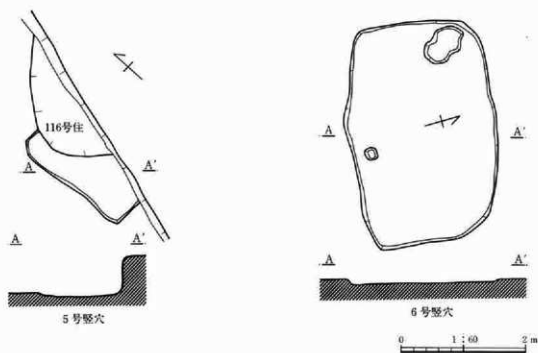
第221回 堅穴遺構(2)
