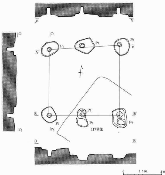
第218図 28号掘立柱建物跡
