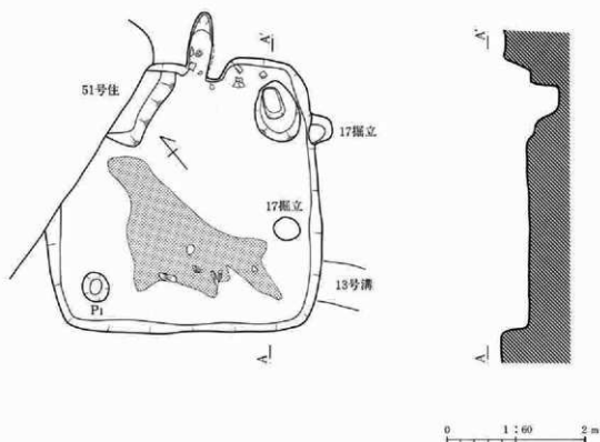
第48図 50号住居跡
