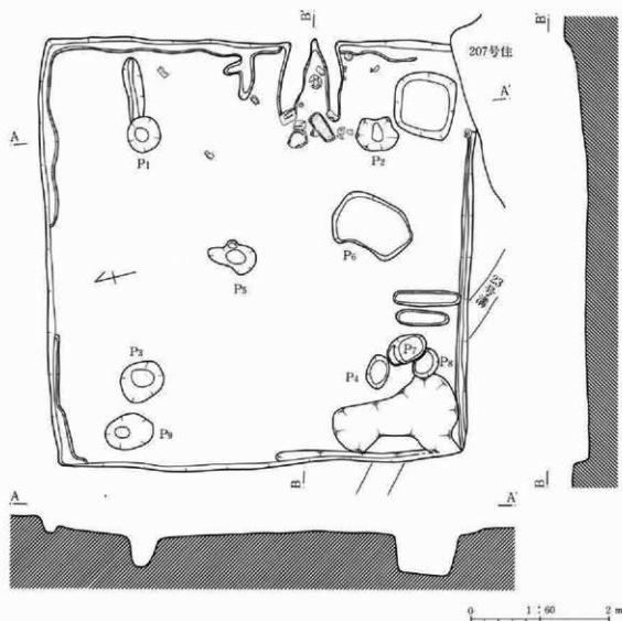
第170図 206号住居跡
