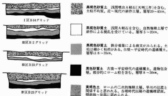
第3図 基本土層
