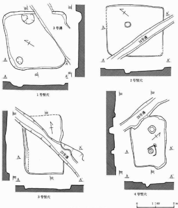
第220図 竪穴遺構(1)
