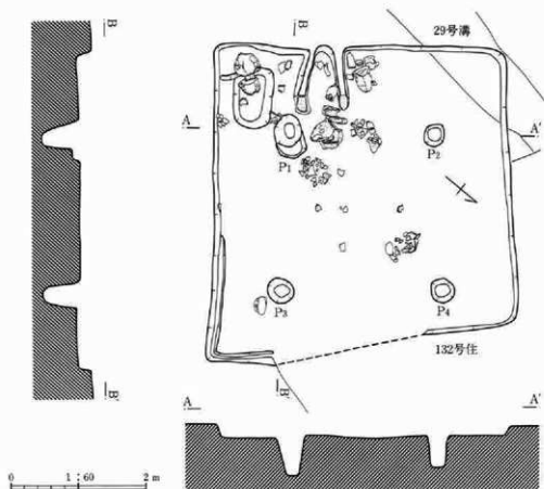
第113図 131号住居跡
