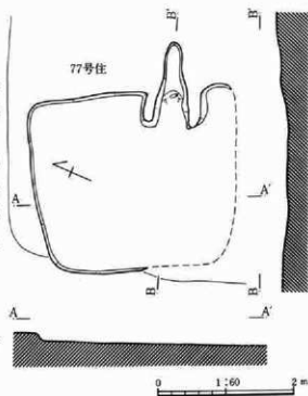
第69図 76号住居跡
