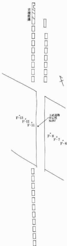
第243図 隣接地トレンチ設定図 1/600
