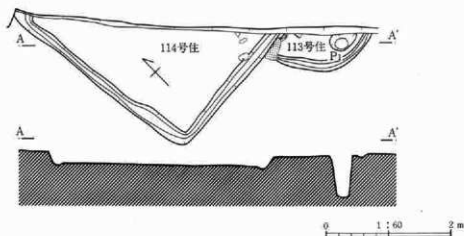
第98図 113号・114号住居跡
