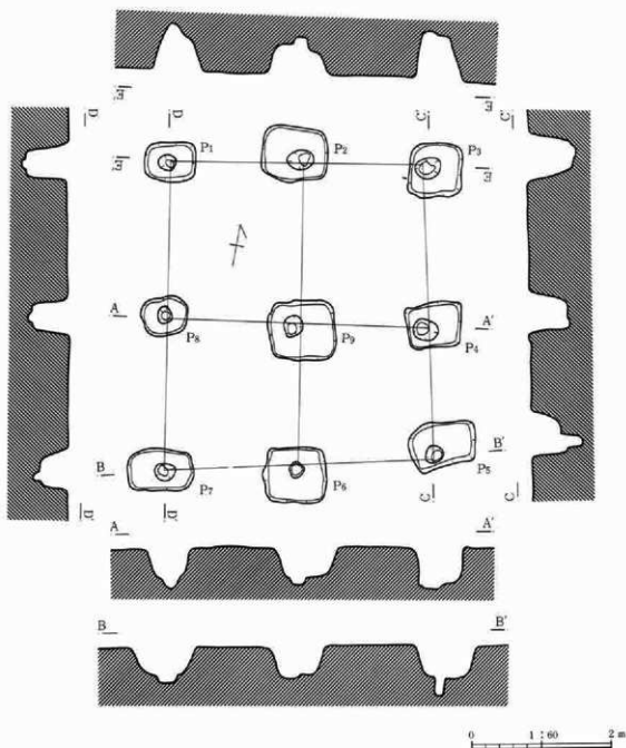
第204図 13号掘立柱建物跡
