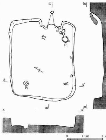
第12図 7号住居跡
