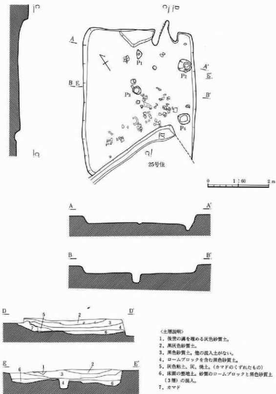
第31図 26号住居跡
