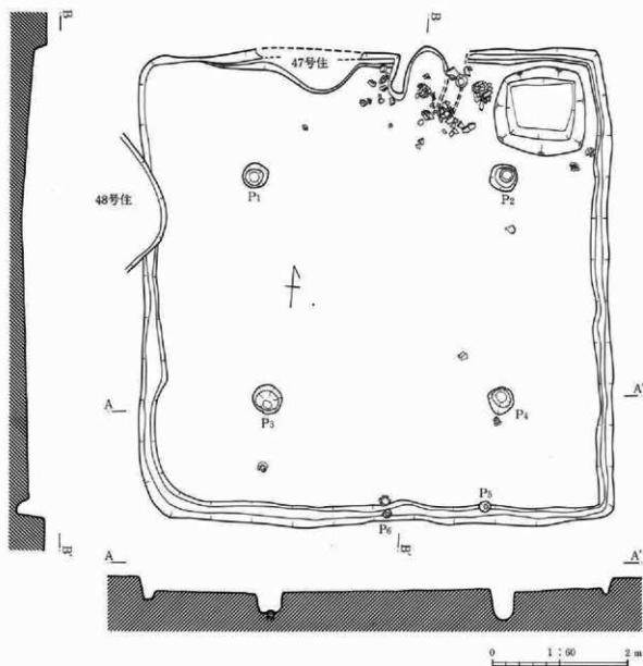
第44図 46号住居跡
