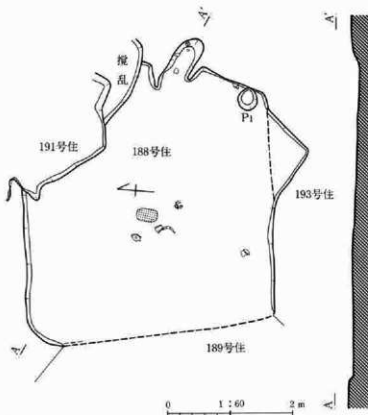
第159図 188号・193号住居跡
