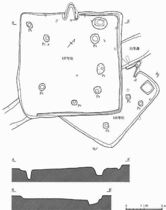
第110図 126号・127号住居跡
