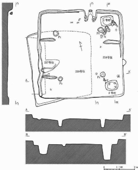
第178図 217号・218号・219号住居跡
