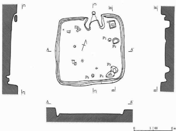
第6図 1号住居跡
