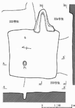
第180図 221号住居跡
