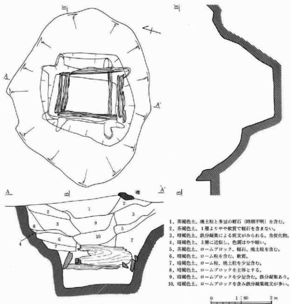
第232図 10号井戸跡
