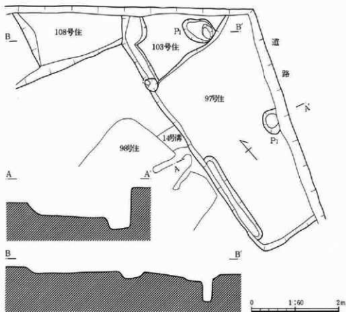
第86図 97号・103号・108号住居跡
