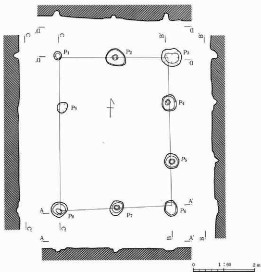
第211図 20号掘立柱建物跡
