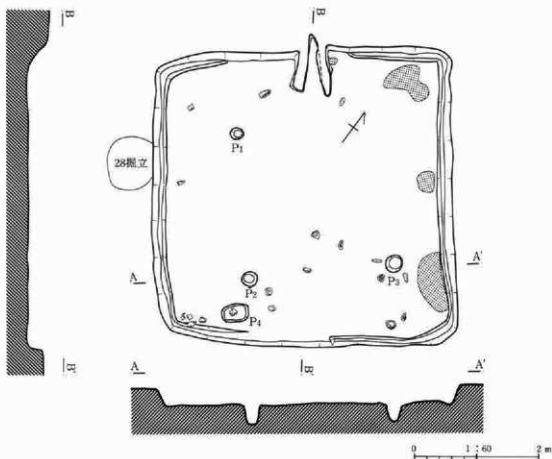
第104図 118号住居跡
