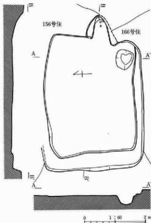
第135図 155号住居跡
