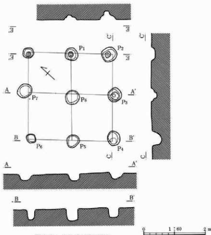
第209図 18号掘立柱建物跡
