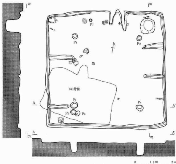
第120図 139号住居跡
