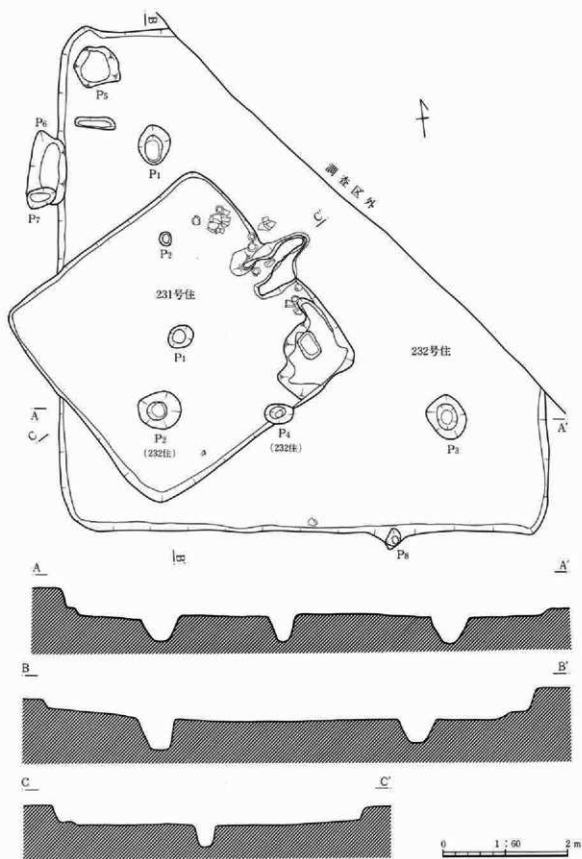
第189図 231号・232号住居跡
