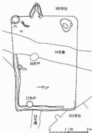
第156図 184号住居跡
