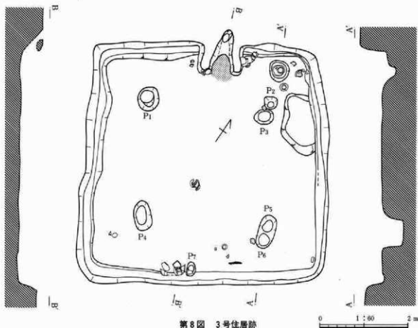
第8図 3号住居跡
