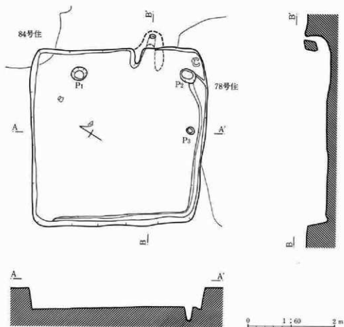
第72図 80号住居跡
