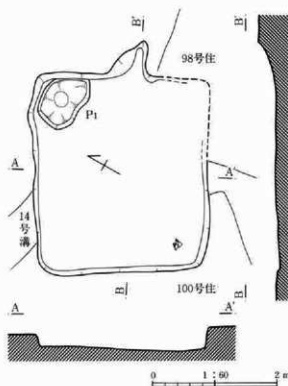
第91図 102号住居跡
