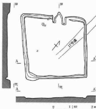
第152図 180号住居跡
