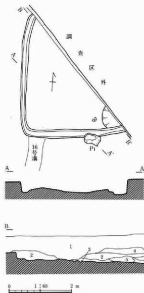
第97図 112号住居跡及び土層断面図
