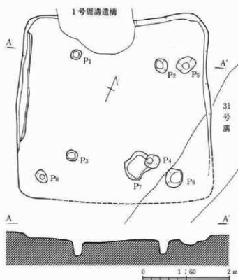
第188図 230号住居跡
