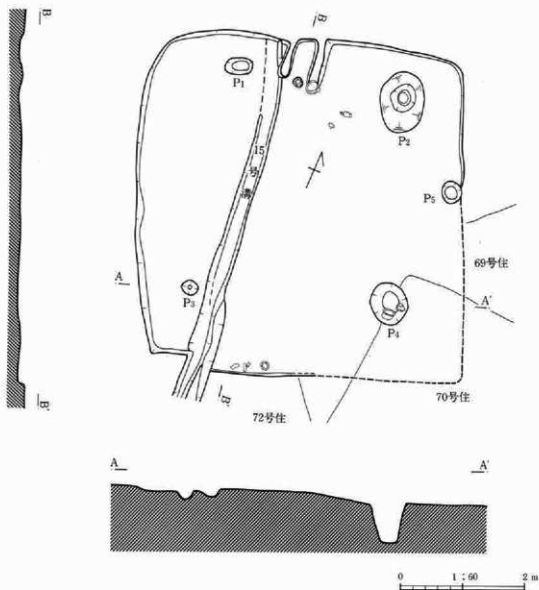
第65図 71号住居跡
