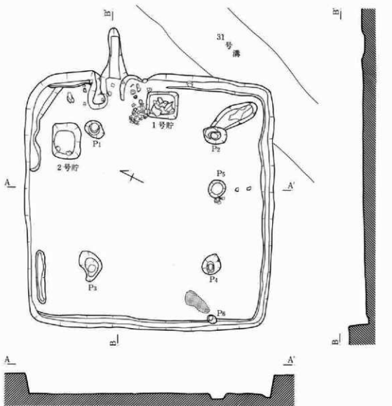
第185図 226号住居跡
