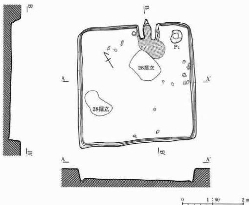
第103図 117号住居跡
