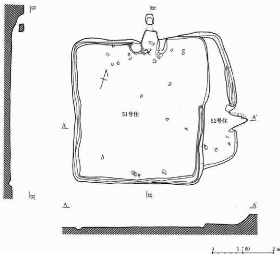
第49図 51号・52号住居跡
