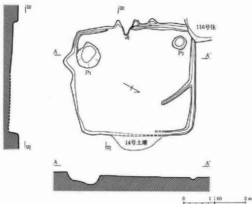
第162図 191号住居跡
