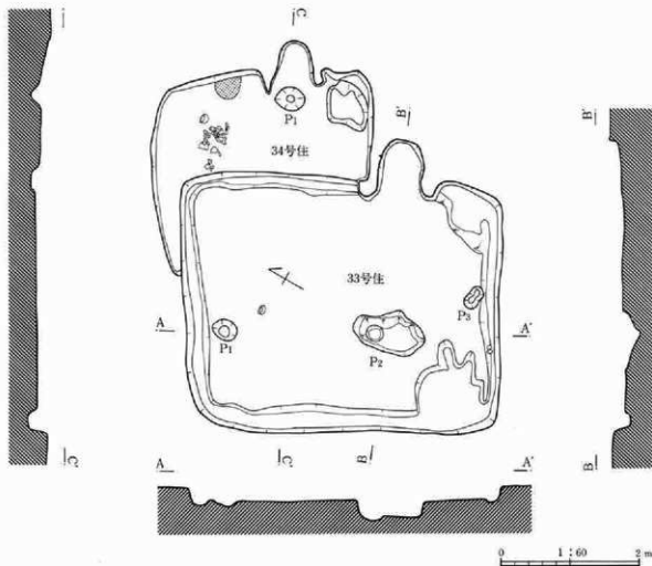
第36図 33号・34号住居跡
