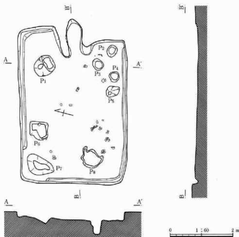
第32図 27号住居跡
