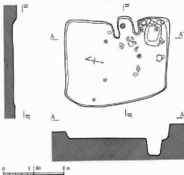
第13図 8号住居跡
