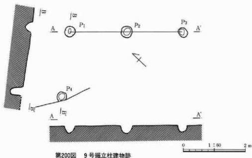
第200図 9号掘立柱建物跡
