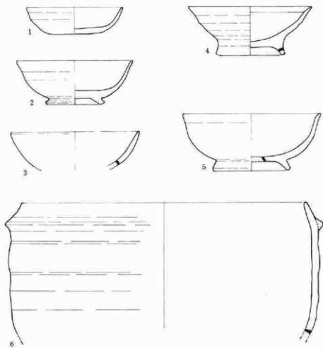
挿図11 3号住居出土遺物
