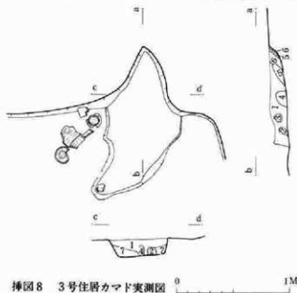
挿図8 3号住居カマド実測図
