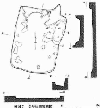
挿図7 3号住居実測図
