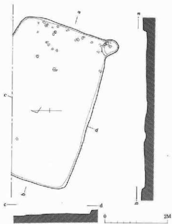
挿図5 2号住居実測図
