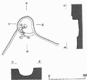
挿図6 2号住居カマド実測図
