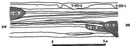
第7図 縄文時代土層断面図（Bトレンチ北側）
