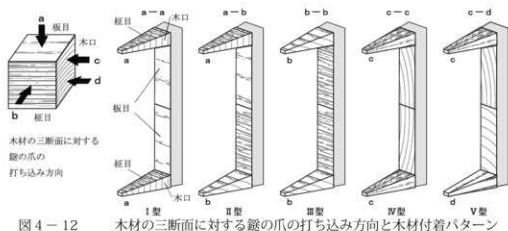
図4-12 木材の三断面に対する鑿の爪の打ち込み方向と木材付着パターン
