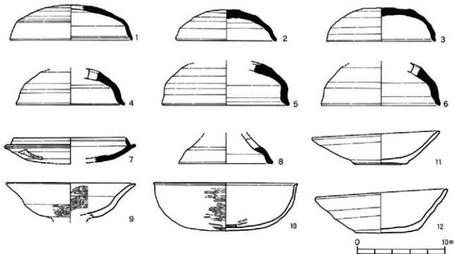
第55図 8号墳出土土器実測図
