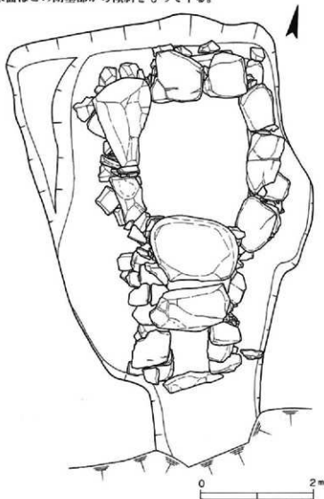
第93図 14号墳石室平面図
