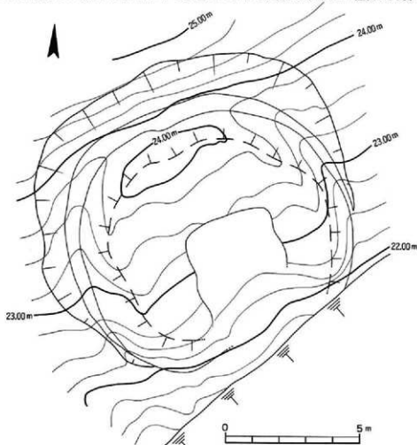
第82図 13号墳墳丘遺存状況図
