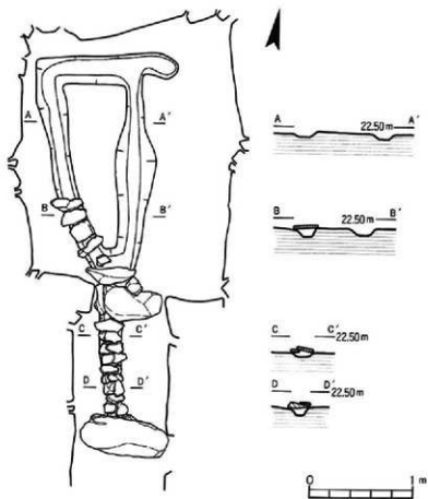
第96图 14号墳石室内排水施設実測図
