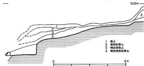
第23図 15号墳Nトレンチ土層断面図
