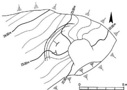
第76図 12号墳墳丘遺存状況図
