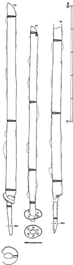
第111図 15号墳出土鉄刀実測図
