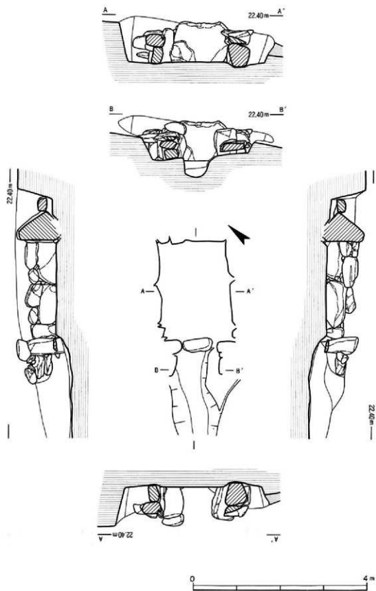
第13图 14号墳石室実測図
