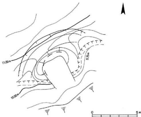
第28図 16号墳墳丘遺存状況図
