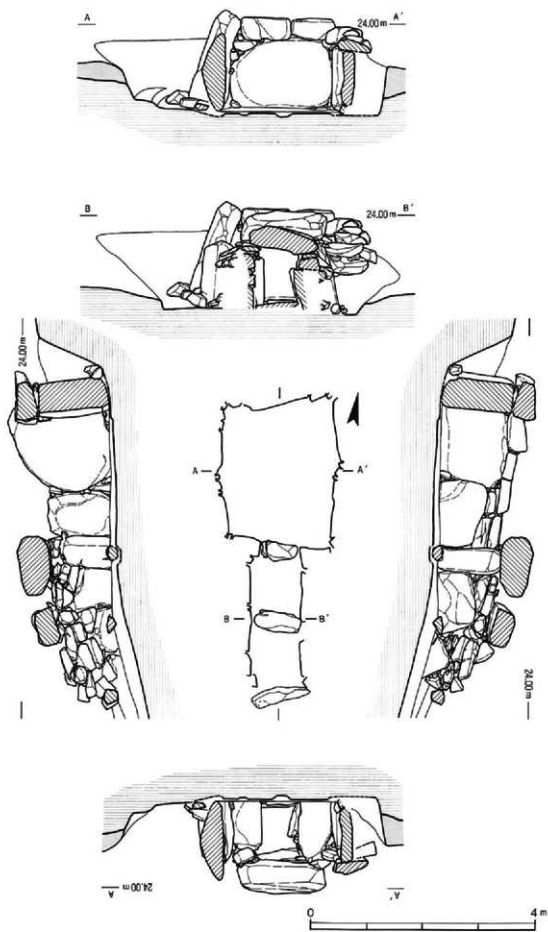
第94图 14号墳石室実測図
