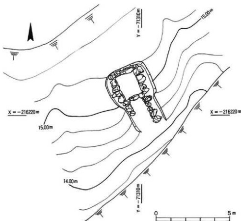
第36図 6号墳調査後地形測量図
