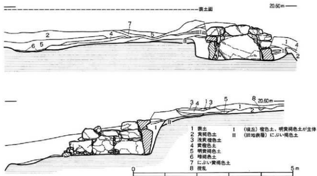
第70図 11号墳墳丘土層断面図
