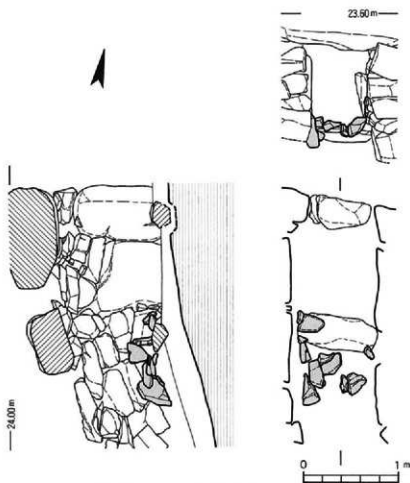
第95图 14号填閉塞施設実測図
