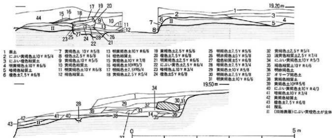
第45図 7号墳トレンチ土層断面図
