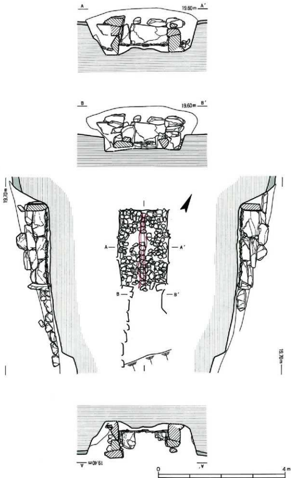
第61图 9号填石室实测图
