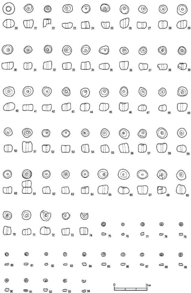
第20图 14号墳出土小玉笏测图
