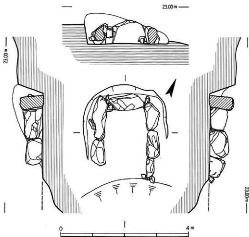
第79図 12号墳石室実測図
