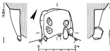
第25図 15号墳石室実測図
