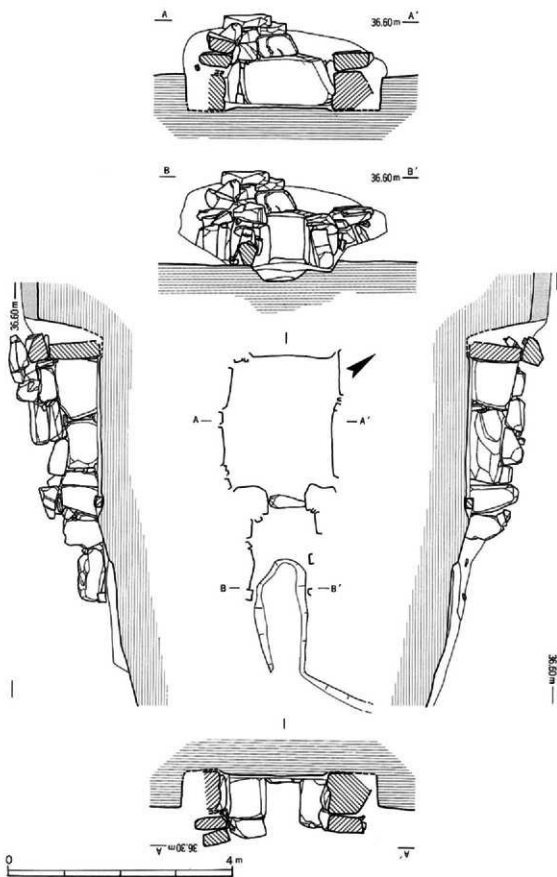
第108图 15号填石室夷冢图
