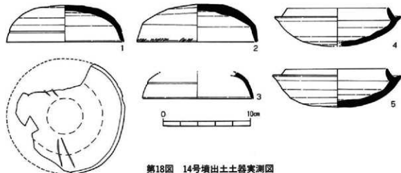
第18図 14号墳出土土器実測図
