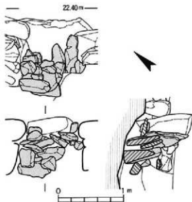
第14図 14号墳閉塞施設実測図
