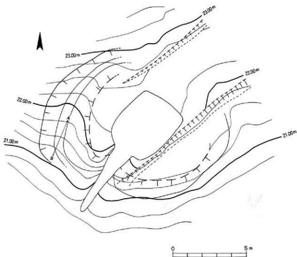
第9図 14号墳墳丘遺存状況図
