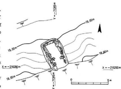
第50図 8号墳調査後地形測量図
