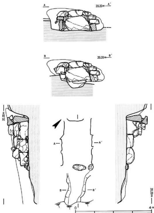
第73図 11号墳石室実測図
