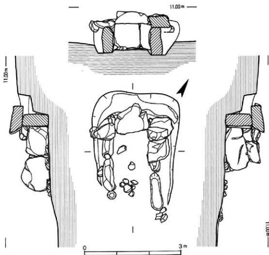
第31図 16号墳石室実測図
