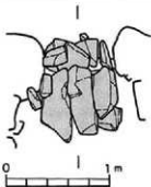
第107図 15号墳閉塞施設実測図
