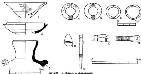
第75図 11号墳出土遺物実測図
