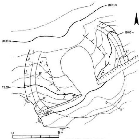
第56图 9号墳墳丘遺存状況図
