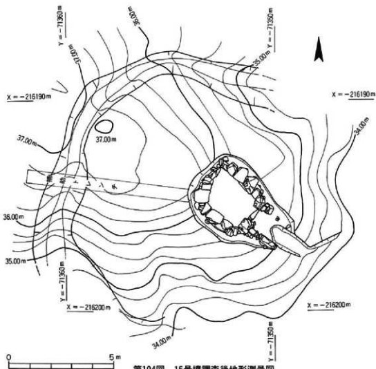
第104図 15号墳調査後地形測量図
