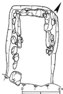
第52図 8号墳石室平面図
