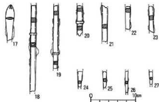
第88図 13号墳出土鉄製品実測図
