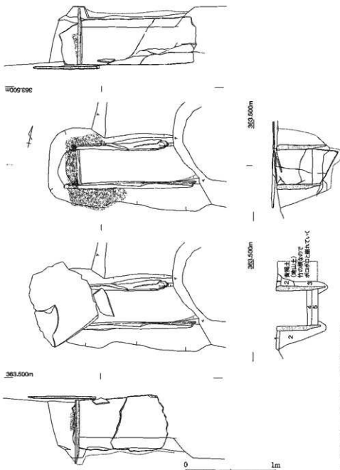
第18図 第3次調査4号石棺実測図 (1/30)
