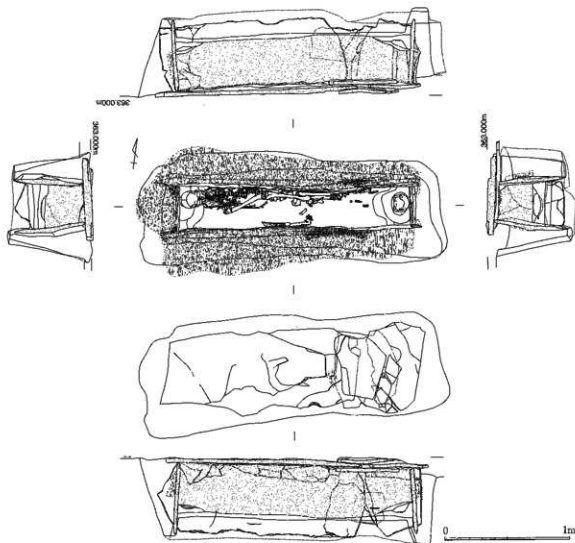
第17図 第3次調査3号石棺実測図 (1/30)
