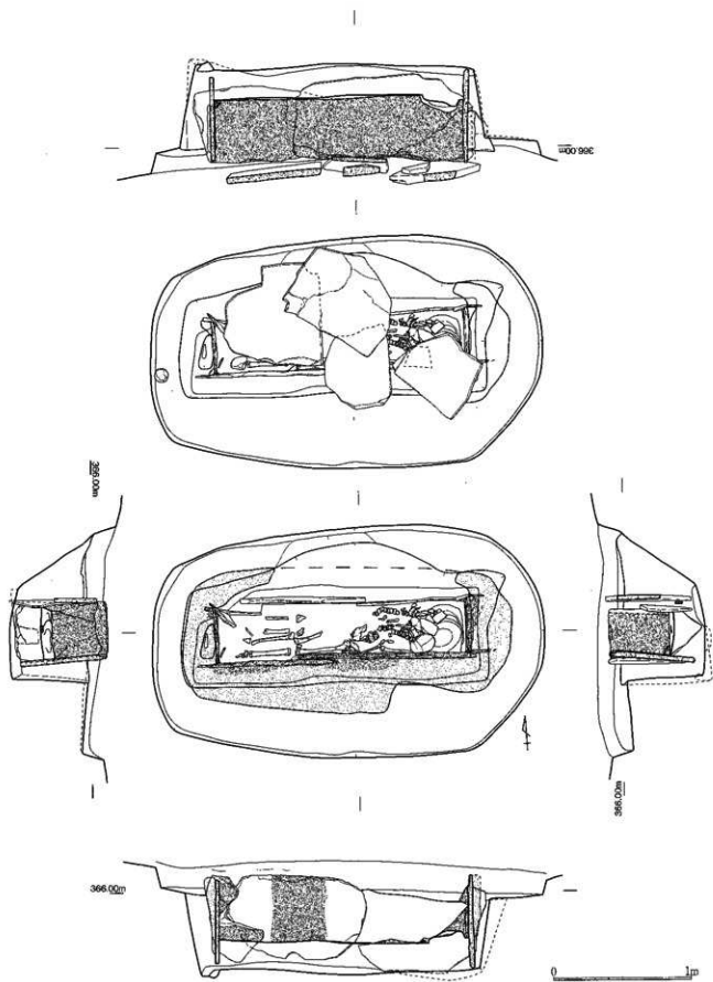
第9図 第2次調査1号石棺実測図 (1/30)
