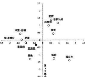
図2 主成分分析結果 (女性)
