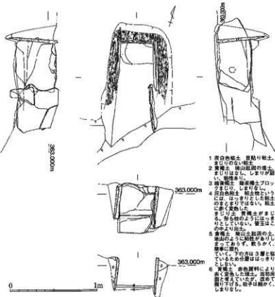
第19図 第3次調査5号石棺実測図 (1/30)
