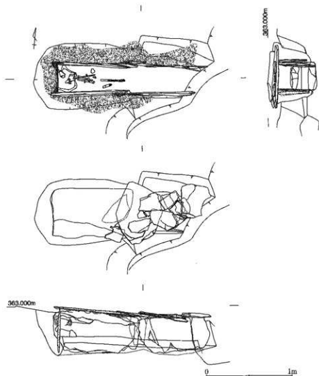
第15図 第3次調査1号石棺実測図 (1/30)
