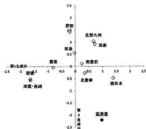
図1 主成分分析結果 (男性)
