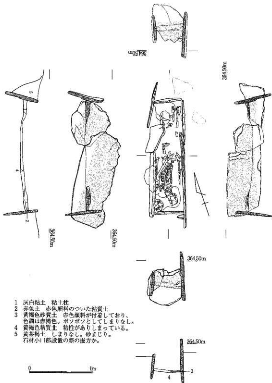
第6図 第1次調査2号石棺実測図（1/30）
