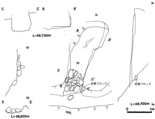
第5図 2号墓実測図
