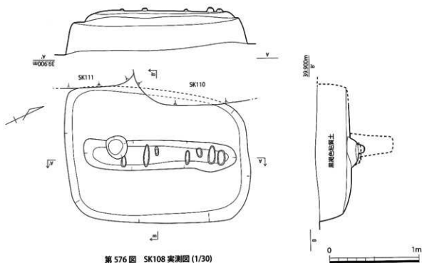
第 576 图 SK108 实测图 (1/30)
