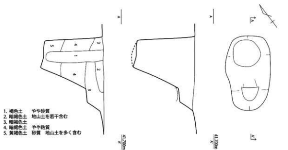
第 662 図 SK204 実測図 (1/30)
