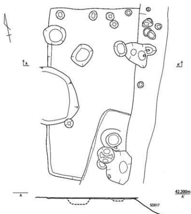
第 443 図 SH166 実測図
