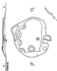
第 534 图 SK064 实测图 (1/30)
