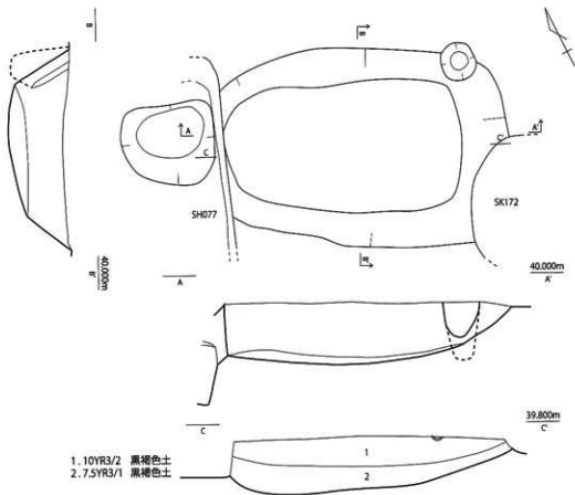
第 630 图 SK171 实测图 (1/30)
