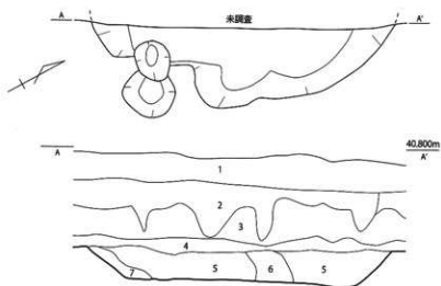
第 621 図 SK161 実測図 (1/30)
