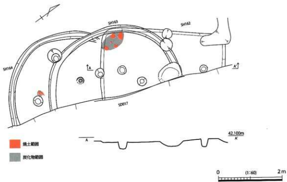
第 439 图 SH162 · SH163 · SH164 实测图
