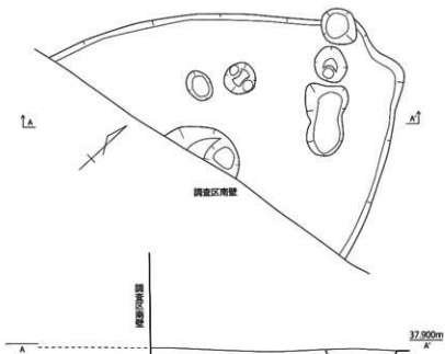
第 472 图 SK002 突测图 (1/30)
