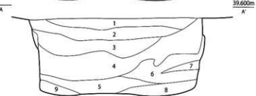
第571図 SK103実測図(1/30)
