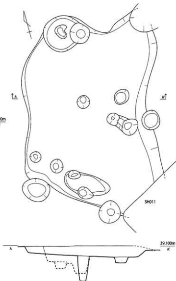
第 531 图 SK061 实测图 (1/30)
