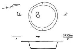
第 549 図 SK081 実測図 (1/30)
