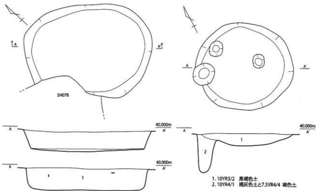
第 628 図 SK169 実測図 (1/30)
