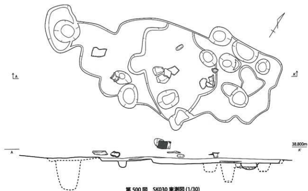
第 500 图 SK030 实测图 (1/30)
