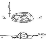
第598図 SK134 実測図 (1/30)
