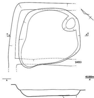
第 582 図 SK114 実測図 (1/30)
