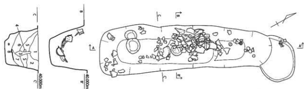
第 649 図 SK191 実測図 (1/30)
