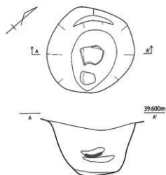
第 569 图 SK101 实测图 (1/30)
