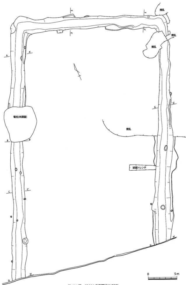
第 694 図 SD006 実測図③(1/200)
