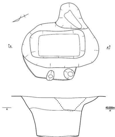
第 659 图 SK201 实测图 (1/30)
