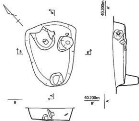
第 652 図 SK194 実測図 (1/30)
