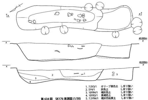
第 634 図 SK176 実測図 (1/30)
