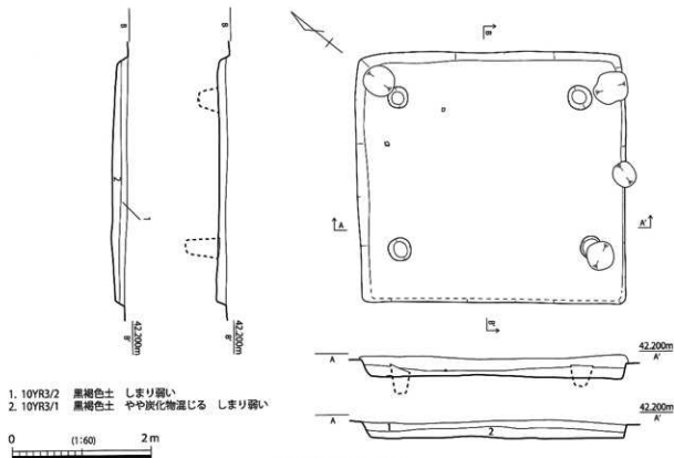
第 451 図 SH175 実測図
