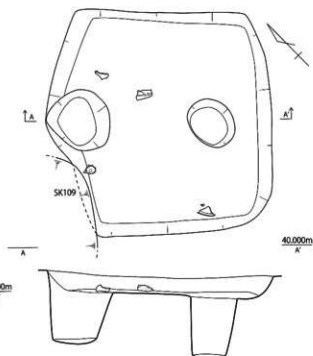
第 575 图 SK107 实测图 (1/30)
