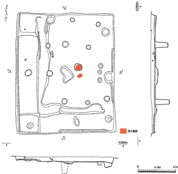
第 446 図 SH169 実測図
