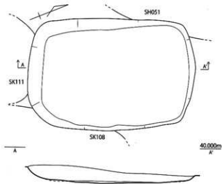
第 578 図 SK110 実測図 (1/30)
