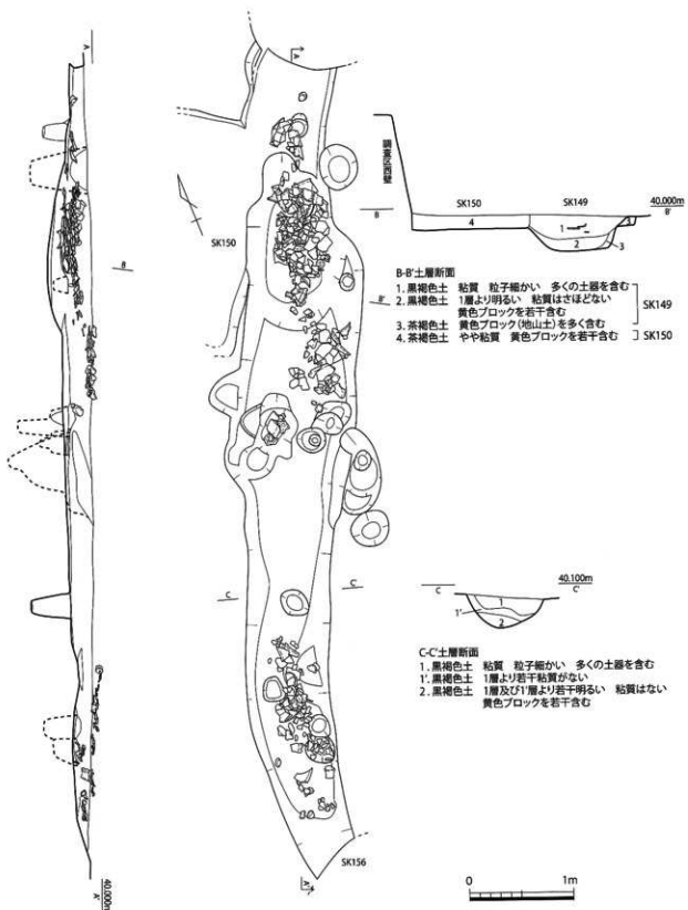
第 612 図 SK149 実測図 (1/40)
