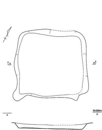
第 500 图 SK030 实测图 (1/30)
