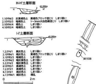
第703図 SD018 実測図②(1/80)
