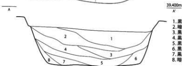
第 553 図 SK085 実測図 (1/30)
