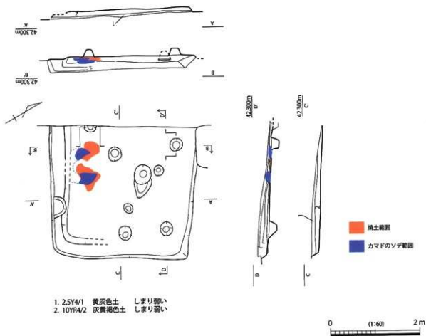
第 460 図 SH184 実測図
