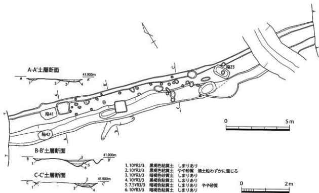
第 707 図 SD023 実測図 (1/150・1/80)
