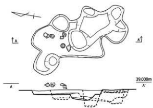
第507图 SK037 实测图(1/30)
