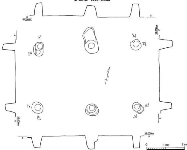
第 464 图 SB002 实测图
