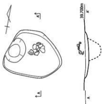
第 564 图 SK096 实测图 (1/30)
