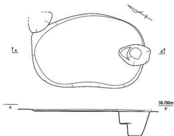
第 498 图 SK028 实测图 (1/30)
