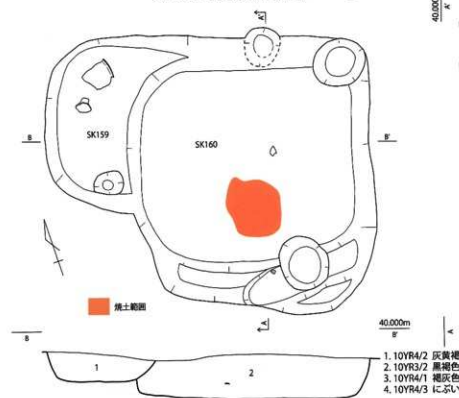
第 620 図 SK159・160 実測図 (1/30)
