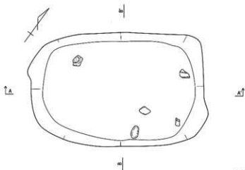
第570図 SK102実測図(1/30)
