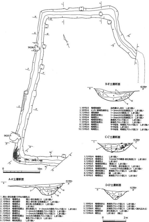
第705図 SD022 実測図①(1/250・1/80)
