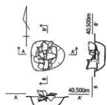
第 654 図 SK196 実測図 (1/30)
