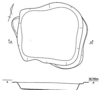
第 516 图 SK046 实测图 (1/30)
