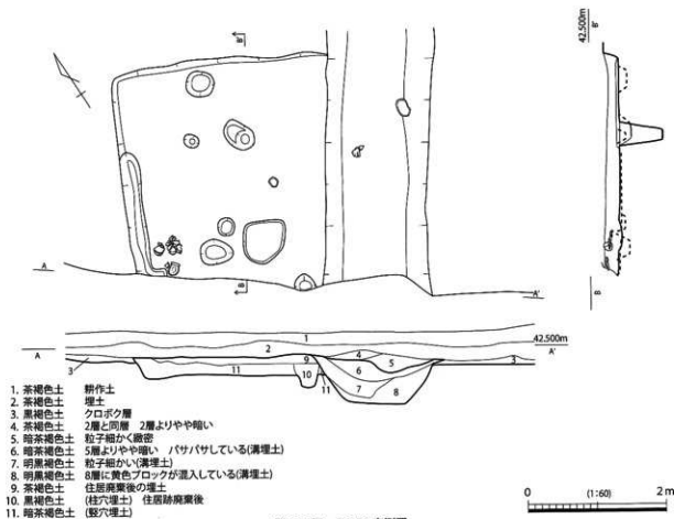
第 452 図 SH178 実測図
