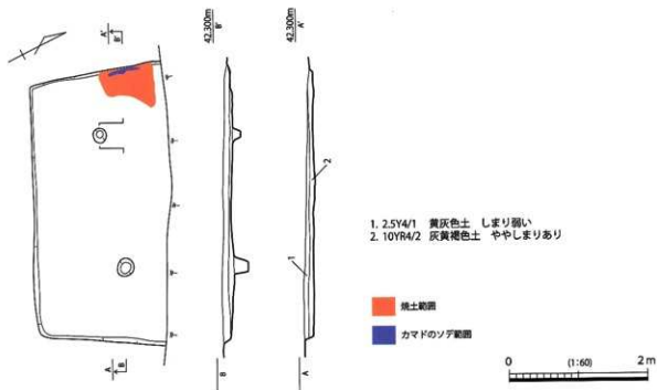
第 459 図 SH183 実測図
