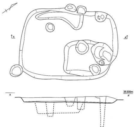
第 543 图 SK075 实测图 (1/30)
