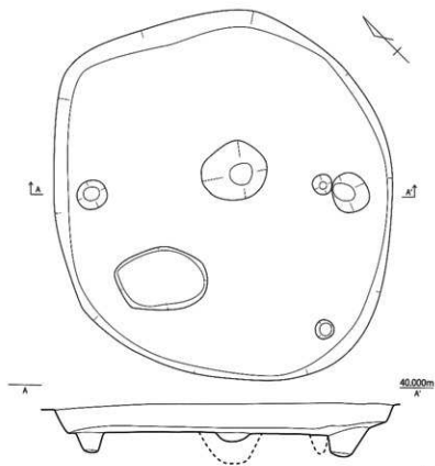
第 586 图 SK118 实测图 (1/30)
