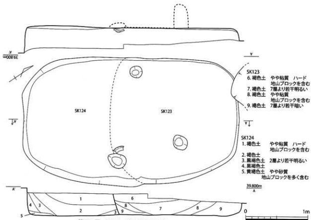
第591図 SK123・124 実測図 (1/30)
