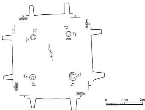
第 463 图 SB001 实测图
