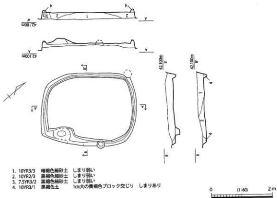
第 456 図 SH180 実測図
