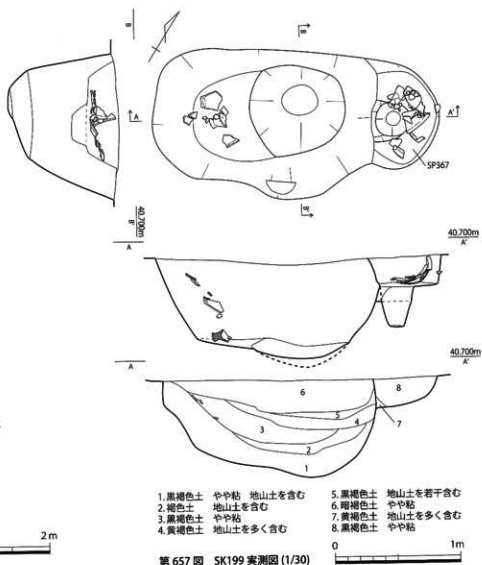
第 657 図 SK199 実測図 (1/30)
