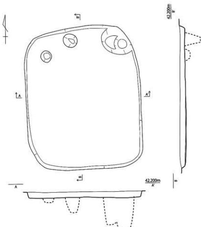
第 676 図 SK218 実測図 (1/30)
