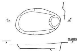
第 475 图 SK005 突测图 (1/30)
