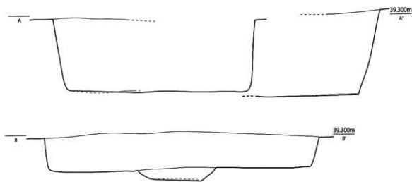
第 542 图 SK072・073・074 实测图 (1/30)
