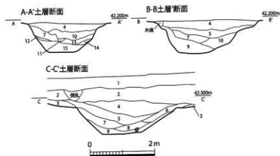
第 697 図 SD015 実測図①(1/300・1/80・1/30)
