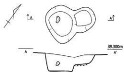
第 551 図 SK083 実測図 (1/30)
