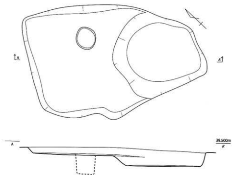
第 557 图 SK089 实测图 (1/30)
