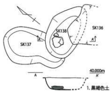
第601図 SK137・138 実測図 (1/30)
