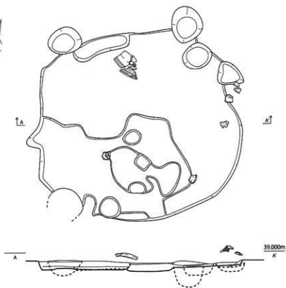
第 520 图 SK050 实测图 (1/30)
