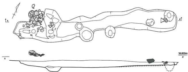
第 486 图 SK016 实测图 (1/30)
