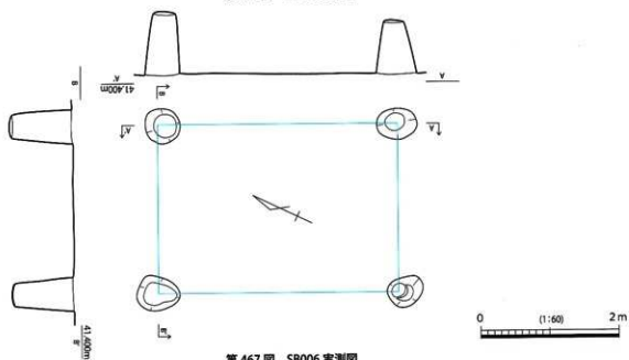
第 467 图 SB006 实测图
