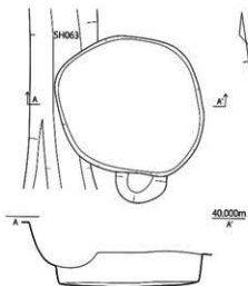
第 614 图 SK151 实测图 (1/30)
