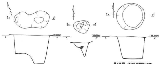
第476図 SK006実測図(1/30)
