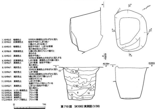
第 710 図 SK1002 実測図 (1/30)
