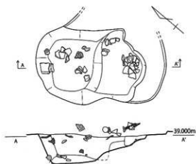
第509图 SK039 实测图(1/30)
