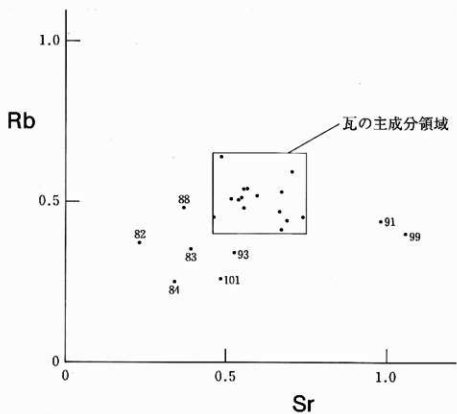
第173図 瓦のRb-Sr分布図
