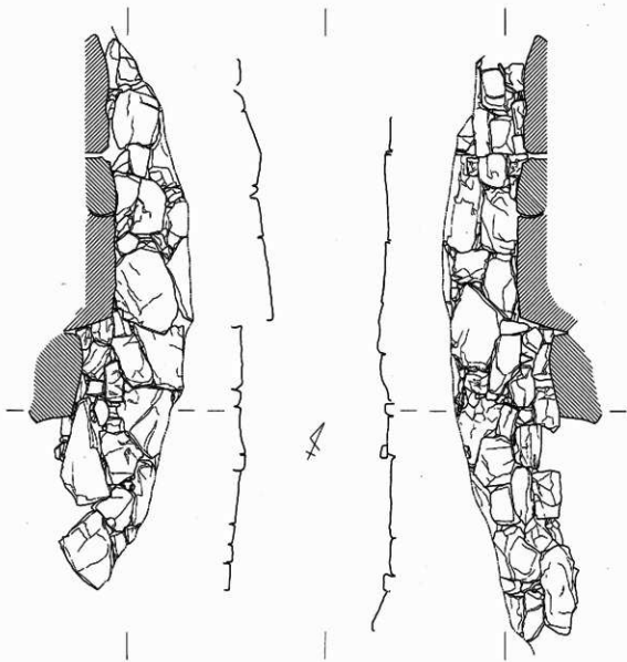
圖112 磨子色山石塔石龕 東面圖
