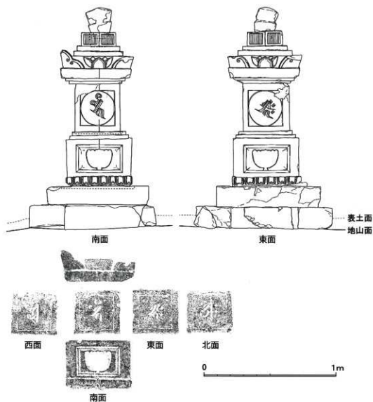
第6図 1号石塔実測図 (1/20)
