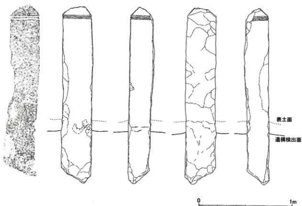
第12図 4号石塔実測図 (1/20)
