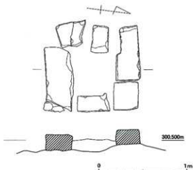
第7図 1号石塔基壇組実測図 (1/30)
