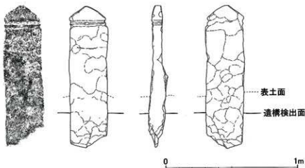
第9図 2号石塔実測図 (1/20)
