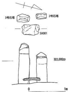
第8図 2・3号石塔とSX001 (1/30)
