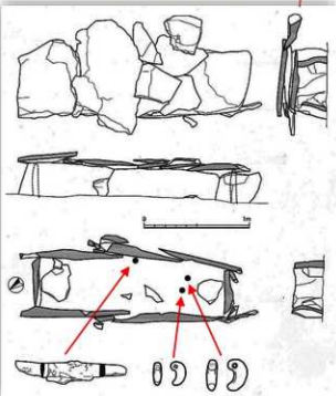
13号石棺の出土状況実測図 (田添夏喜氏の原因をトレース)
