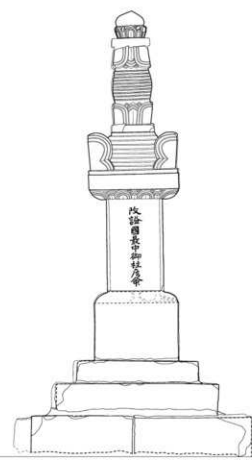
背面図
