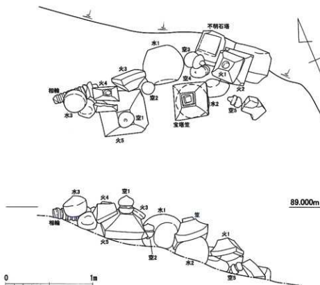
第8図 平田中村地区石造物群実測図 (S=1/30)
