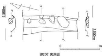
SD2001実測図
