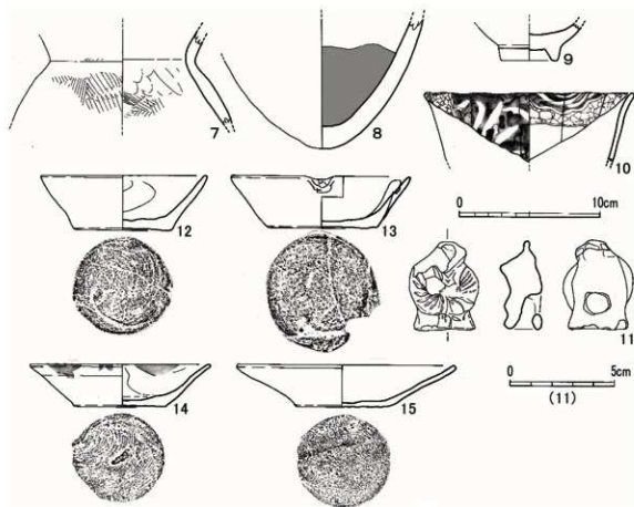
第5図 国・その他機関事業に伴う試掘確認・立会調査出土遺物実測図（1/3・1/2）
