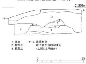
馬場の土手土層断面図(1/50)
