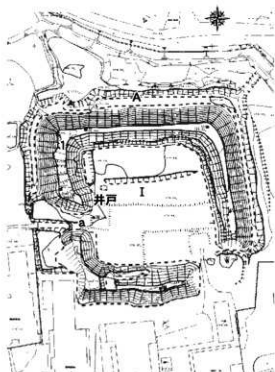
第22図 竹中城 遺構位置図
