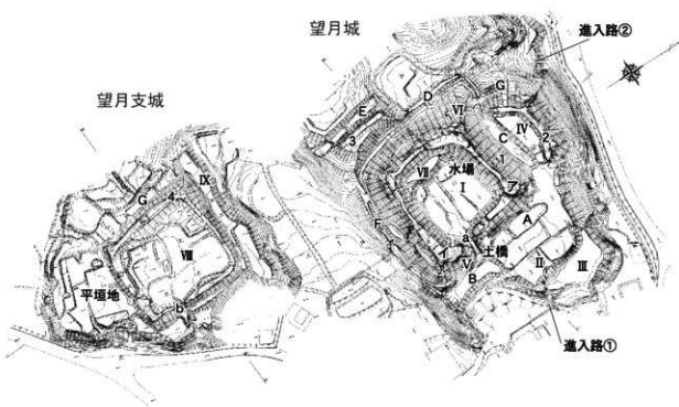
第4図 望月城・望月支城 遺構位置図
