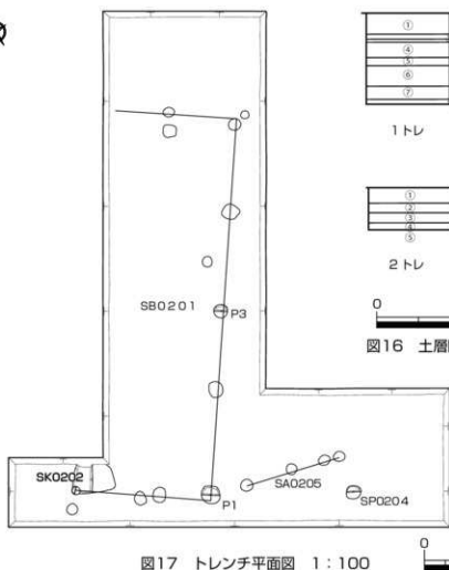
図17 トレンチ平面図 1:100
