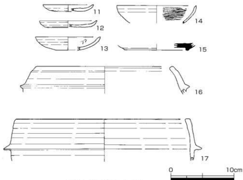
図15 出土遺物 1:3
