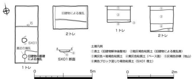
図3 平面図 1:100
