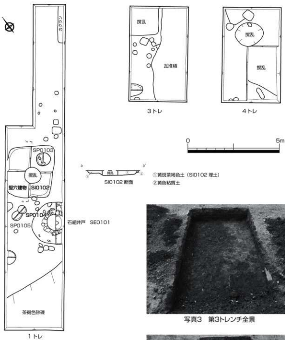
図8 平面図 1:100
