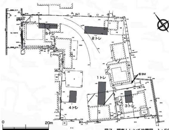
図7 調査トレンチ位置図 1:500
