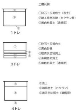
図6 土層断面図 1:50
