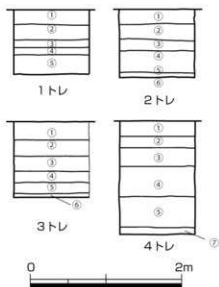
図19 土層断面図 1:50
