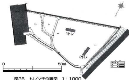
図36 トレンチ位置図 1:1000
