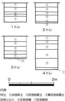
図19 土層断面図 1:50
