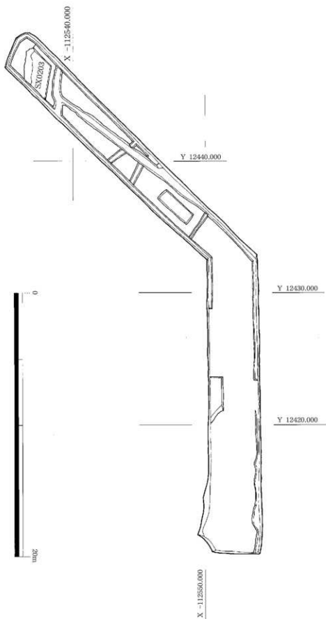
図20 第2トレンチ遺構図 1 : 200
