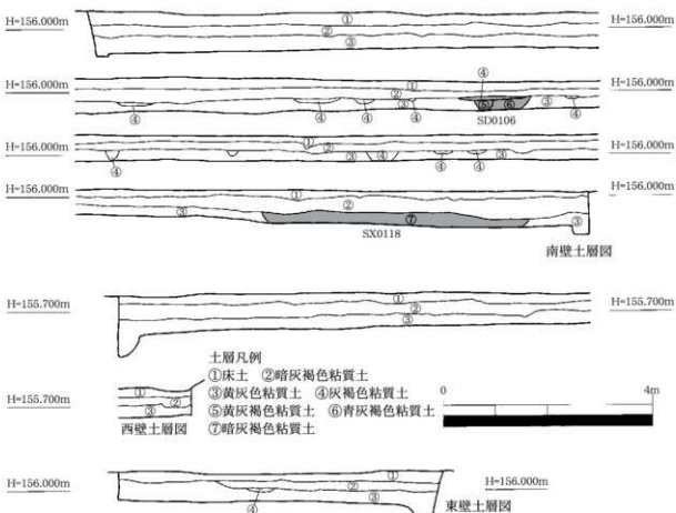
図13 第1トレンチ土層図 1:80
