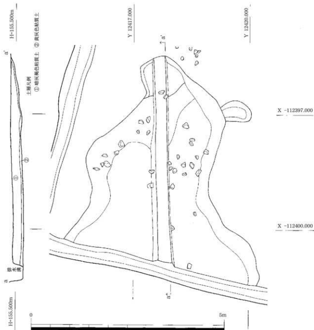
図 16 SX0118 平面図・断面図 1:50
