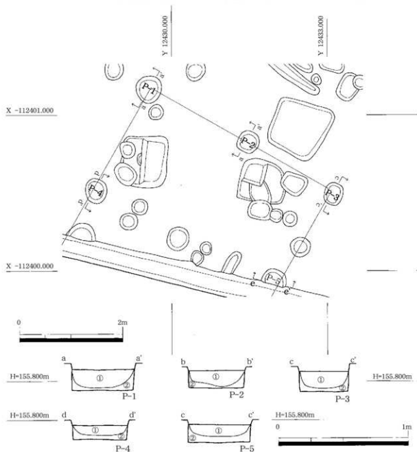
図18 SB0121 平面図 (1:50)・断面図 (1:20)
