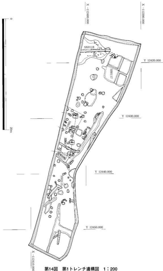
第14図 第1トレンチ遺構図 1:200
