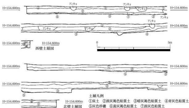
図19 第2トレンチ土層図 1:80
