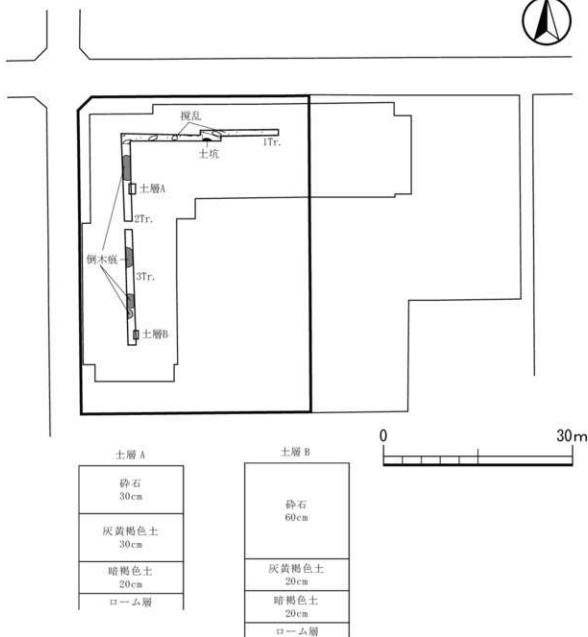
第3図 確認調査平面図・断面図
