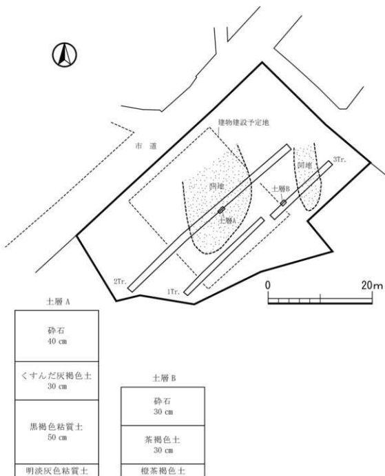
第9図 確認調査平面図・断面図
