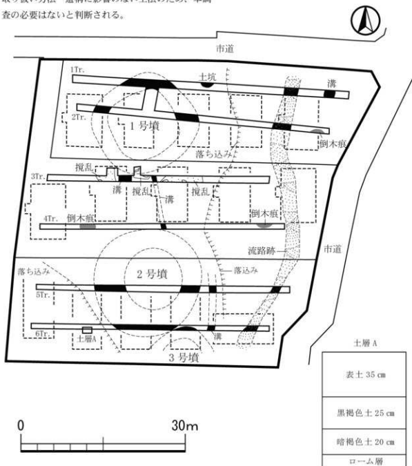
第19図 確認調査平面図・断面図
