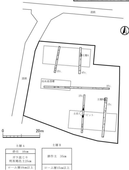
第44図 確認調査平面図・断面図
