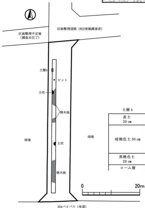
第25図 確認調査平面図・断面図
