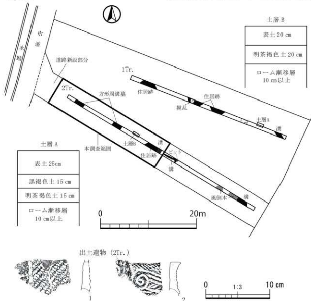
第33図 確認調査平面図・断面図・出土遺物実測図
