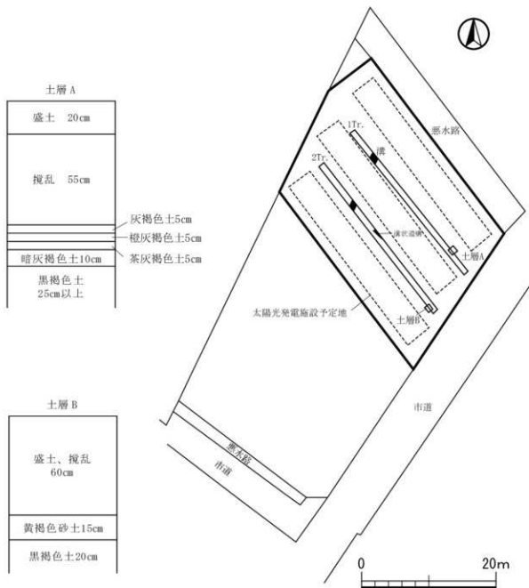
第43図 確認調査平面図・断面図
