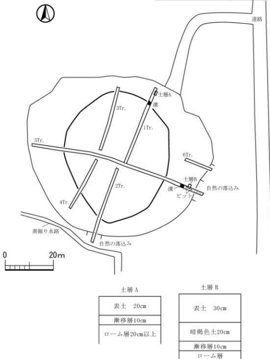
第46図 確認調査平面図・断面図
