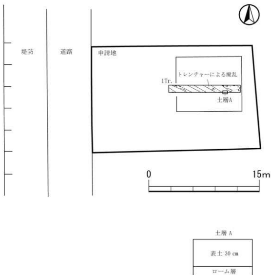
第5図 確認調査平面図・断面図
