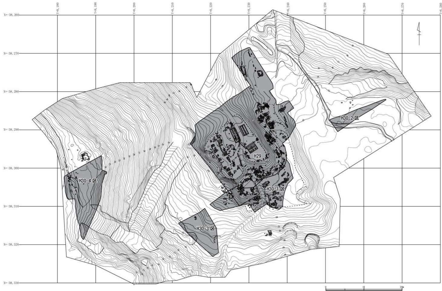
第2図 現況測量図 (縮尺1/300)
