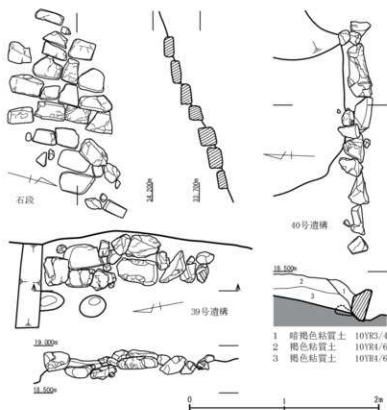
第16図 遺構実測図10 (縮尺1/40)
