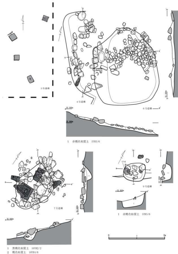
第9図 遺構実測図3 (縮尺1/40)
