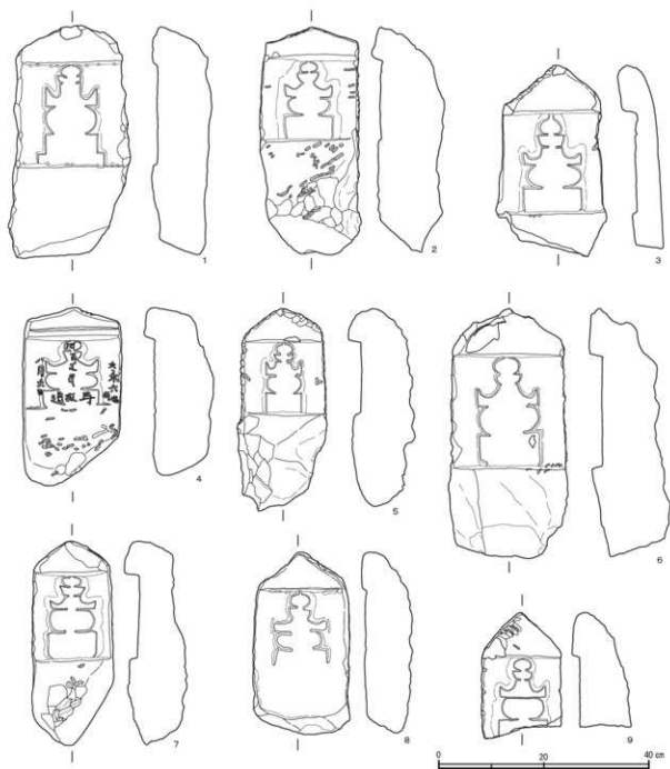
第21図 遺物実測図5 (縮尺1/8)
