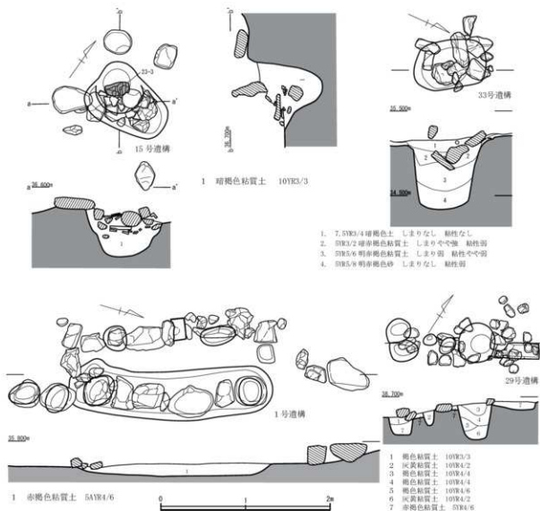
第8図 遺構実測図2 (縮尺1/40)
