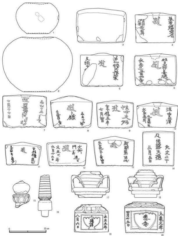
第19図 遺物実測図3 (縮尺1/6)
