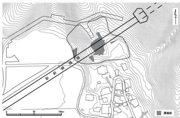
第1図 大蔵北遺跡の位置図（縮尺1/2,000）
