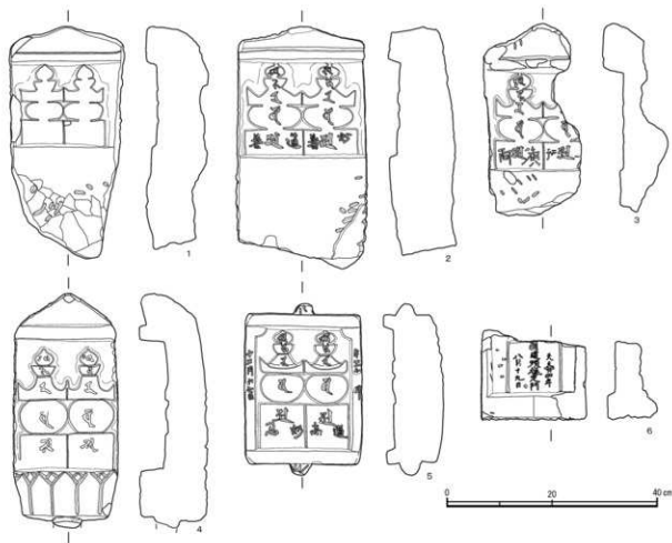
第22図 遺物実測図6 (縮尺1/8)
