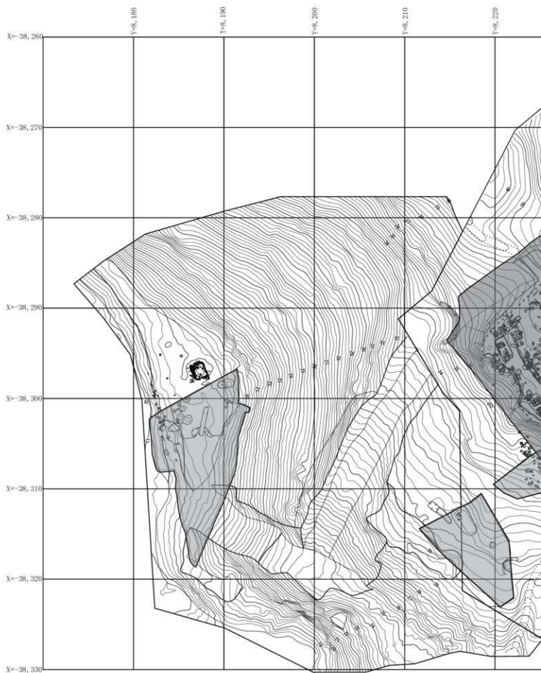
第2図 現況測量図 (縮尺 1 / 300)
