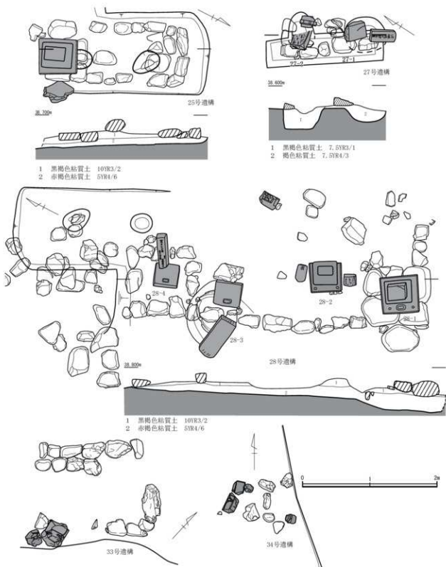
第13図 遺構実測図7 (縮尺1/40)
