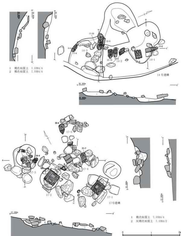
第11図 遺構実測図5 (縮尺1/40)
