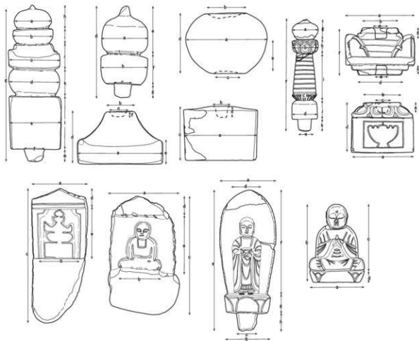
第25図 石遺物計測部位模式図
