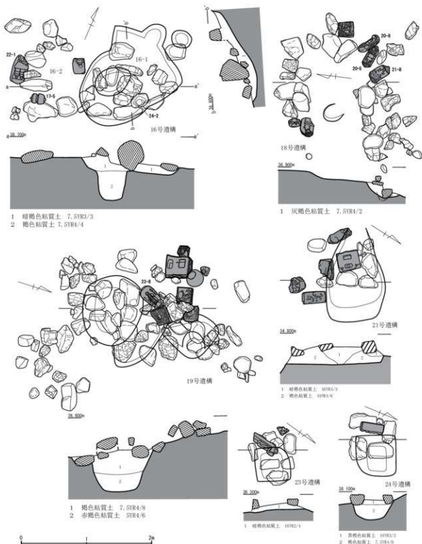
第12図 遺構実測図6 (縮尺1/40)
