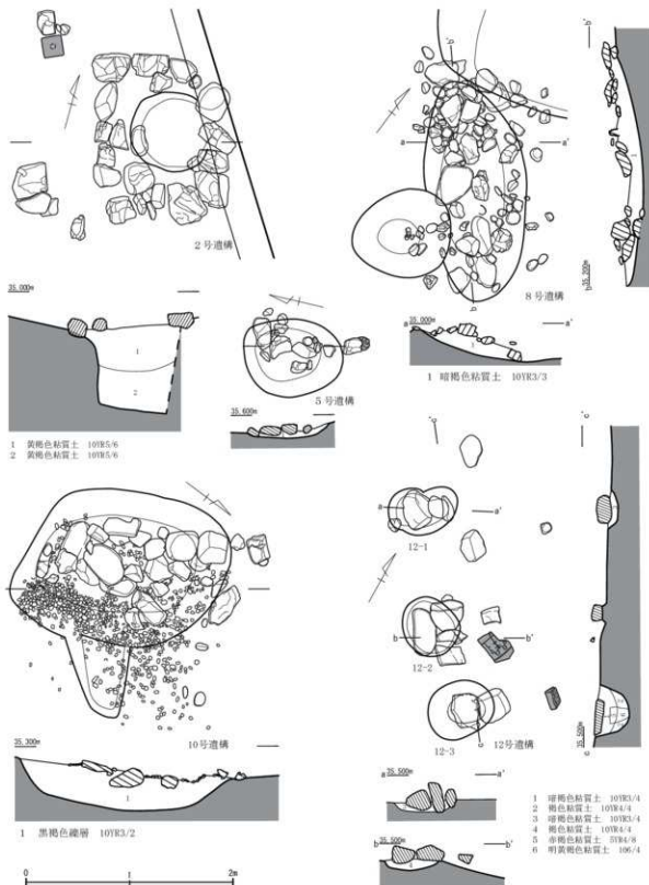
第7図 遺構実測図1 (縮尺1/40)
