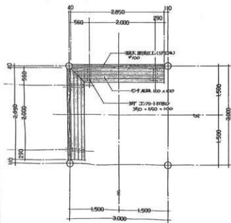
第25図 四角構造図
