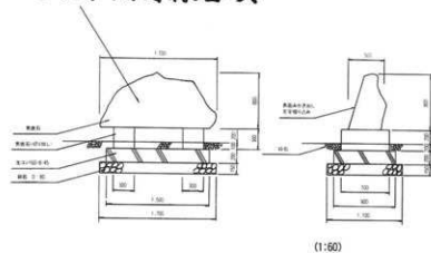
第20図 史跡名称碑構造図
