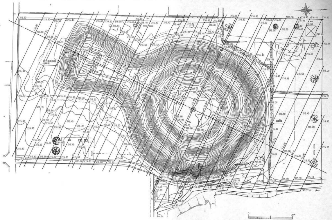
第8図 土工事平面図
