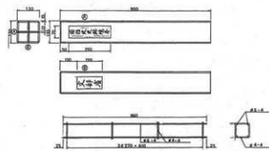
第29図 史跡境界杭構造図
