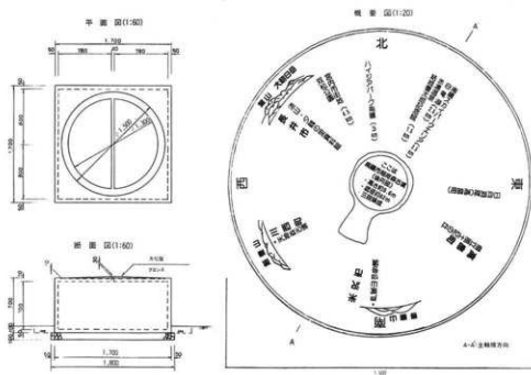
第21図 方位盤構造図
