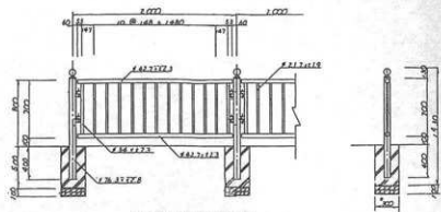
第28図 防護柵構造図
