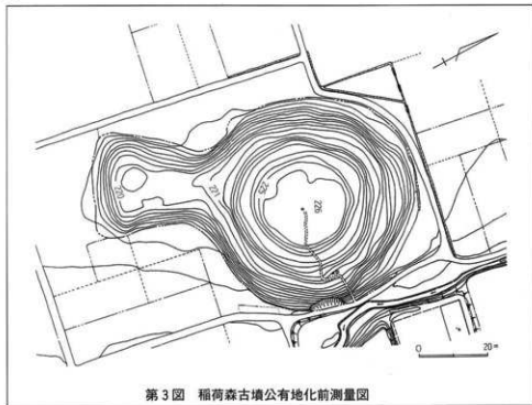
第3図 稲荷森古墳公有地化前測量図
