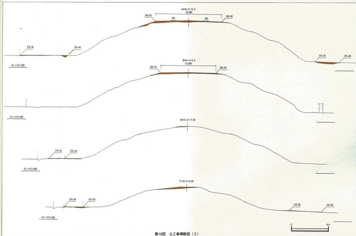
第10図 土工事横断面図(2)
