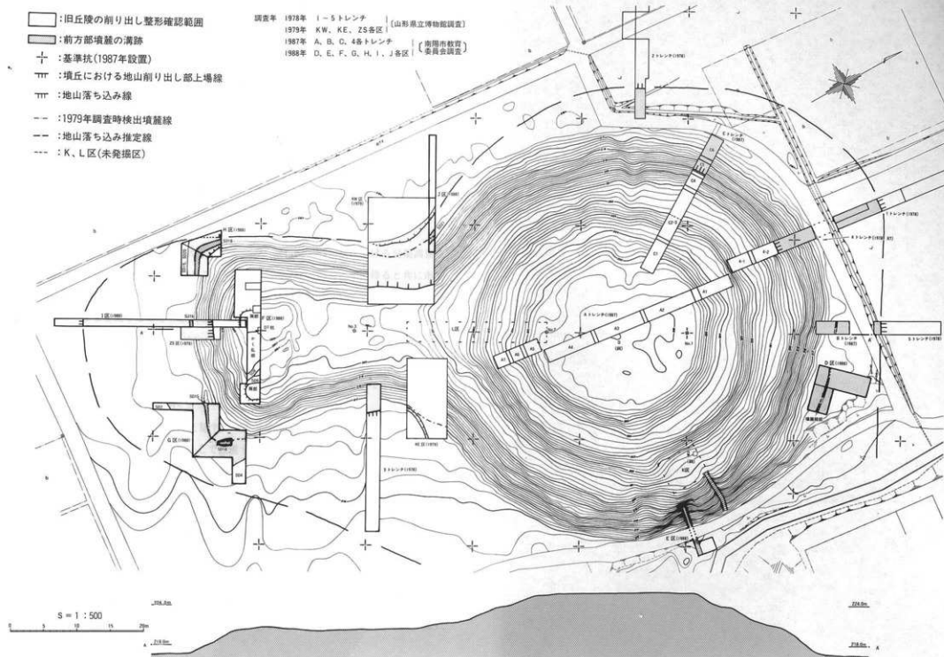
第6図 稲荷森古墳調査全体図
