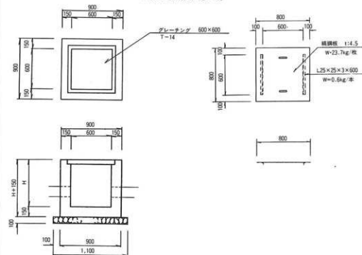
第14図 給水工・排水工詳細図
