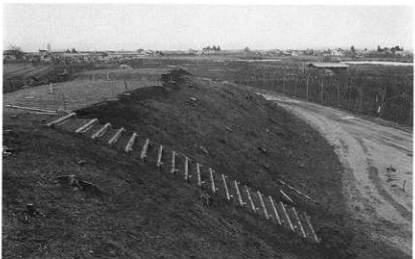
図版8 填丘階段工事 (平成2年度)
