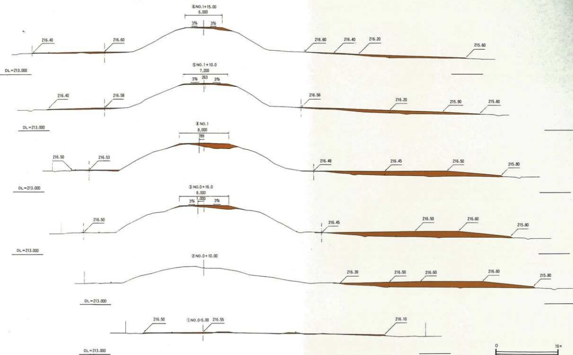
第9圖 土工事横断面圖(1)
