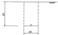
(2)暗渠構造図(1:20)
