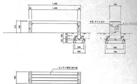
第26図 ベンチ構造図
