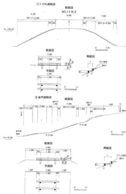
第16図 階段工詳細図
