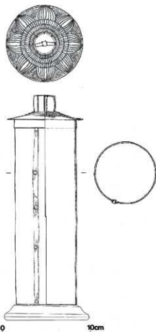
図3 経筒実測図
