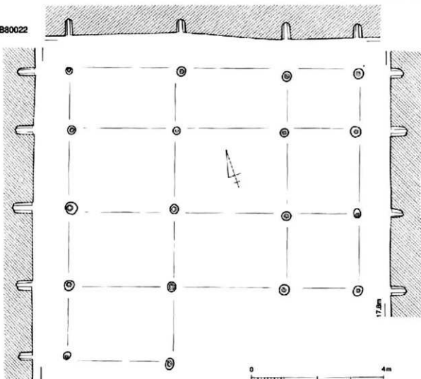
掘立柱建物11 (SB80021・80022)
