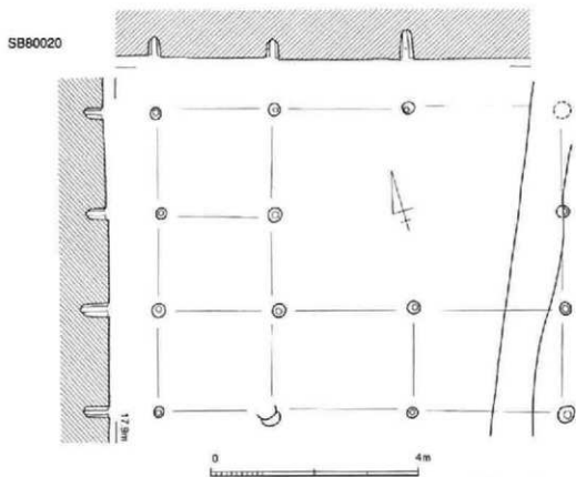
掘立柱建物10 (SB80019・80020)
