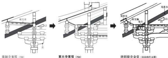
図18 奈良時代の三手先組物の変遷
