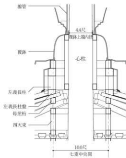
図12 奈良時代創建の東大寺東塔 相輪下部断面図 1:300
