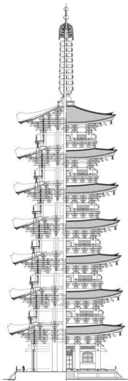
図17 鎌倉時代再建の東大寺東塔（東西面） 立断面図 1:500
