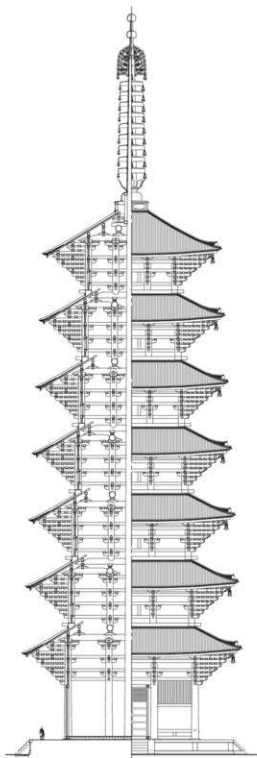
図16 鎌倉時代再建の東大寺東塔（東西面） 立断面図 1:500
