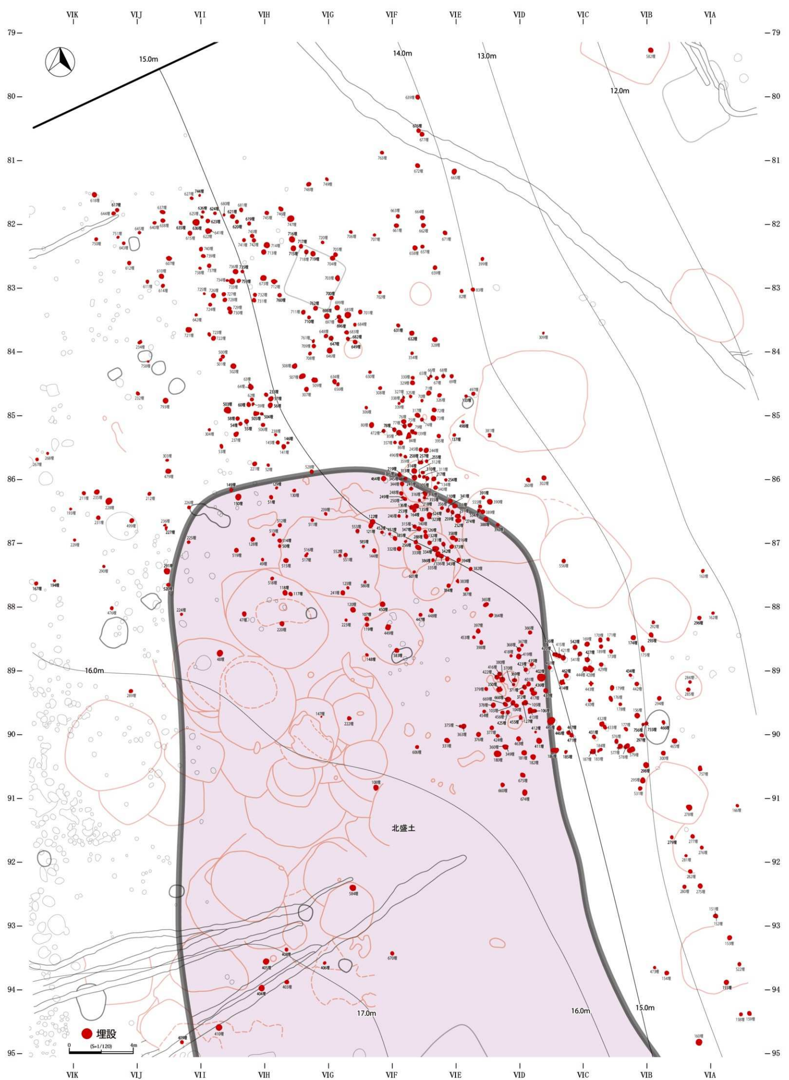
付図 3-1 旧野球場建設予定地埋設土器遺構配置図
