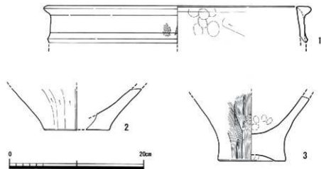
第4図 5号土坑出土土器実測図 (S=1/4)
