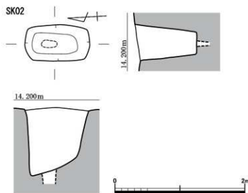
第22図 2号土坑 平面図・断面図 (S=1/40)
