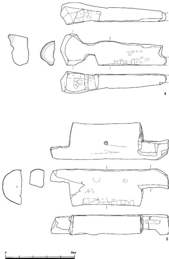
第18图 1号井戸出土木杵④、⑤実測図(S=1/8)
