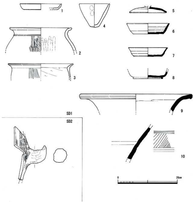
第9图 1号・2号沟出土土器实测图 (S=1/4)
