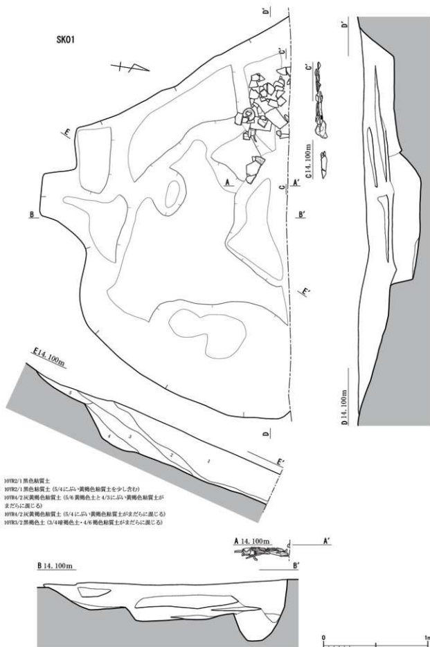
第 12 図 1 号土坑 平面図・断面図 (S=1/25)
