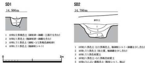
第8図 1号・2号溝 土層断面図 (S=1/40)
