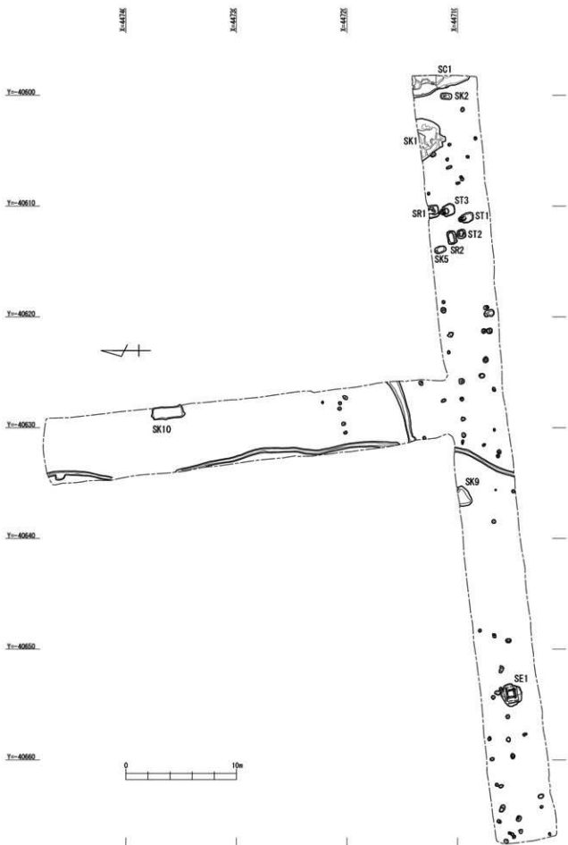
第2図 大板井遺跡 32 遺構配置図 (S=1/300)
