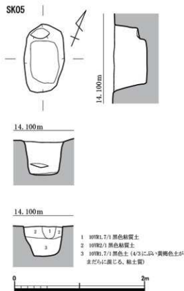
第3図 5号土坑 平面図・断面図 (S=1/40)
