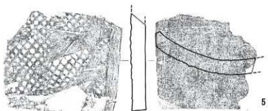
第15图 1号土坑出土瓦实测图②(S=1/4)
