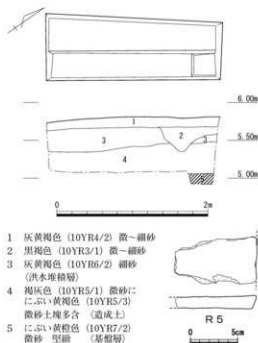
第14図 T 7 (1/50)・出土遺物 (1/4)
