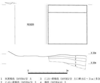
第18図 T11 (1/50)
