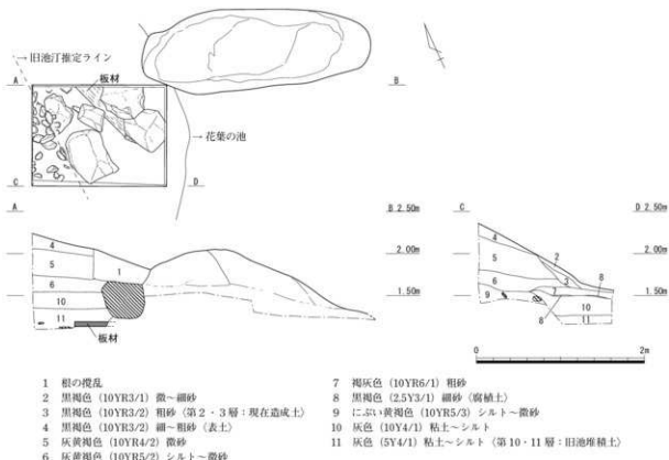
第10図 T5 (1/50)
