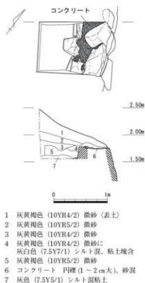
第6図 T1 (1/50)
