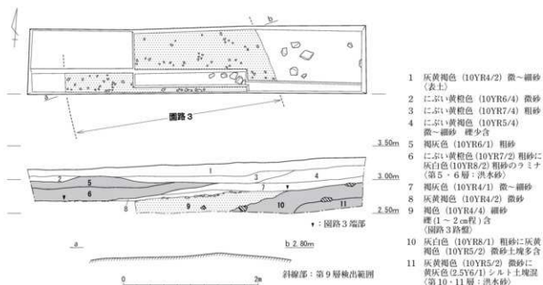
第21図 T13 (1/50)
