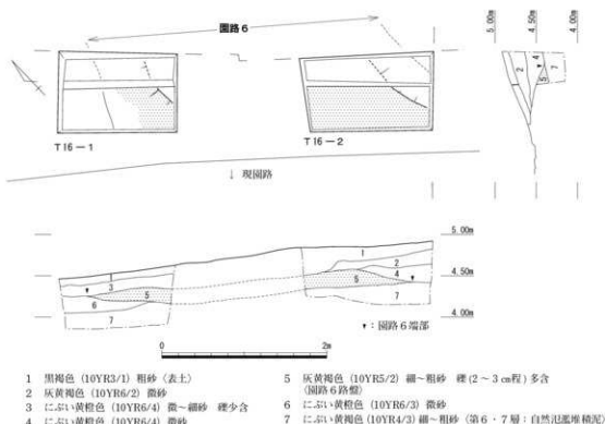
第25図 T16-1・T16-2 (1/50)
