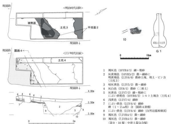
第22図 T14 (1/50)・出土遺物(1/4)
