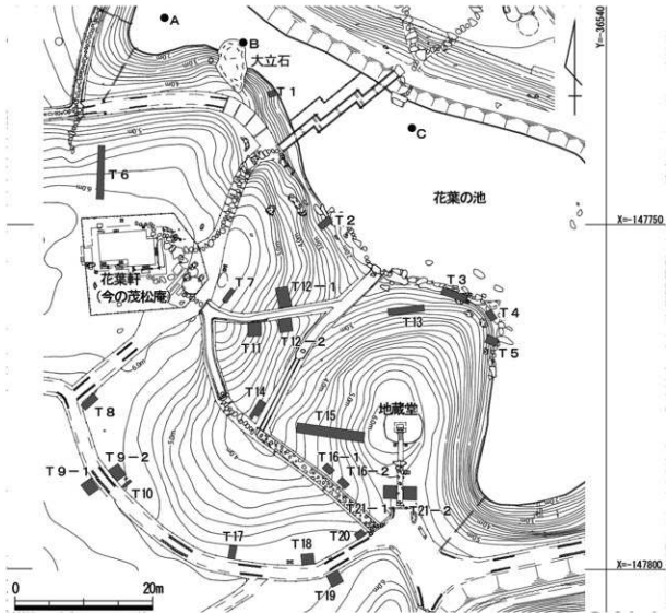
第5図 トレンチ配置図 (1/600)
