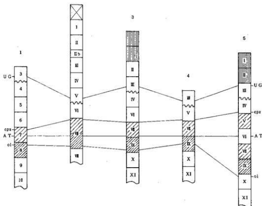
(1. B区V-35グリッド、2. 海浜市中三谷、3. 藤川市提灯木山、4. 伊奈町大山、 5. 武蔵野台地。柱状図は模式。UG:UG層準、AT:AT層準、cpx:単斜輝石層準、ol:カンラン石層準。)
