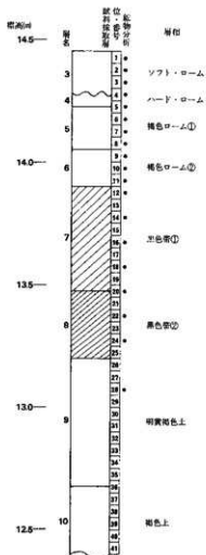
第72図 B区V-35 深掘の横式柱状図 および植物分析試料採取位置
