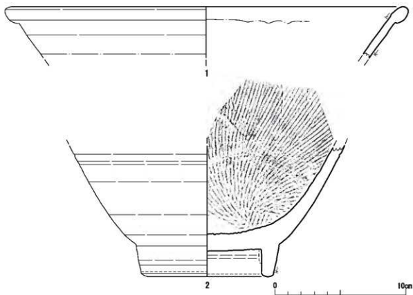
第31図(図版28) 本土産陶器：摺鉢
