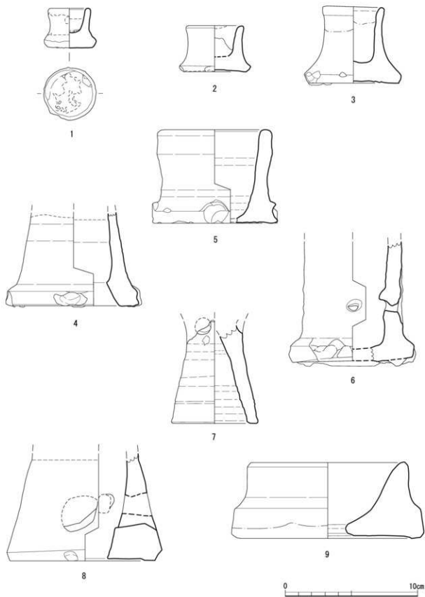
第24図(図版21) 窯道具：筒状のトチン
