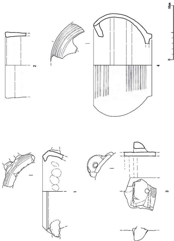
第20图(图版17) 陶質土器：炉
