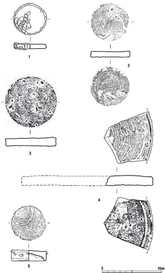
第22図(図版19) 窯道具：円形ハマ
