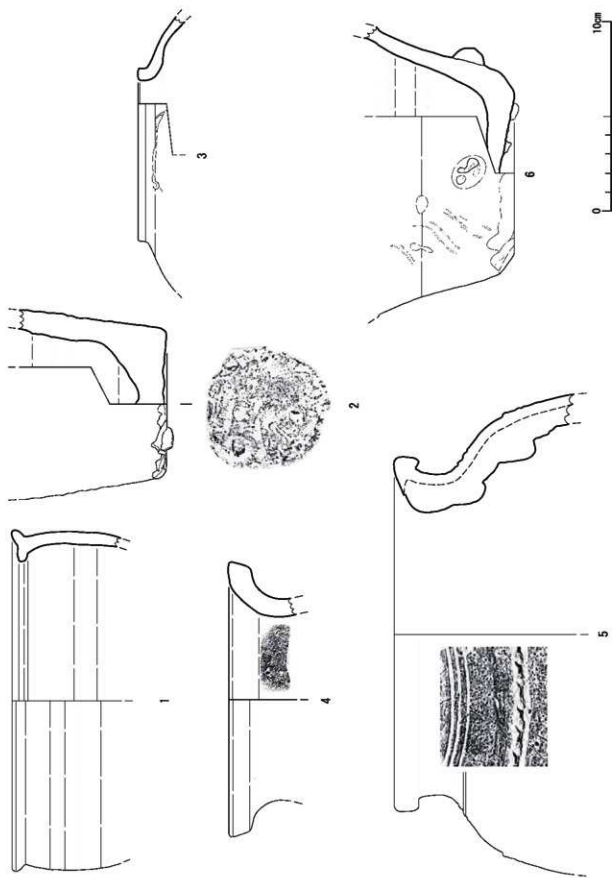
第18图(图版15) 無軸陶器：鉢 (1)、德利 (2)、壺 (3~6)
