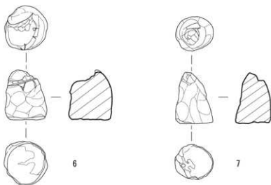
第 26 図(図版 23) 窯道具：円柱状製品
