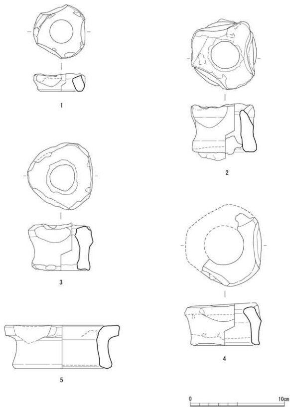
第23図(図版20) 窯道具：抉り入りハマ
