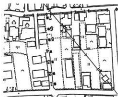
第9図 トレンチ配置図(1/2,500)
