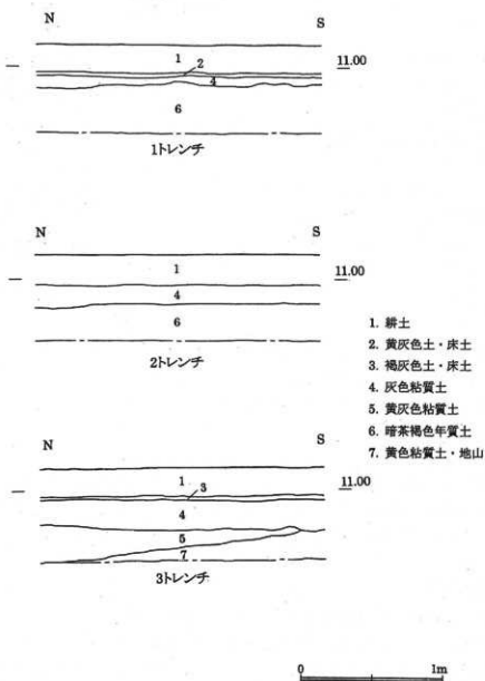
第8図 土層断面図
