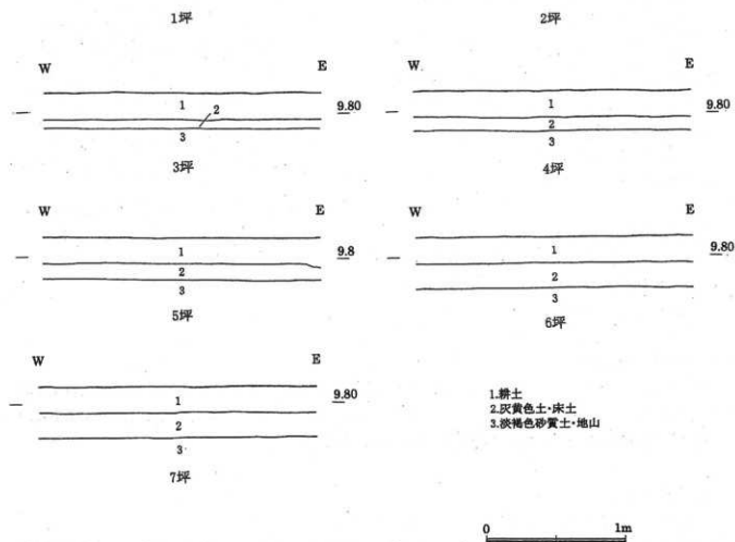
第 21 图 土層断面图
