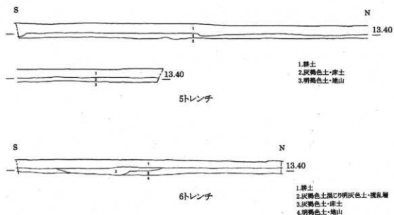
第14図 土層断面図(2)
