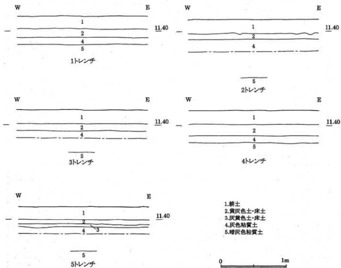
第 23 図 土層断面図
