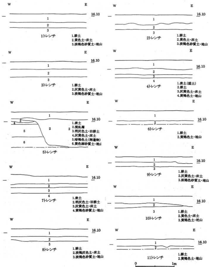
第 17 図 土層断面図(1)
