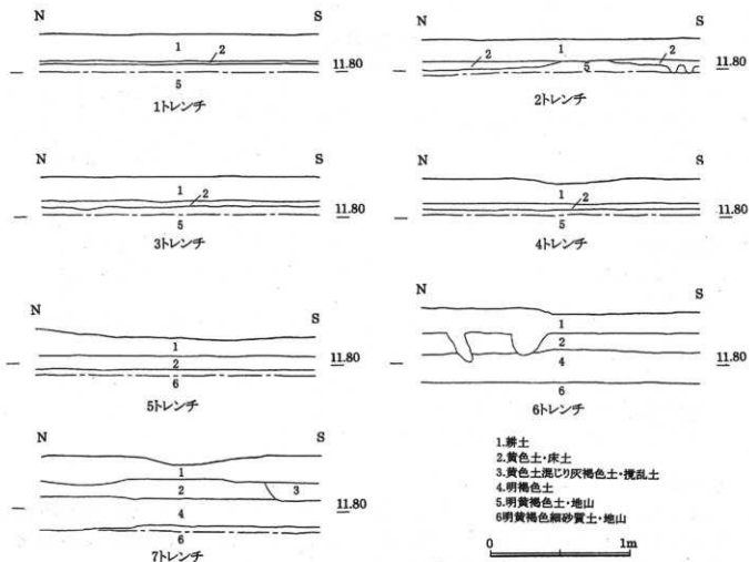
第10図 土層断面図
