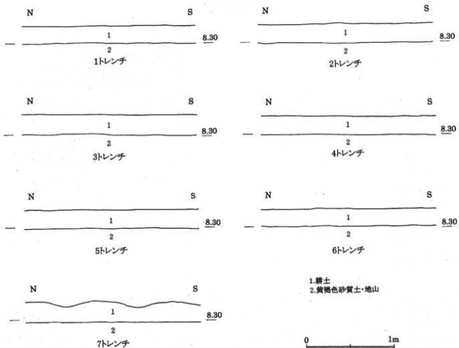
第4図 土層断面図
