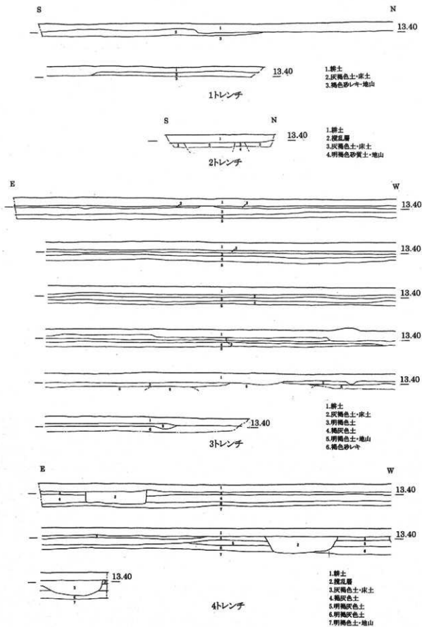
第13図 土層断面図(1)
