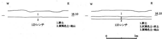
第18図 土層断面図(2)
