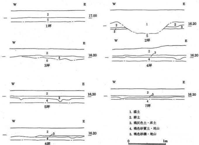
第6図 土層断面図
