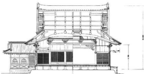
圖8 聖德殿前殿桁行断面圖 (文化財建造物保存技術協會作成)
