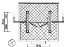
図44 表門平面図
