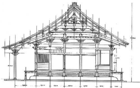
图6 講堂梁行断面图 (中道建築設計事務所作成)
