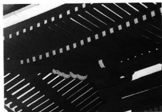
写真52 鐘樓組物・兩持送
