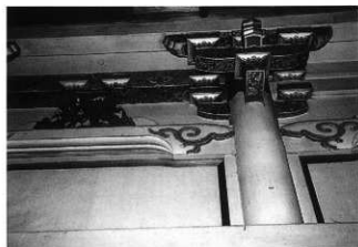
写真36 聖徳殿後殿入側柱外側組物
