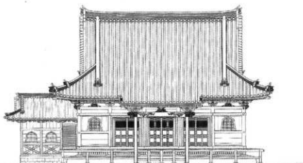
圖7 聖德殿前殿正立面圖 (文化財建造物保存技術協會作成)
