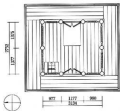
図16 鐘樓平面図 (左: 上層, 右: 下層)
