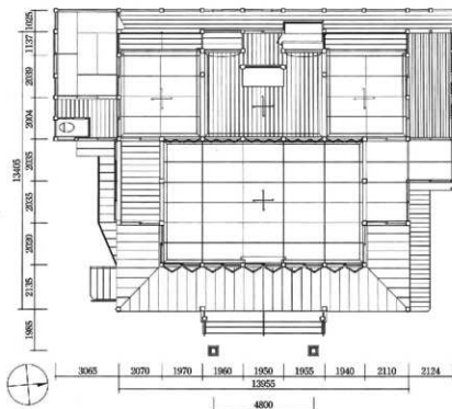
図55 本堂平面図
