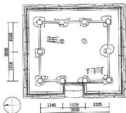
図16 鐘樓平面図 (左: 上層, 右: 下層)
