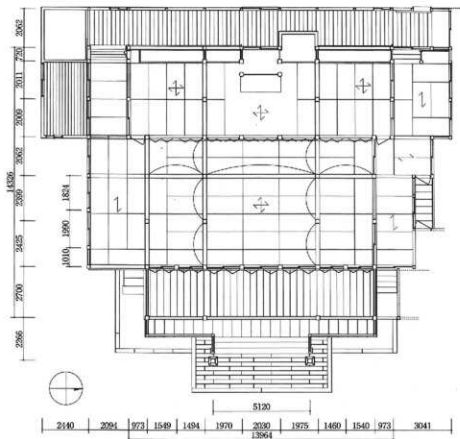
図67 本堂平面図
