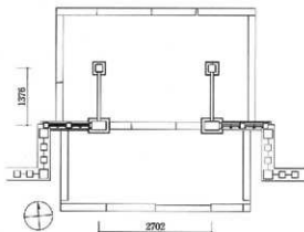
図34 表門平面図
