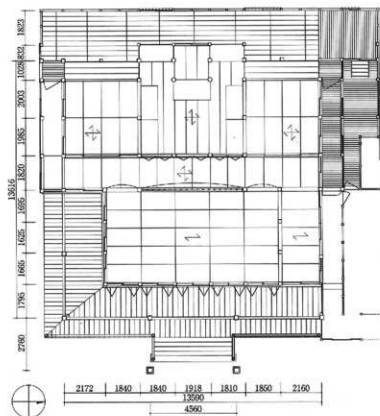
図39 本堂平面図
