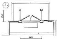
図57 表門平面図
