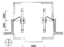
図22 表門平面図
