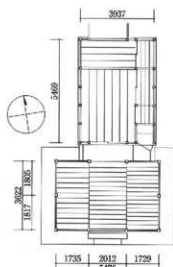
図36 拝殿・幣殿平面図
