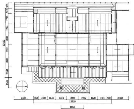
図29 本堂平面図
