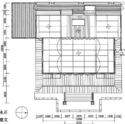
図74 本堂平面図
