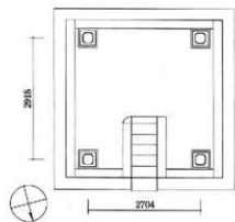
図26 鐘樓平面図
