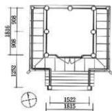
図71 本殿平面図
