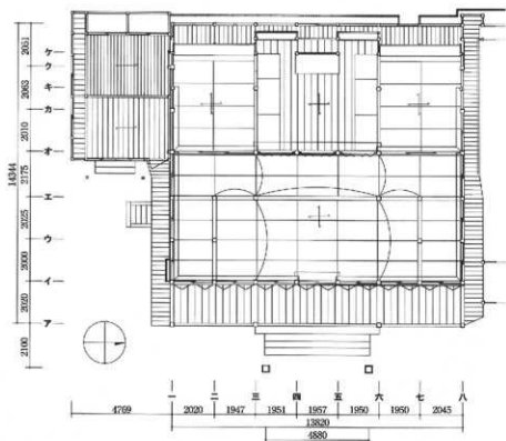
图58 本堂平面图
