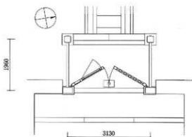
図38 表門平面図
