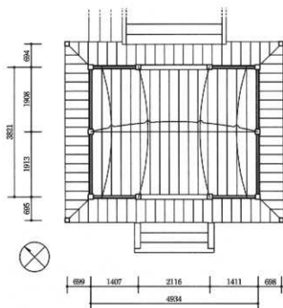
図65 拝殿平面図
