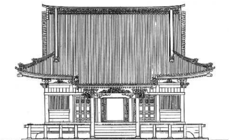
圖5 講堂正立面圖 (中道建築設計事務所作成)
