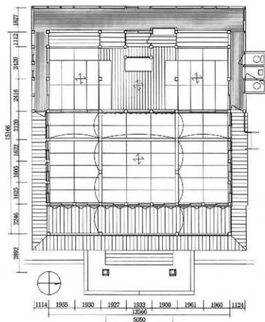
図61 本堂平面図
