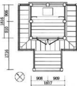
図64 本殿平面図
