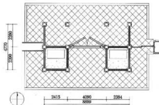
図11 仁王門平面図
