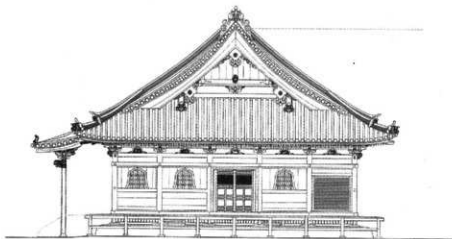
图10 聖德殿前殿側立面图 (文化財建造物保存技術協会作成)
