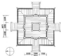
图14 三重塔平面图
