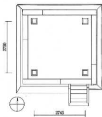
図59 鐘樓平面図
