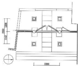
図54 表門平面図
