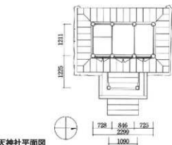
图17 天神社平面图
