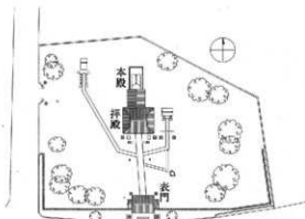
図33 崇導神社配置図
