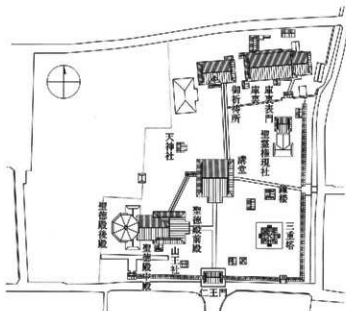
図4 斑鳩寺配置図
