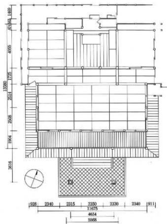
図76 本堂平面図
