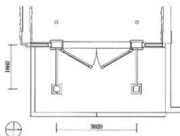
図48 表門平面図
