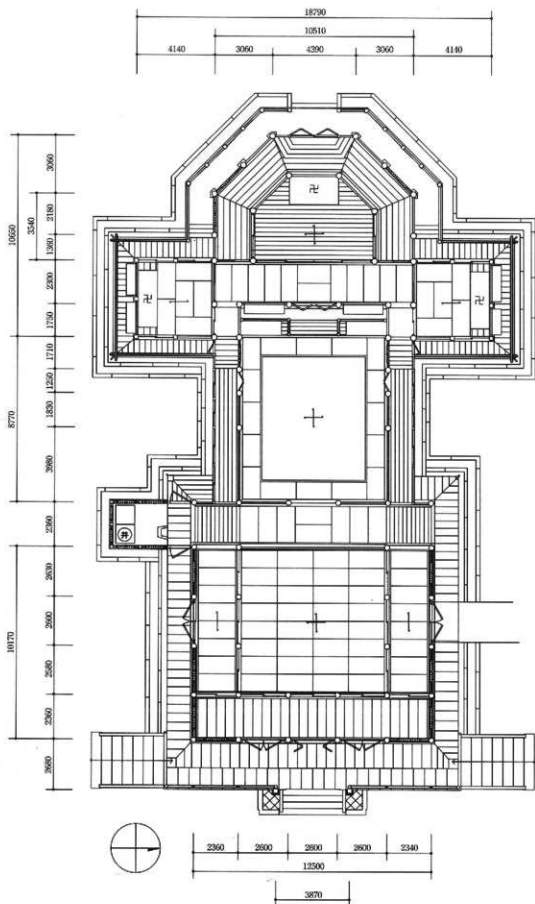
图13 聖德殿前殿·中殿·後殿平面图
