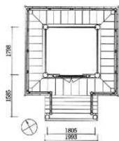
図45 本殿平面図
