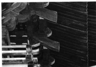
写真48 三重塔三層組物
