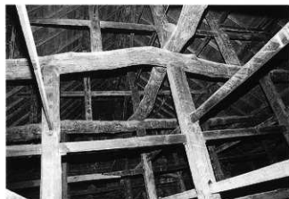
写真124 本堂小屋組
