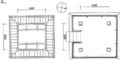
図75 鐘樓平面図 (左:上層、右:下層)
