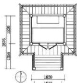
図51 本殿平面図
