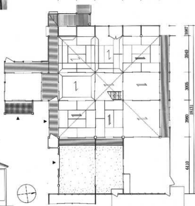
図69 庫裏平面図(上:二階、下:一階、一点鎖線×印部に二階が載る)
