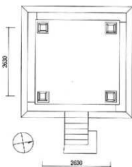
図32 鐘楼平面図
