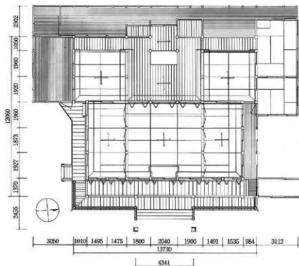
図31 本堂平面図
