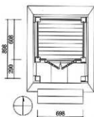
図42 本殿平面図
