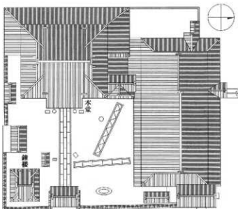
図30 了源寺配置図
