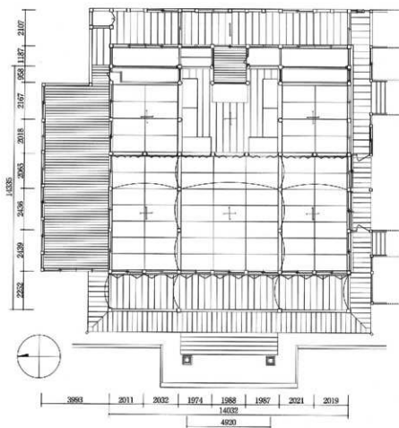
図25 本堂平面図
