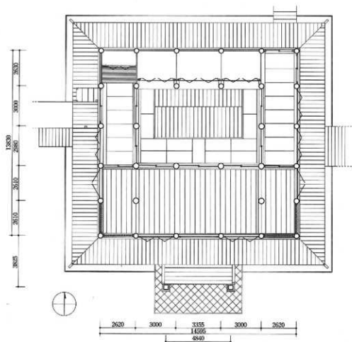
図12 講堂平面図
