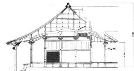
图9 聖德殿前殿梁行断面图 (文化財建造物保存技術協会作成)
