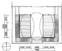
図46 拝殿平面図
