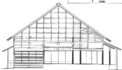
图20 庫裏断面図
