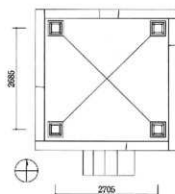
図70 鐘楼平面図
