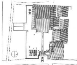
図37 蓮光寺配置図
