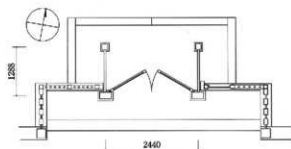
図50 表門平面図
