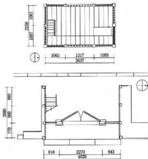
図28 鐘樓門平面図(上:上層、下:下層)
