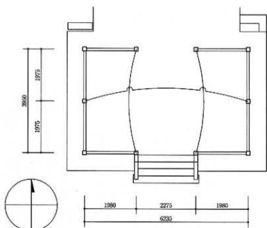
图52 拝殿平面図
