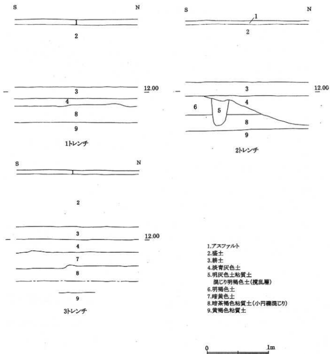
第8図 土層断面図
