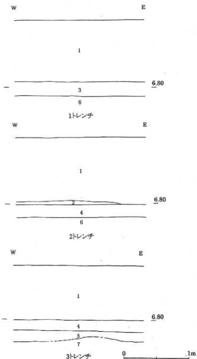
第4図 土層断面図
